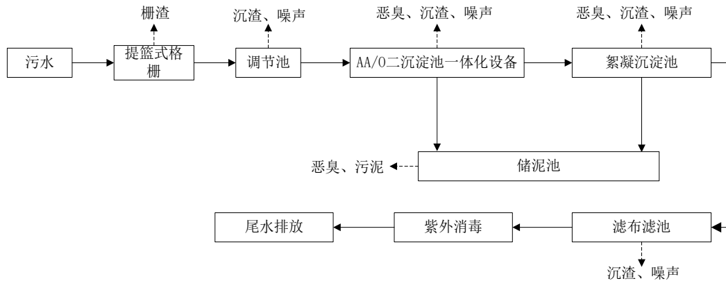
图 2.1-6 污水处理工艺流程图
