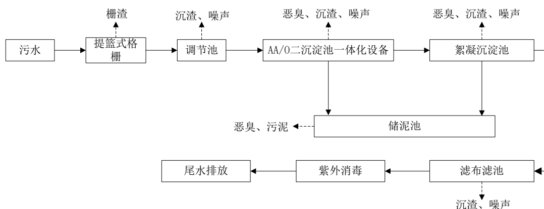
图 2.1-5 A 2 /O 工艺流程图
