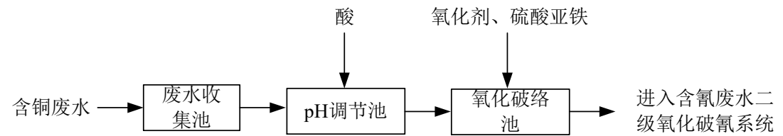
图 4.3-29 含铜废水处理工艺流程图
