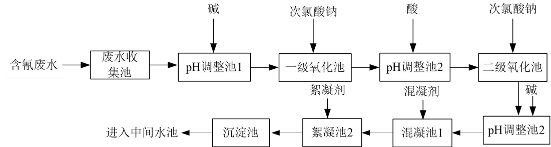
图 9.2.2-1 含氰废水处理工艺流程图
