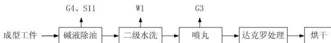
图 3.1-11 达克罗工艺产污节点图
