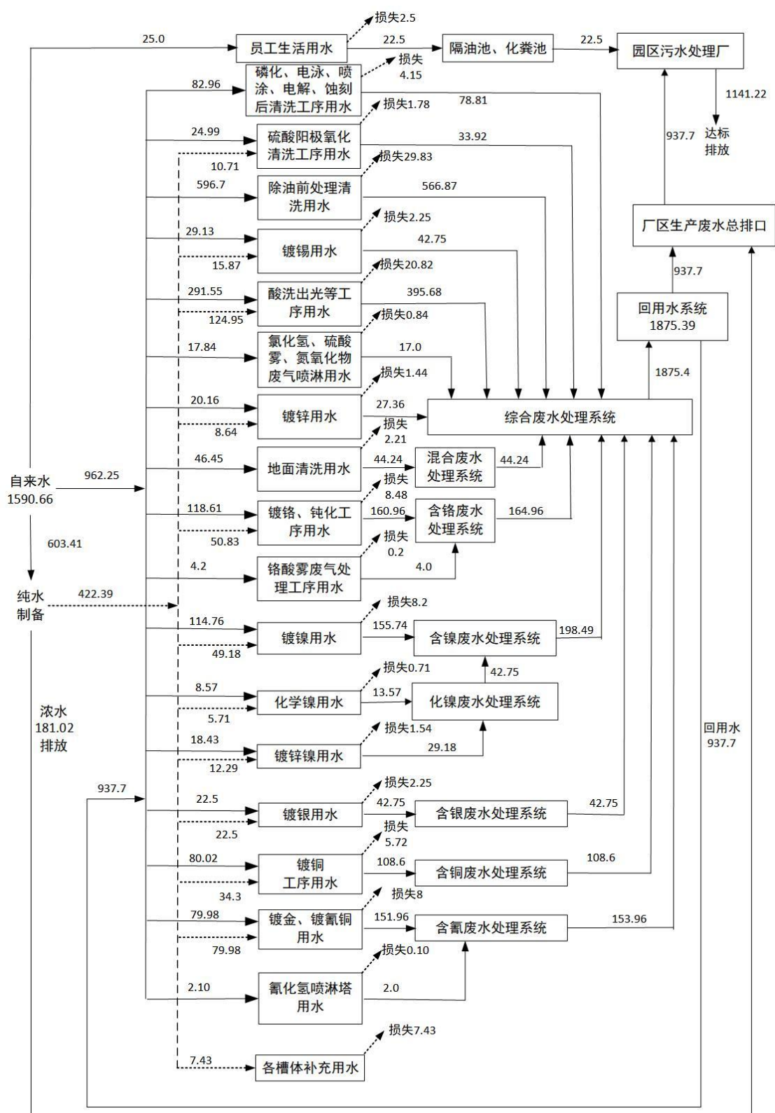
图 4.2-1 项目水平衡图 单位: \text{m}^3/\text{d}
