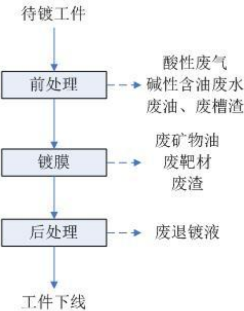
图 4.1-20 真空镀工艺流程及产污环节图
