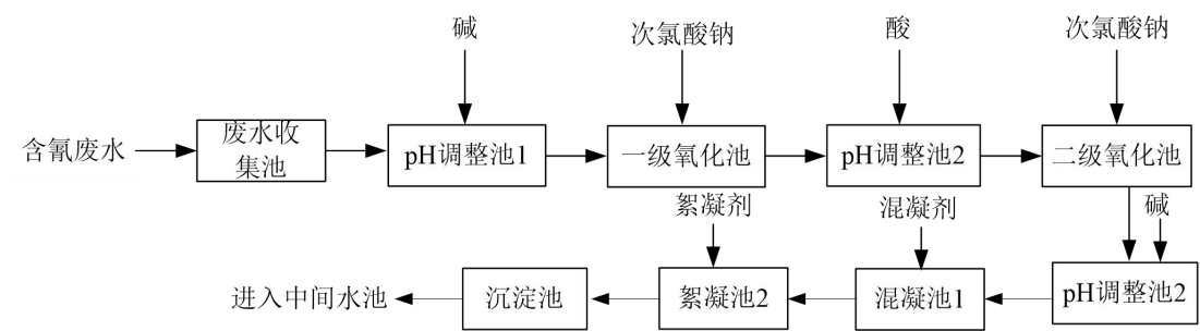
图 4.3-28 含氰废水处理工艺流程图
