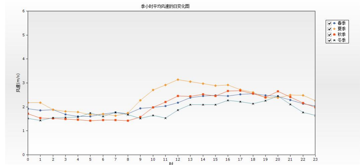
图 7.2-6 2024 年各季日平均风速变化曲线图
