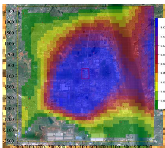
图 7.2-10 叠加后 PM 10 最大日均 (95%保证率) 浓度影响 (μg/m 3 )
