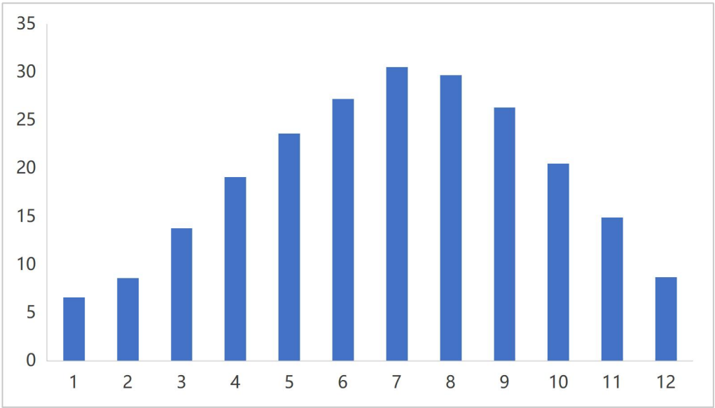
图 7.2-3 衡阳月平均气温（单位：℃）
