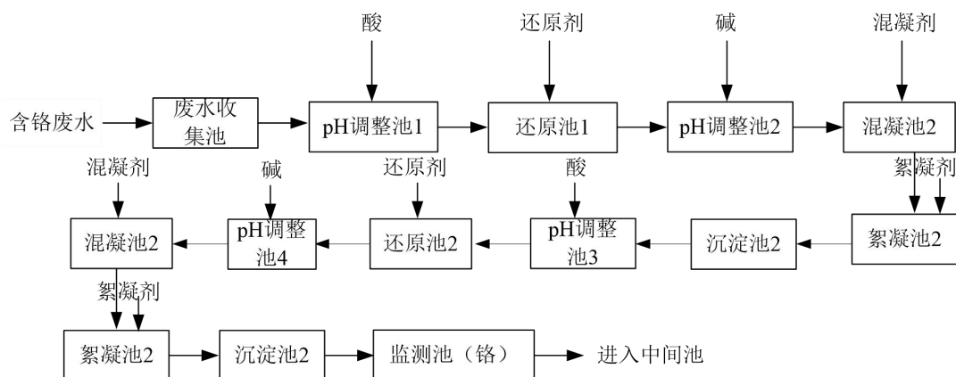
图 9.2.2-4 含铬废水预处理流程
