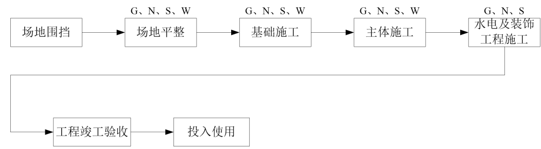
注：G 废气、N 噪声、S 固废、W 废水 图 4.3-1 项目施工工艺流程及产污节点图
