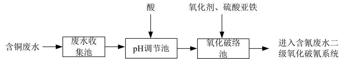
图 9.2.2-6 含铜废水预处理流程
