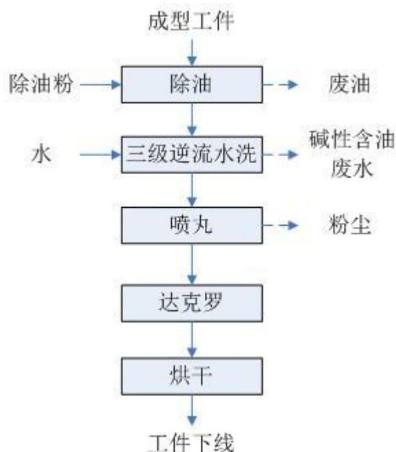
图 4.1-21 达克罗工艺流程及产污节点图
