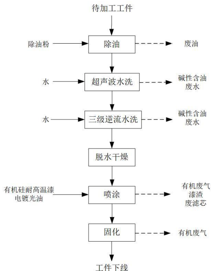
图 4.1-19 喷涂线工艺流程及产污环节图
