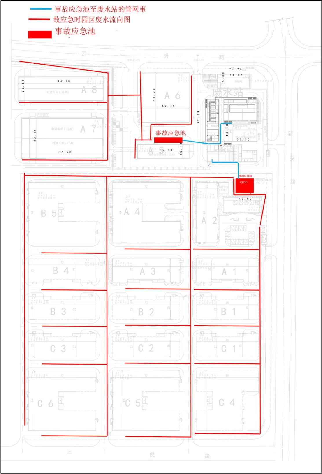
图 8.7-2 事故废水排放路径图
