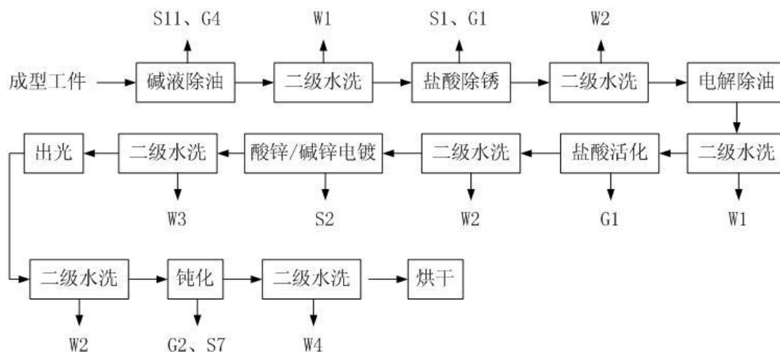
图 3.1-2 酸锌、碱锌电镀产污节点图
