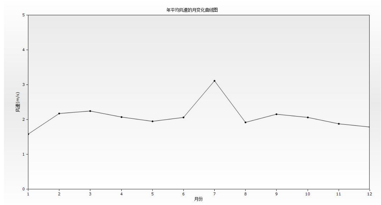
图 7.2-5 2024 年各月平均风速变化曲线图
