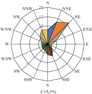
图 7.2-2 衡阳风向玫瑰图（静风频率 5.3%）
