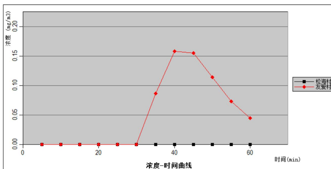
图 8.6-2 最不利气象条件主要关心点 HCl 浓度随时间变化情况图
