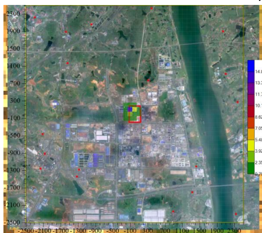
图 7.2-13 叠加后 TSP 最大年均浓度影响 ( \mu\text{g}/\text{m}^3 )
