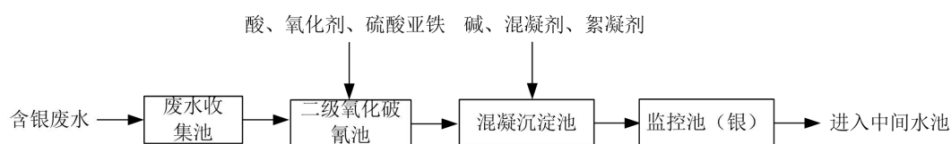
图 9.2.2-5 含银废水预处理流程
