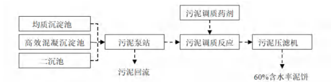
图 5.3-2 常德高新技术开发区污水处理厂污泥处理工艺流程图
