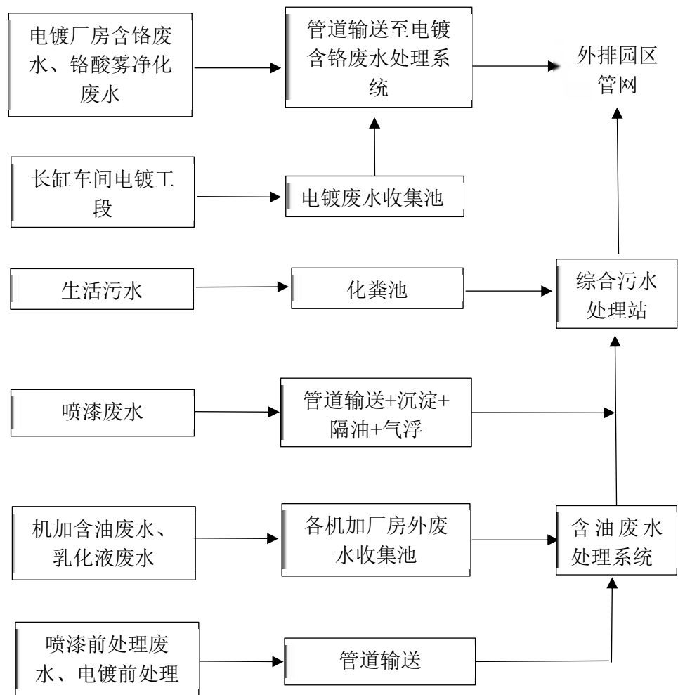
图 3.1-11 现有工程全厂废水走向图
