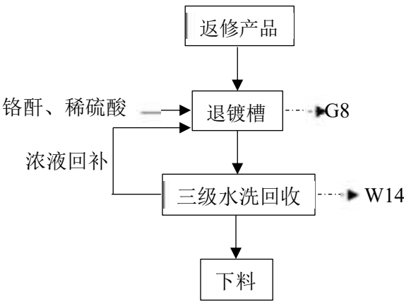
图 4.2-4 退镀线工艺流程及产污环节图
