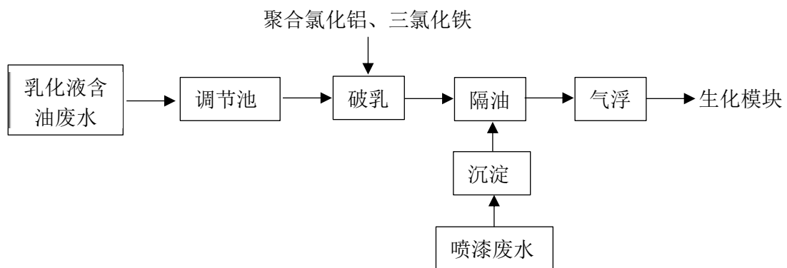
图 3.1-13 含油废水、喷漆废水处理工艺流程图
