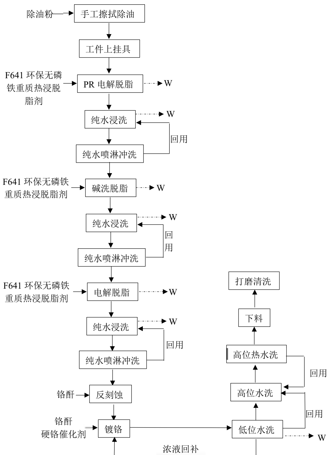
图 3.1-3 2.8m 活塞杆镀铬生产线工艺流程及产污环节图
