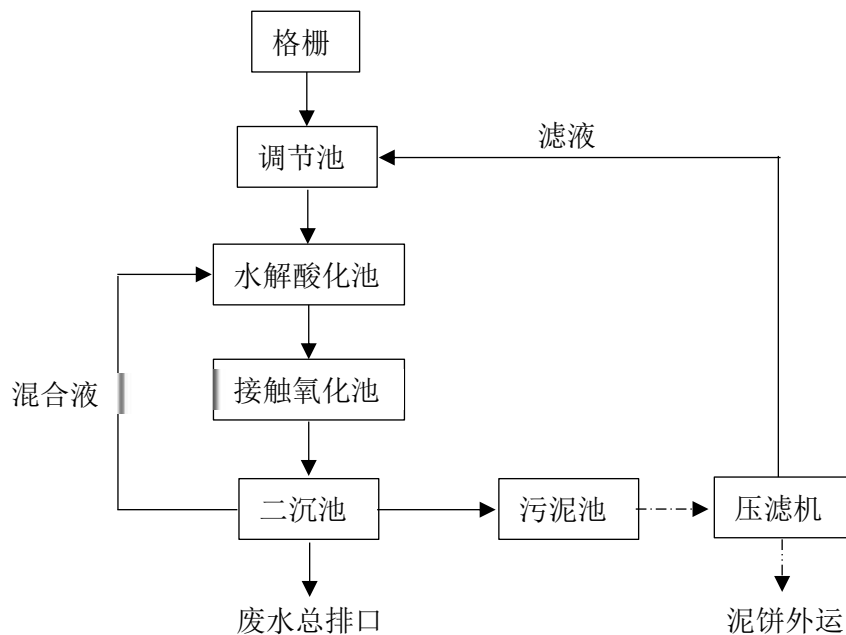
图 3.1-14 综合污水处理工艺流程图
