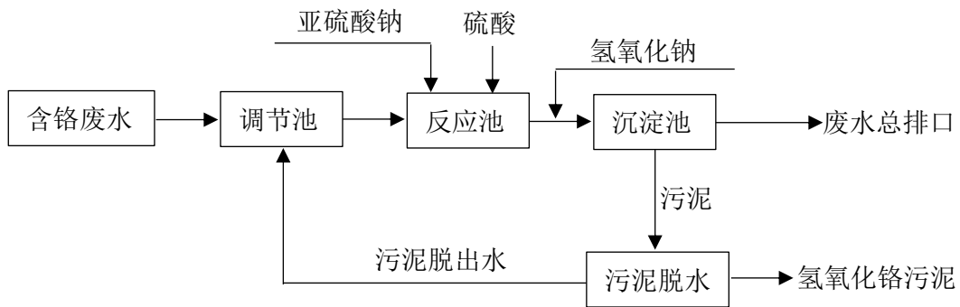
图 7.2-3 含铬废水处理模块处理工艺流程图
