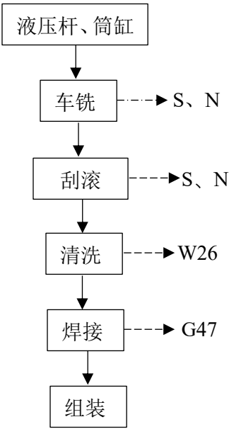
图 4.2-12 机加区工艺流程及产污环节图
