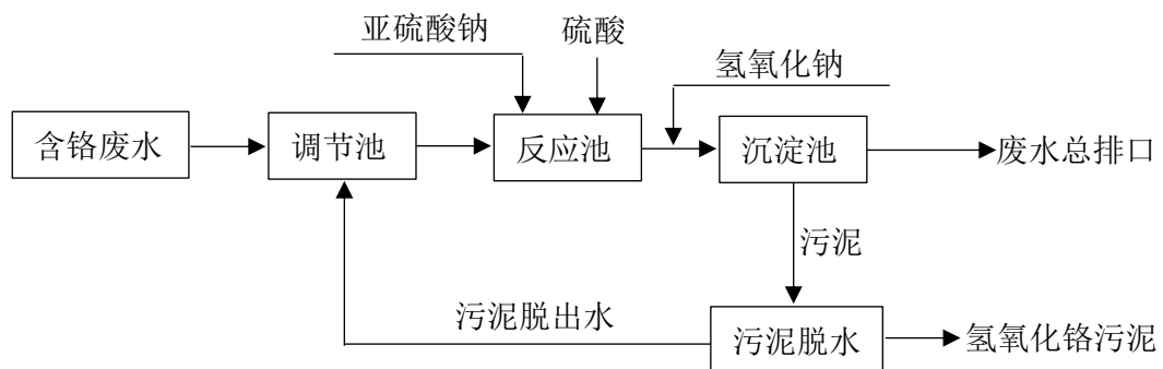
图 3.1-12 电镀含铬废水处理工艺流程图
