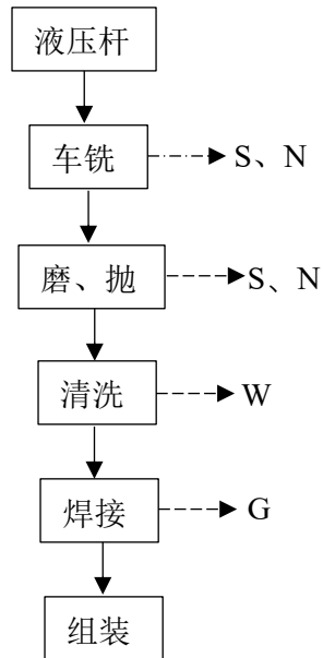
图 3.1-9 机加区工艺流程及产污环节图
