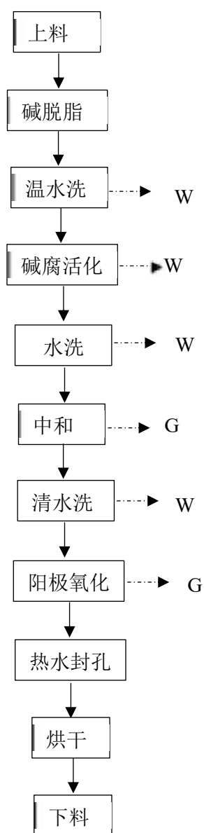
图 3.1-6 阳极氧化生产线工艺流程及产污环节图
