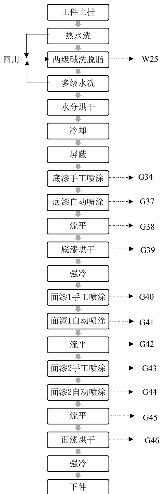
图 4.2-11 涂装区生产线工艺流程及产污环节图
