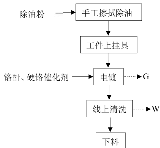
图 3.1-8 滚镀、连镀生产线工艺流程及产污环节图
