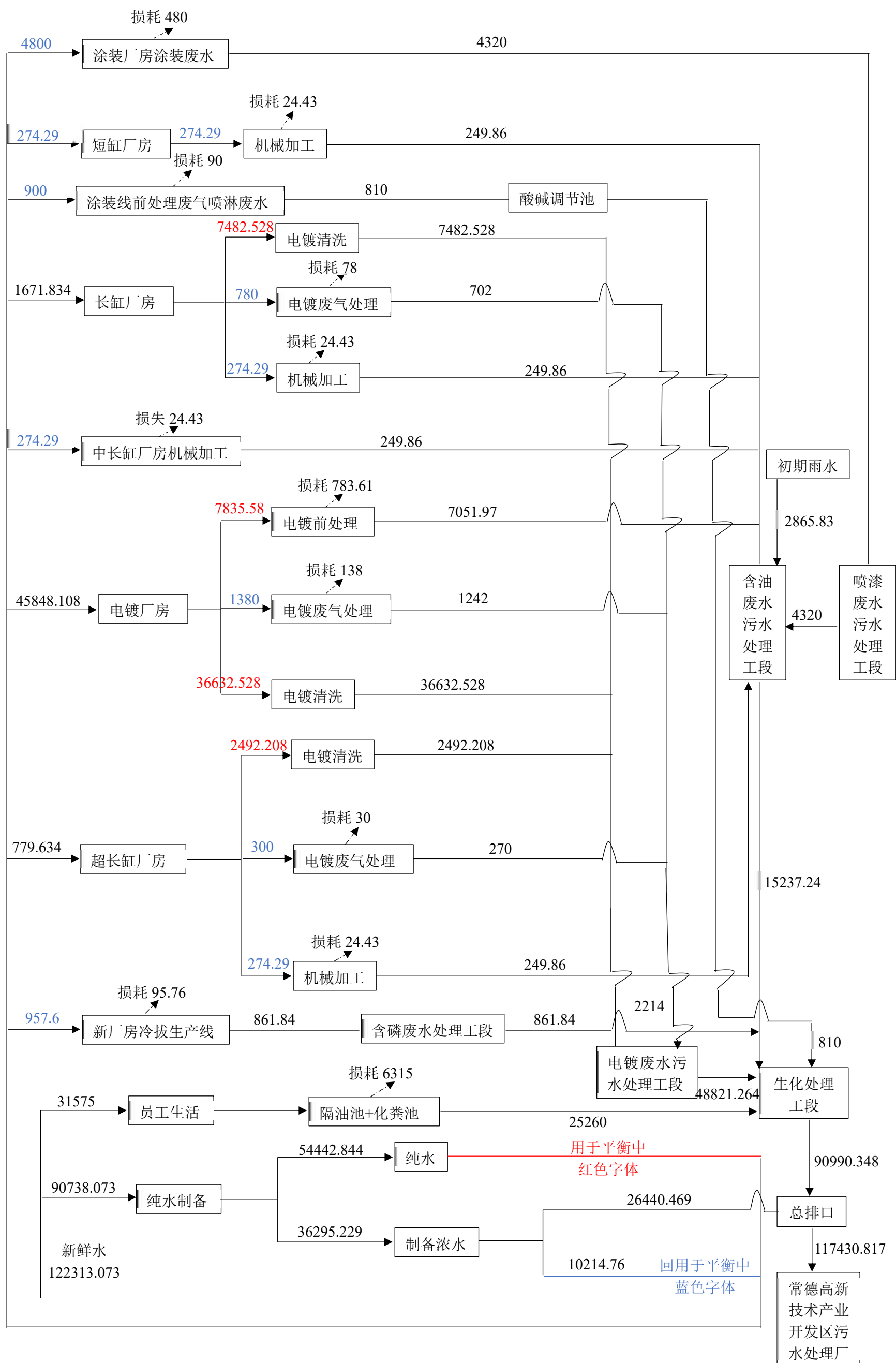
图 4.2-1 厂区水平衡图 单位: \text{m}^3/\text{a}
