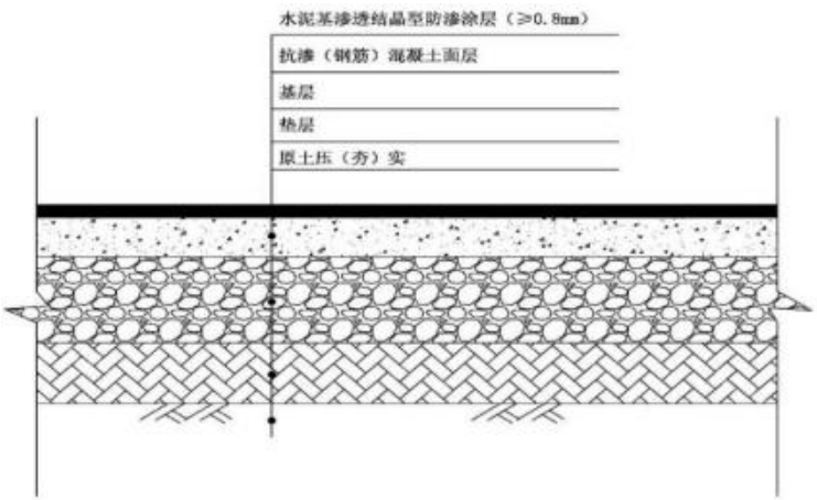
图 7.2-11 重点防渗区地面刚性防渗示意图
