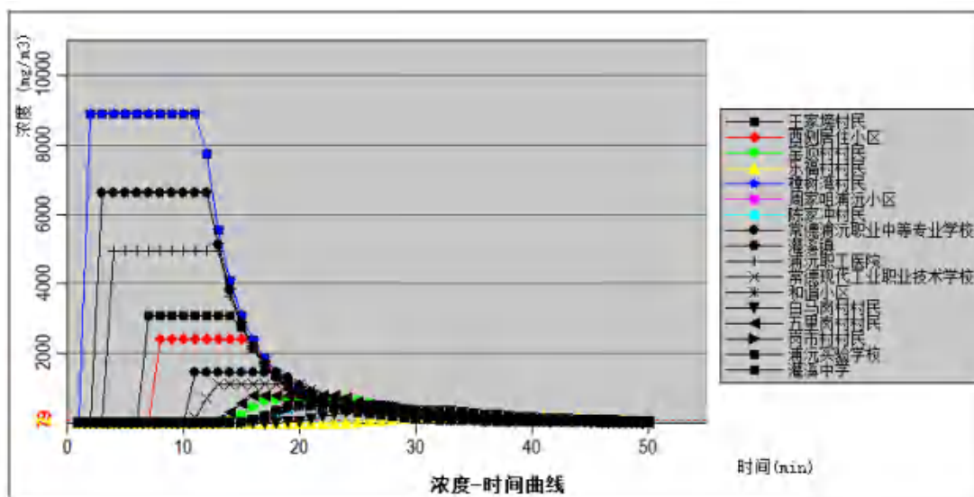
图 8.6-2 主要关心点二氧化硫浓度随时间变化情况图
