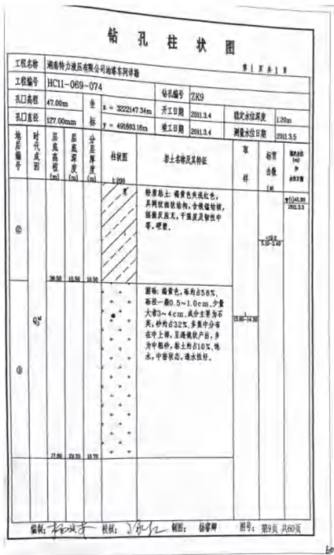
图 6.2-1 厂区水文地质图
