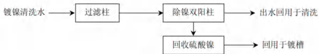
图 7.2-7 离子交换技术工艺流程图
