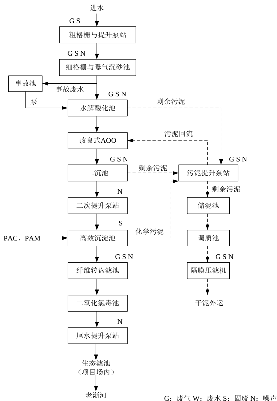
图 6.2-1 常德高新技术产业开发区污水处理厂污水处理工艺流程图
