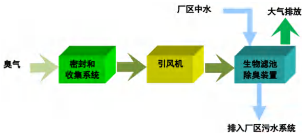
图 5.3-3 常德高新技术开发区污水处理厂除臭处理工艺流程图
