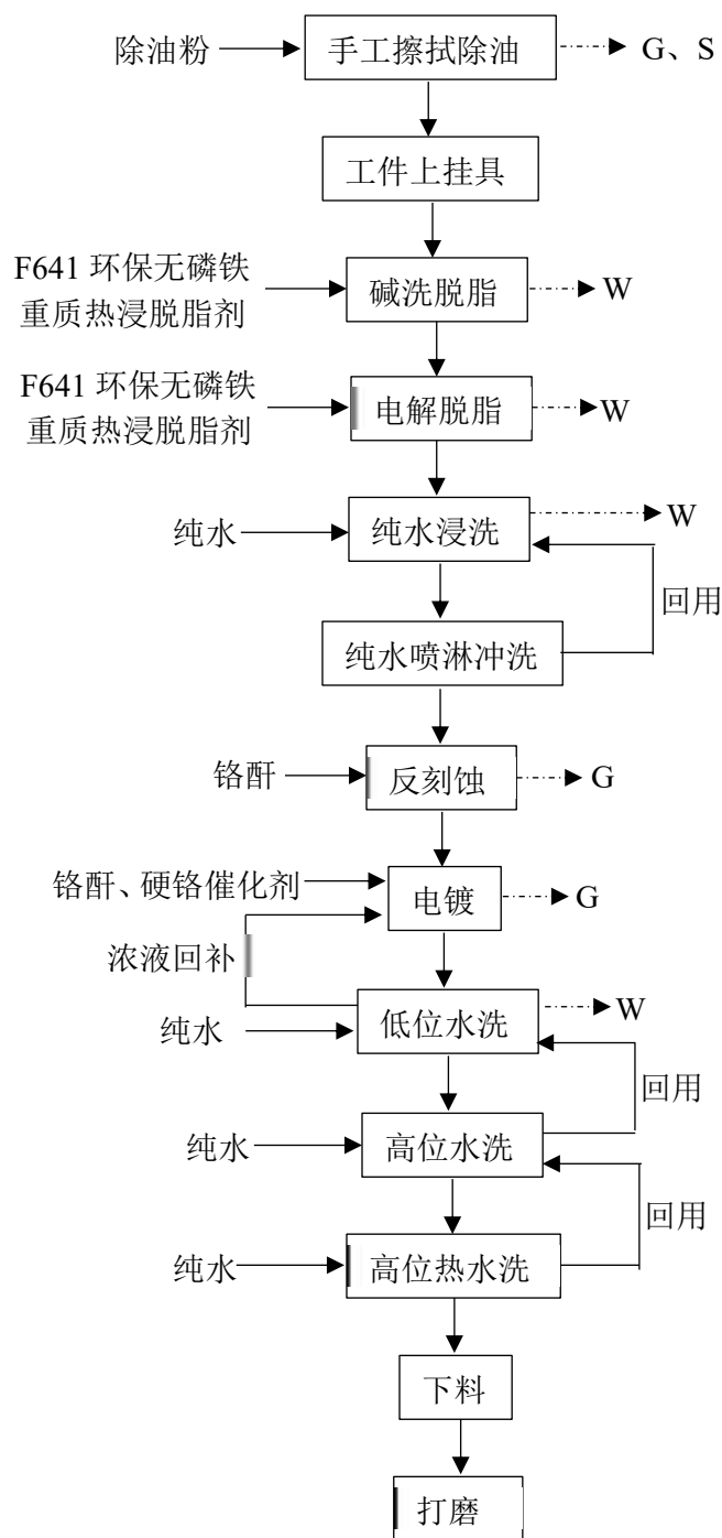
图 3.1-2 3m、5m 活塞杆镀铬生产线工艺流程及产污环节图
