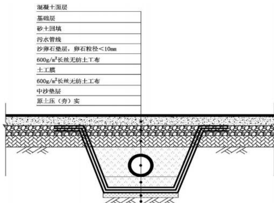
图 7.2-13 地下污水管线防渗示意图
