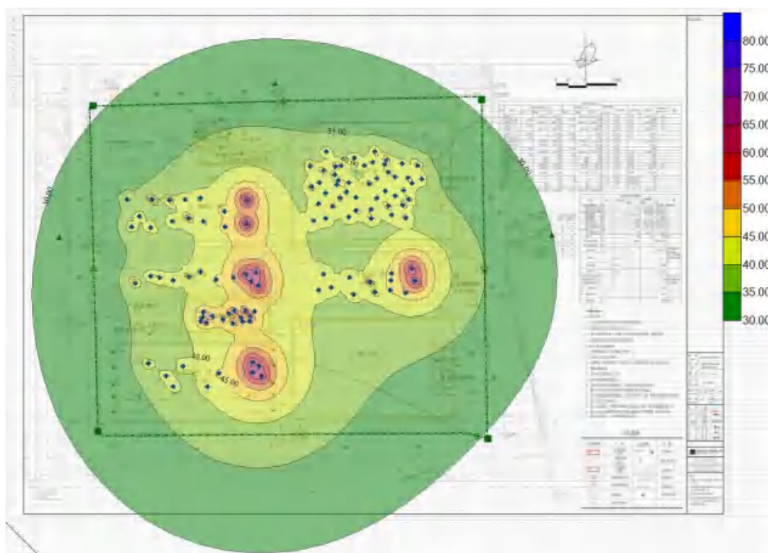
图 6.2-1 项目贡献值等值线图
