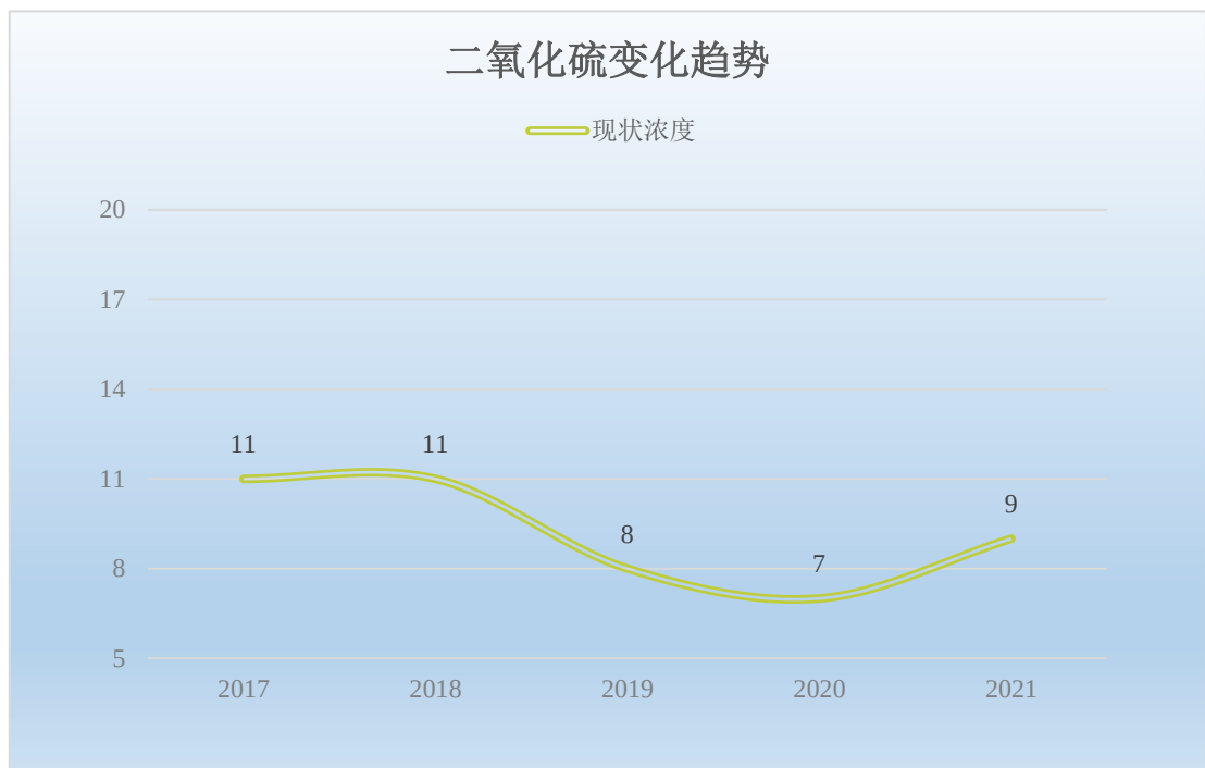
图 5.4-1 SO 2 年平均浓度变化趋势图
