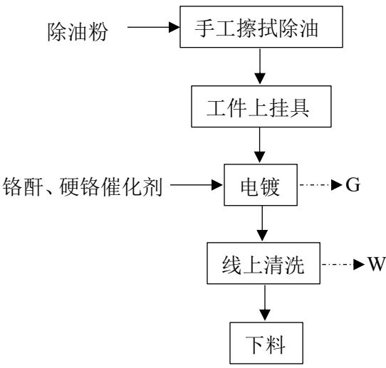
图 3.1-5 深井镀生产线工艺流程及产污环节图
