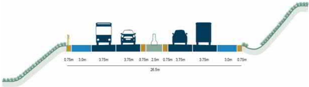
图 2.6-1 整体式路基标准横断面图（宽度 26.5m）
