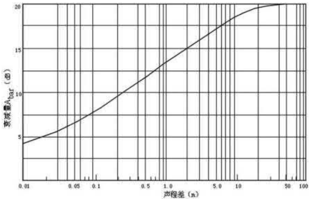
图 6.4-4 噪声衰减量 A_{\bar{a}} 与声程差 \delta 关系曲线 ( f=500\text{Hz} )
