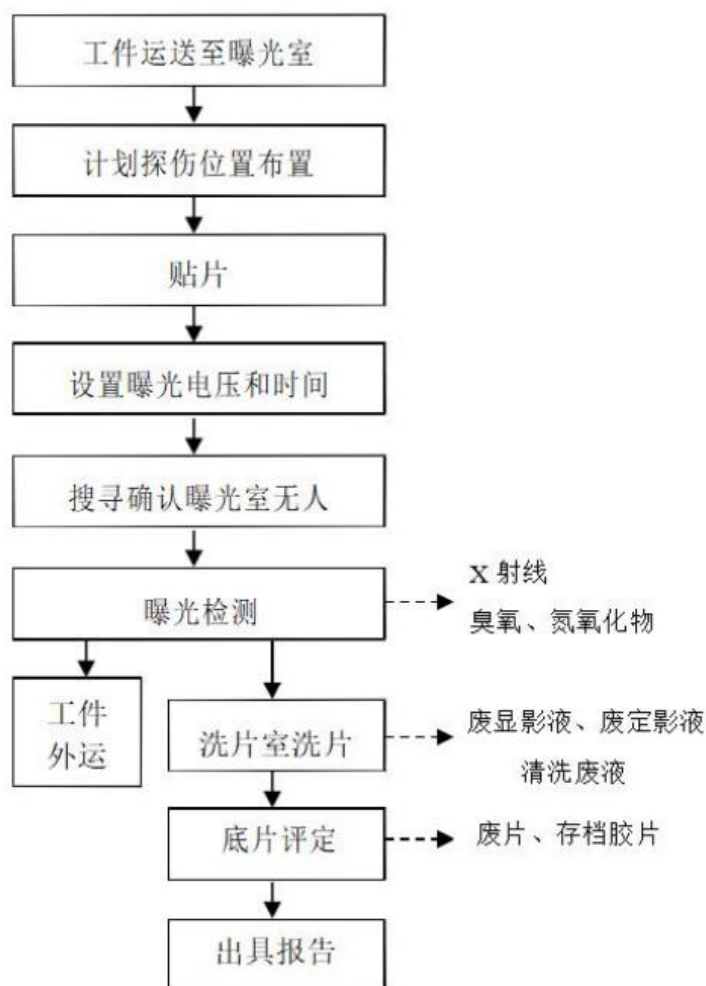
图 9-3 探伤工艺流程简图
