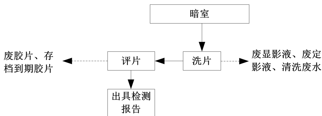
图 9-4 X 射线探伤机工艺流程及产污环节图
