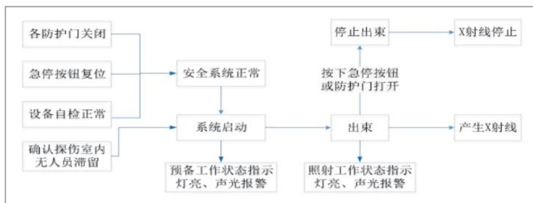
图 10-3 辐射安全防护联锁逻辑图
