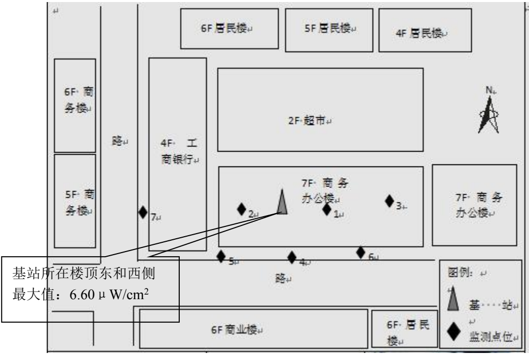
图 6-3-1 洞口县供销大厦基站监测布点示意图
