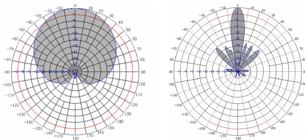
图 3-6 电磁波波束水平方向剖面图 图 3-7 电磁波波束垂直方向剖面图
