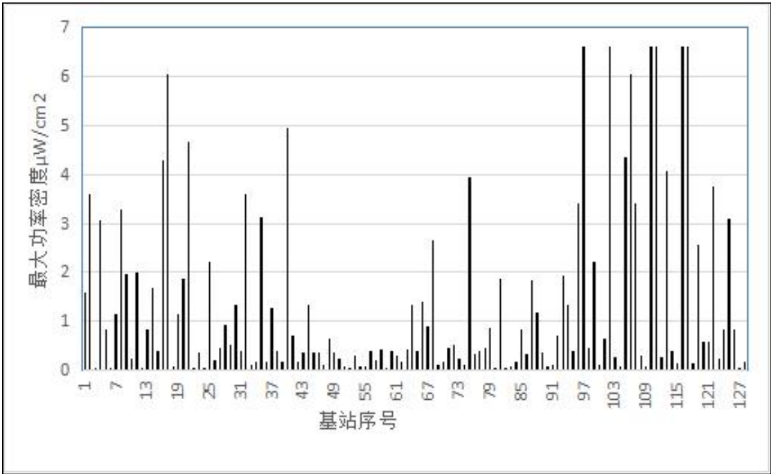
图 6-1 抽测基站等效平面波功率密度最大值统计柱状图
