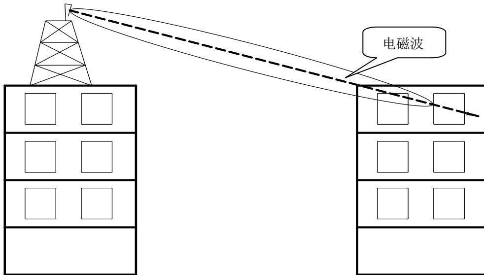
图 3-10 移动通信基站电磁辐射传播示意图
