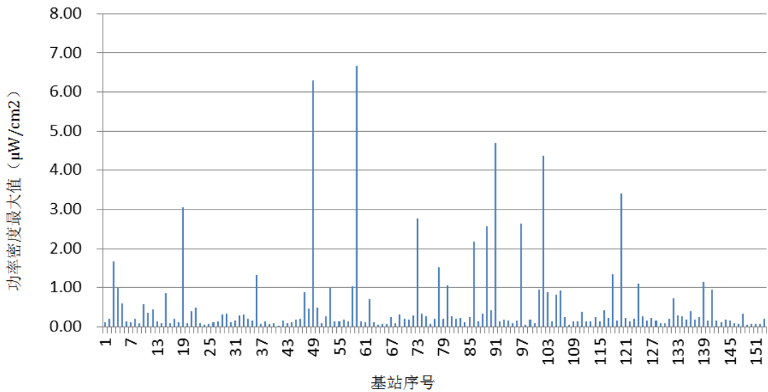
图 6-1 抽测基站等效平面波功率密度最大值统计柱状图
