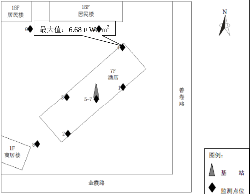
图 6-3-1 常德市区-鼎城征稽所基站监测布点示意图
