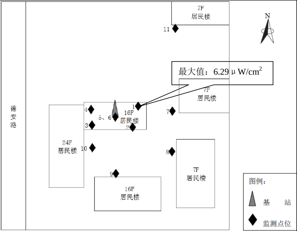
图 6-2-1 常德市区-鼎城浙风名邸基站监测布点示意图
