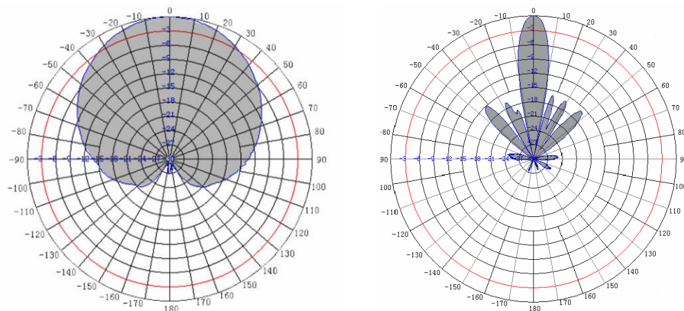
图 3-6 电磁波波束水平方向剖面图 图 3-7 电磁波波束垂直方向剖面图
