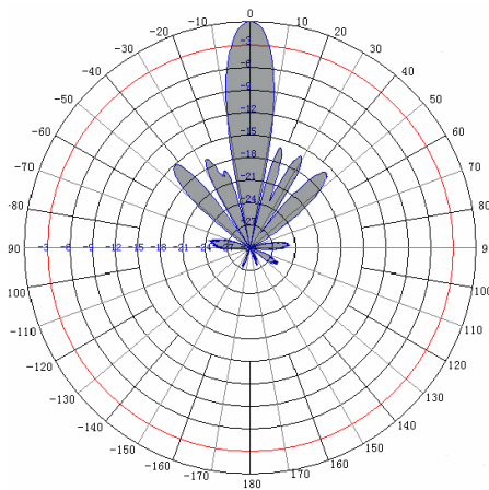
图 3-6 电磁波波束水平方向剖面图 图 3-7 电磁波波束垂直方向剖面图
