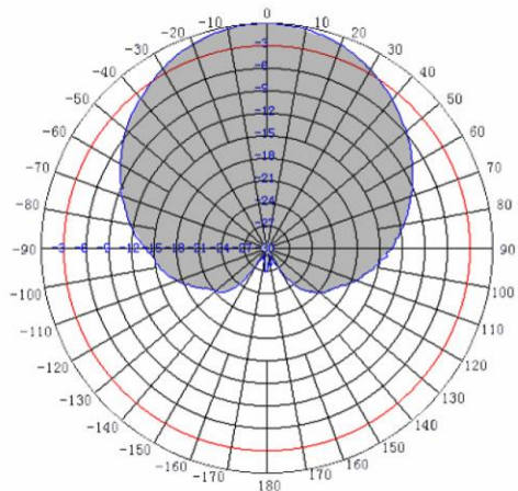
图 3-6 电磁波波束水平方向剖面图 图 3-7 电磁波波束垂直方向剖面图
