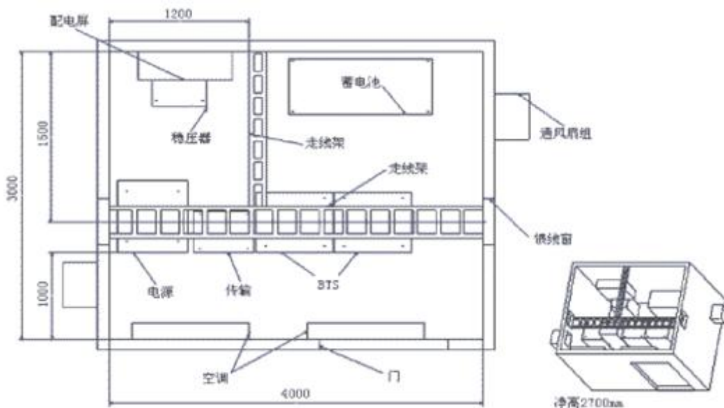
图 3-1 基站机房设备组成
