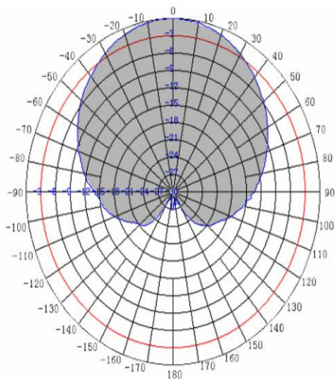
图 3-6 电磁波波束水平方向剖面图 图 3-7 电磁波波束垂直方向剖面图
