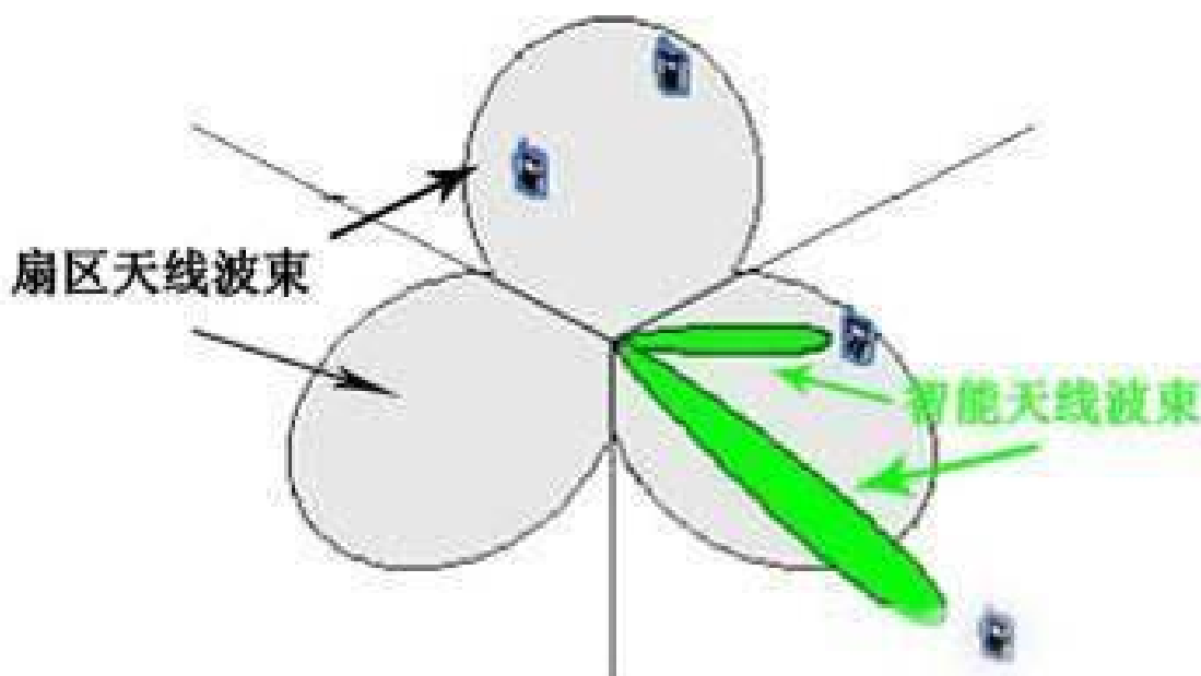
图 3-9 智能天线与扇区天线之间的差别
