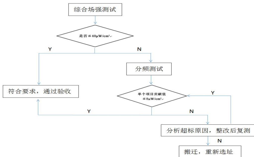
图 4-1 基站验收监测工作流程图
