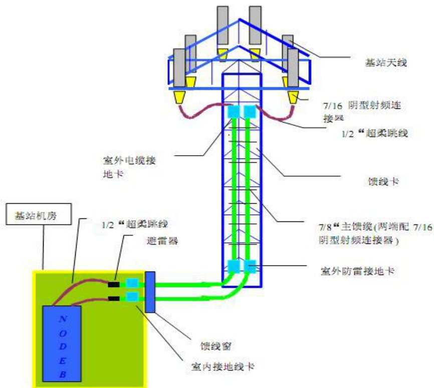
图 3-2-2 基站机房设备组成
