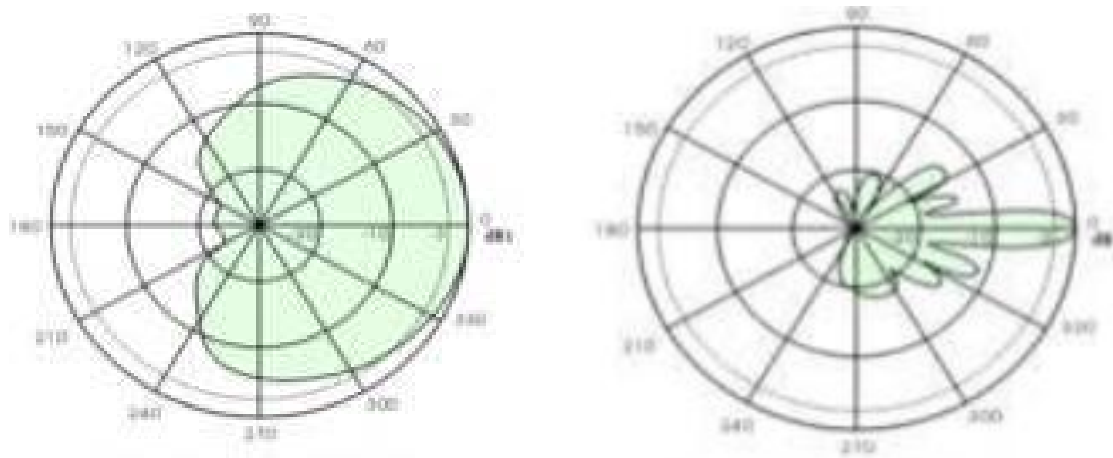
定向智能天线单天线水平方向
