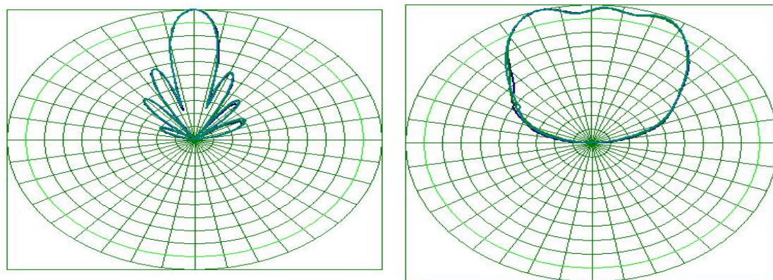
定向智能天线0°业务波束
