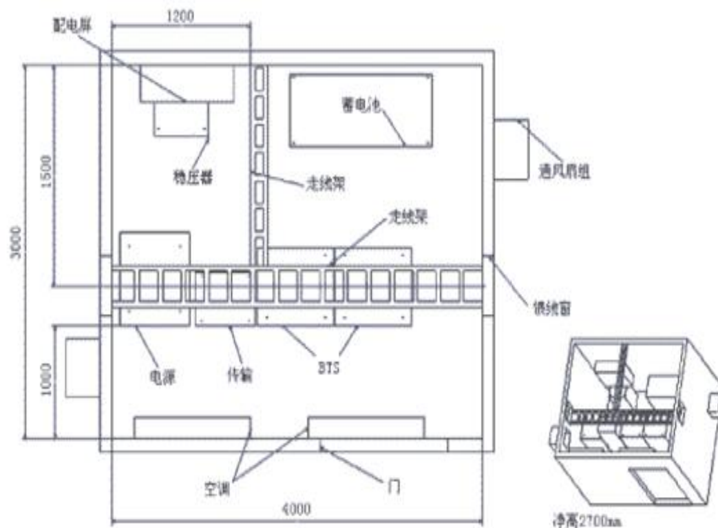
图 3-2-1 基站机房设备组成
