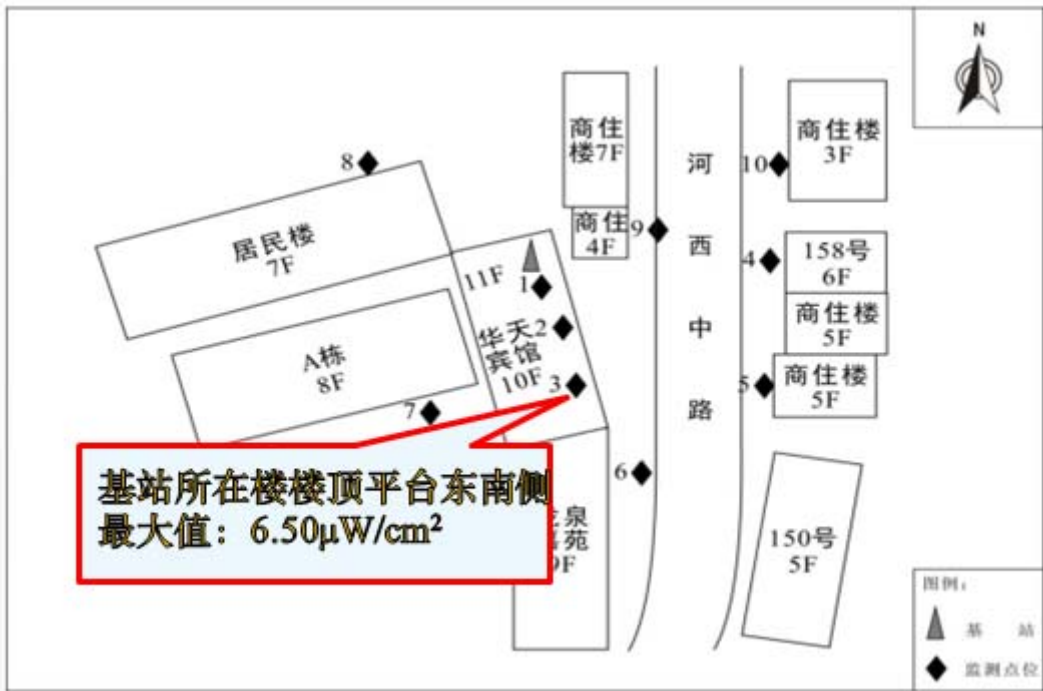
图 6-4 LFH-永顺县建华宾馆基站监测布点示意图
