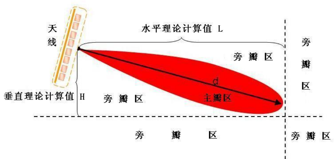
图 7-1 基站天线理论防护区
