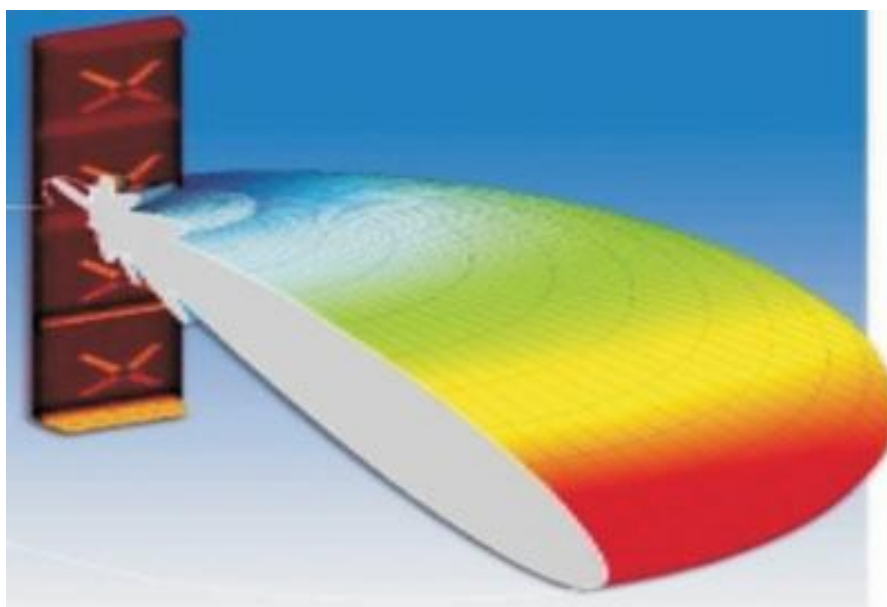
图 5-6 定向天线电磁波波束三维模拟图
