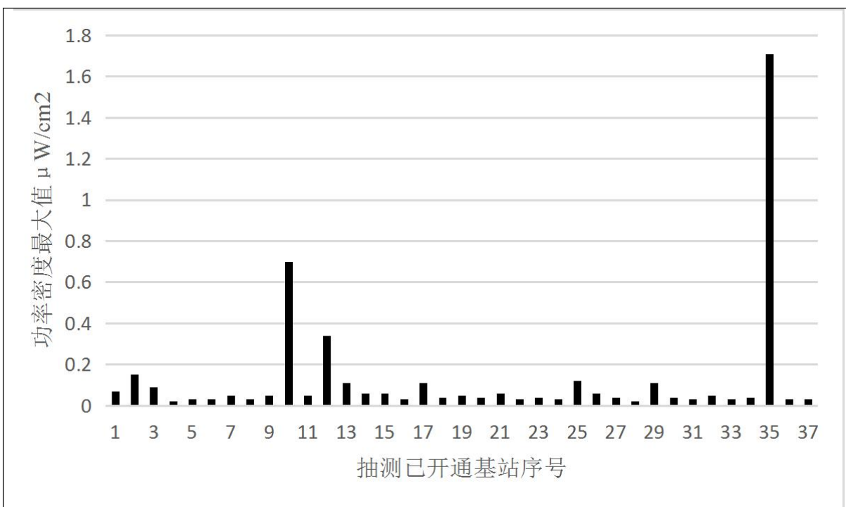
图 3-1 抽测基站电磁辐射测量最大值示意图
