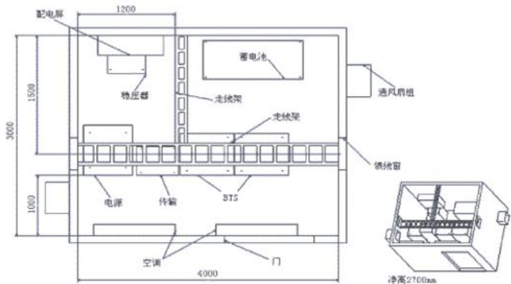
图 5-1 基站机房设备组成
