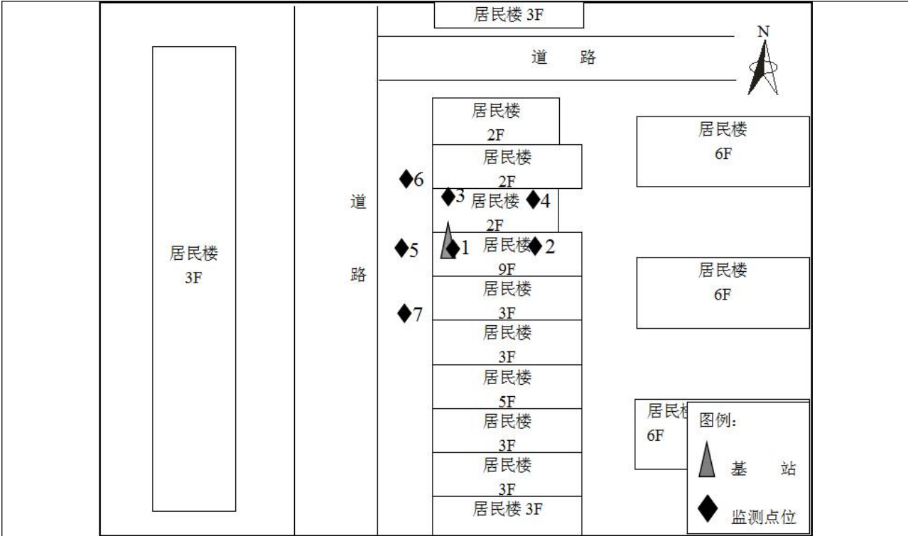
图 3-2-1 江华苍松西路口基站监测布点示意图
