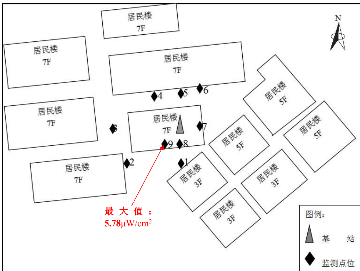
图 3-5-1 零陵区方圆小区基站监测布点示意图
