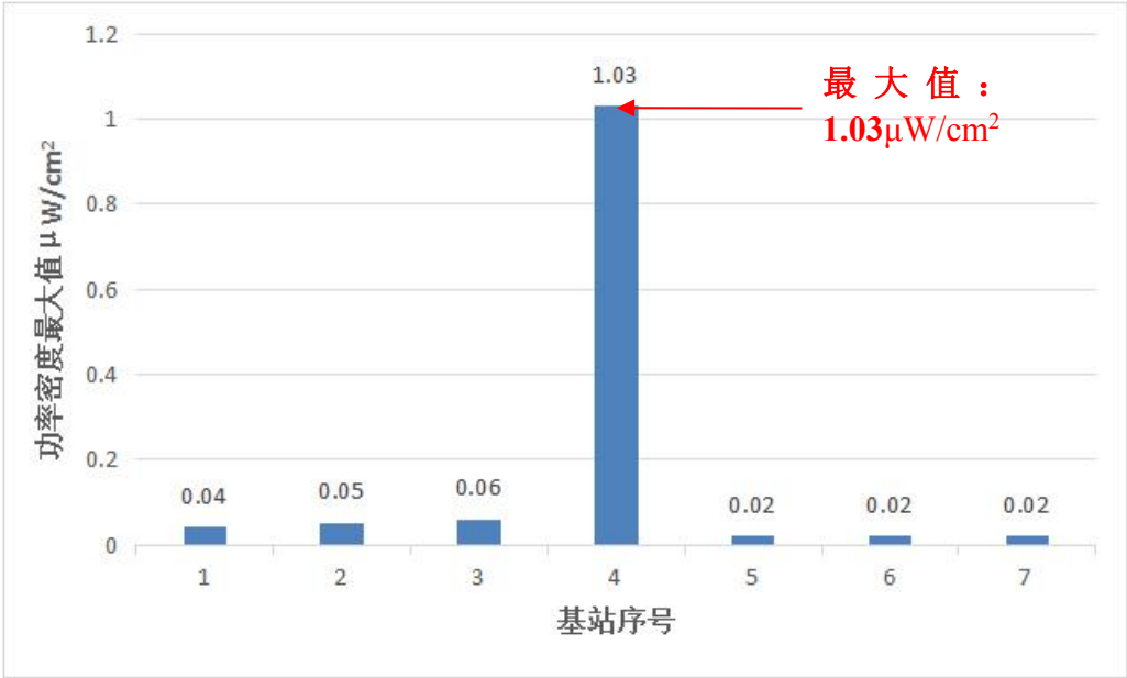
图 3-1 抽测未开通基站电磁辐射测量最大值统计柱状图
