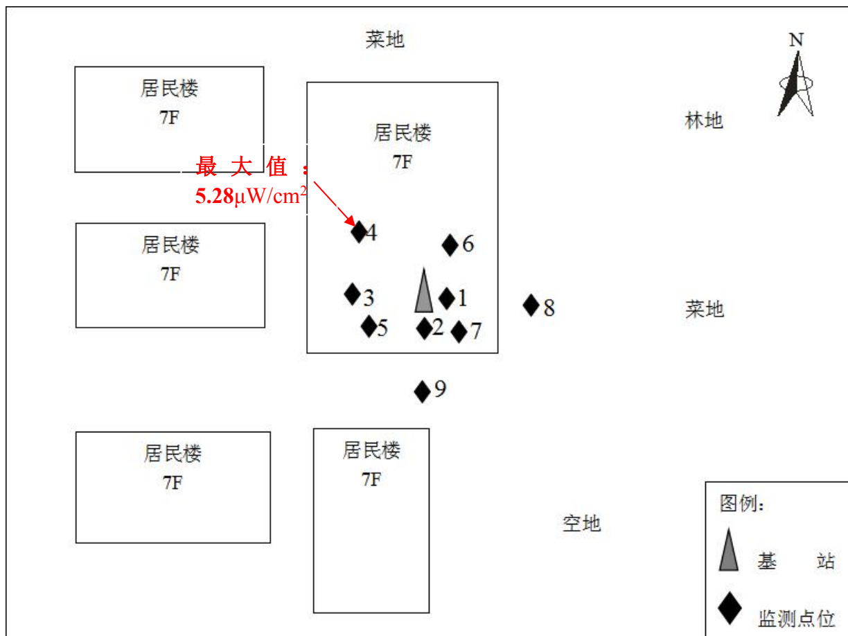
图 3-7-1 祁阳县盘龙路廉租房 1 基站监测布点示意图
