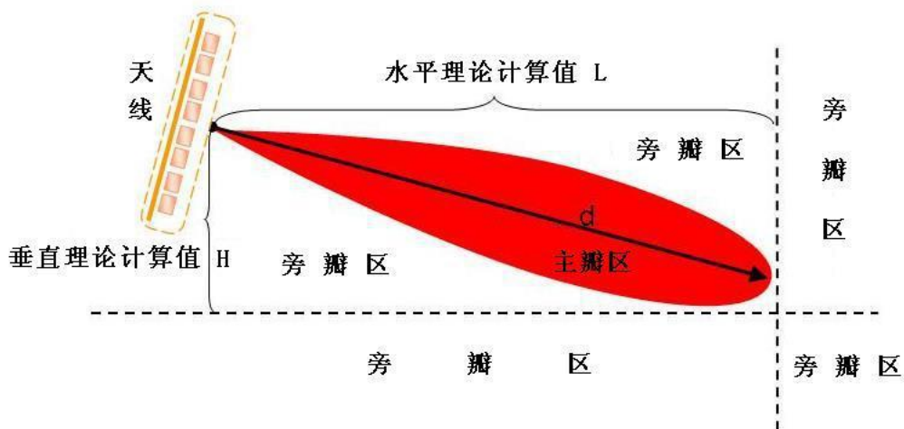
图 7-1 基站天线理论防护区
