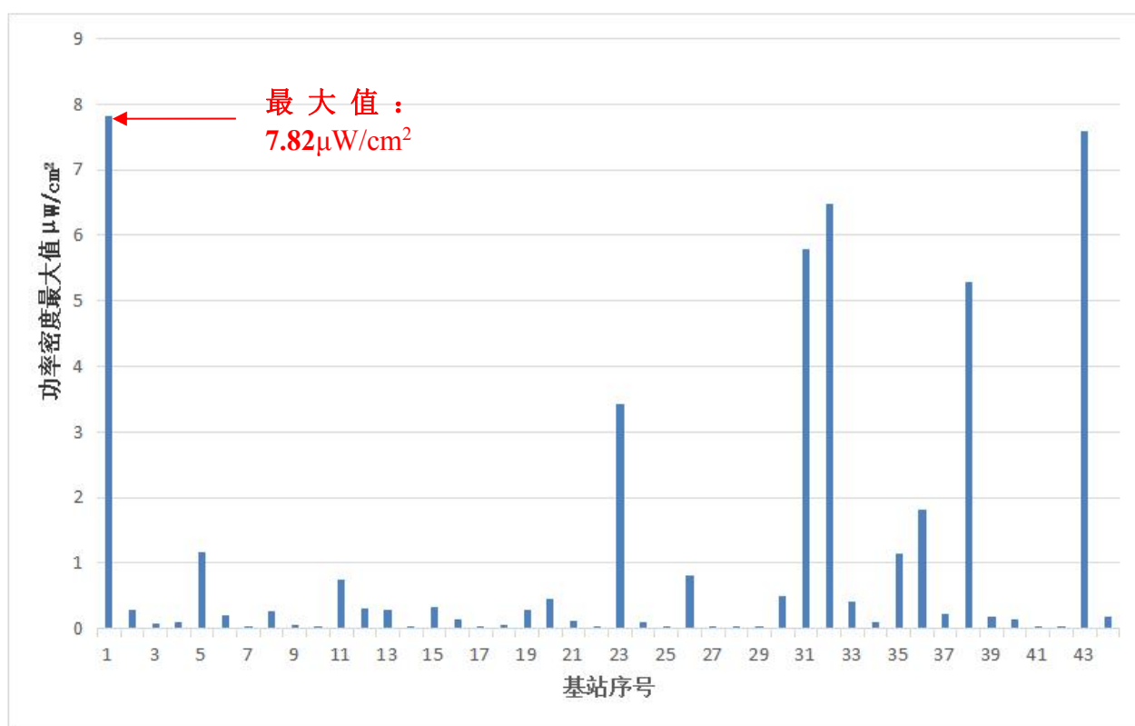
图 3-3 抽测已开通基站电磁辐射测量最大值统计柱状图
