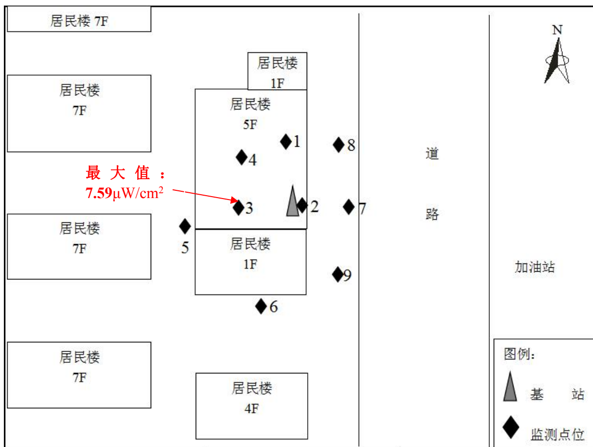
图 3-7-1 祁阳县腾龙实验学校基站监测布点示意图
