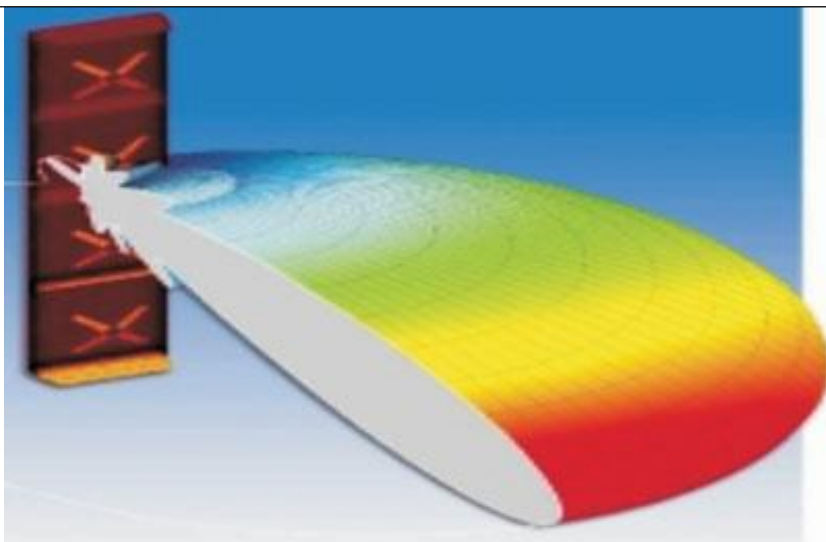
图 5-5 定向天线电磁波波束三维模拟图
