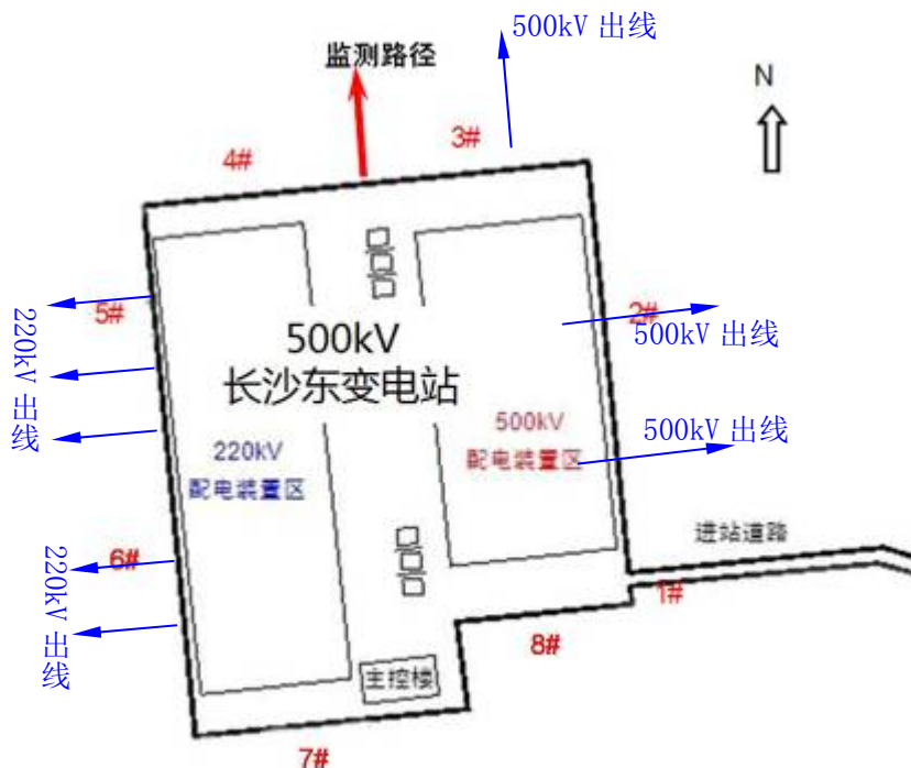
图 6-1 长沙东 500kV 变电站电磁环境影响类比监测布点图
