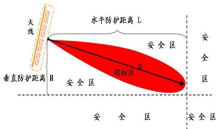
图 7-1 基站天线安全防护区
