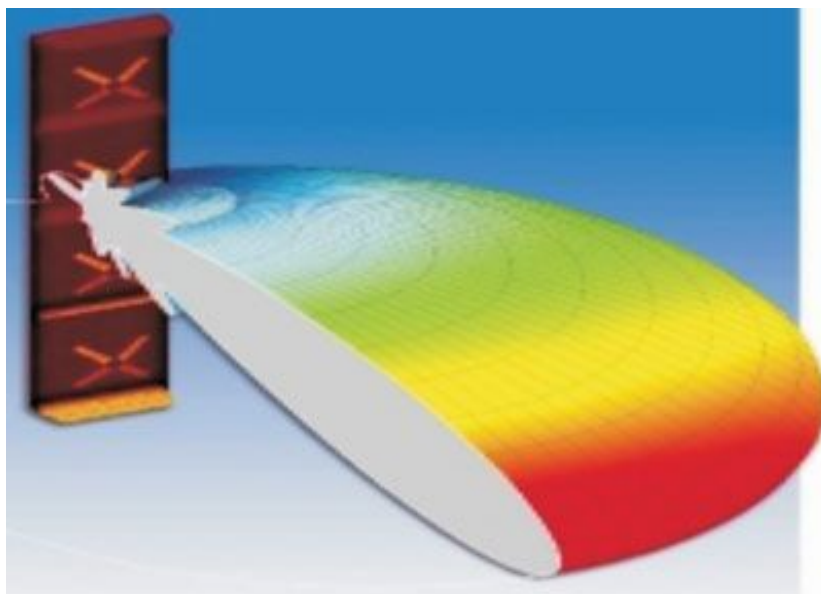
图 5-5 定向天线电磁波波束三维模拟图
