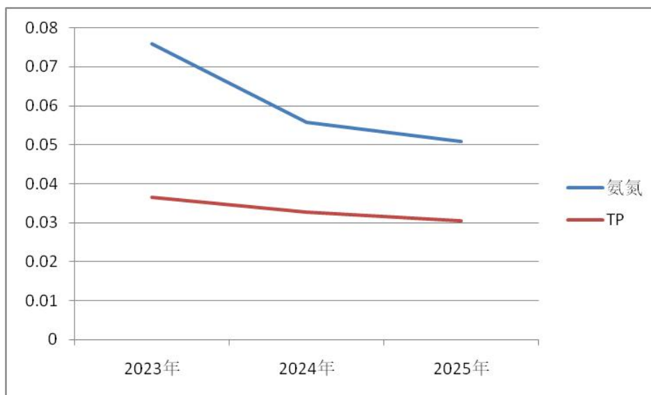
图 4.2-2 观音寺省控断面主要因子水环境变化特征
