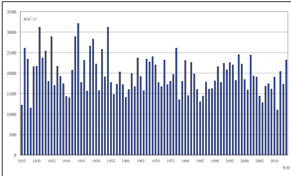
图 3.2-1 五强溪坝址年平均流量柱状图
