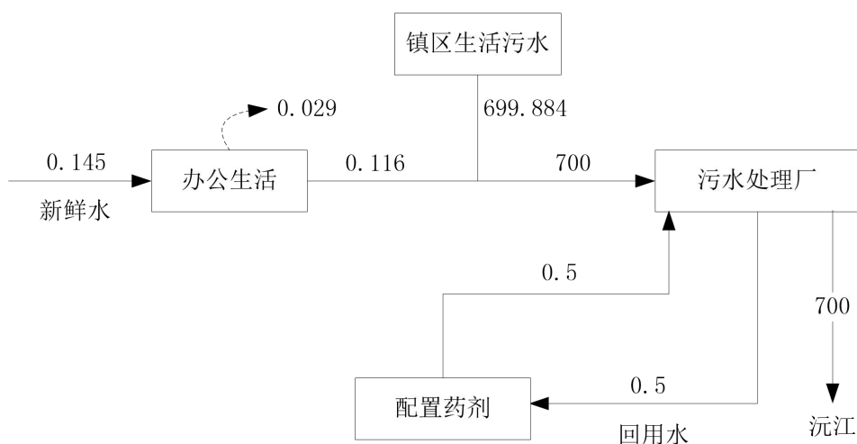
图 3.4-1 水平衡图 (t/d)
