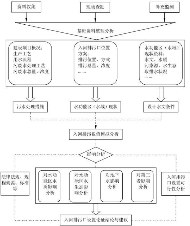
图 1.6-1 入河排污口论证工作程序框图
