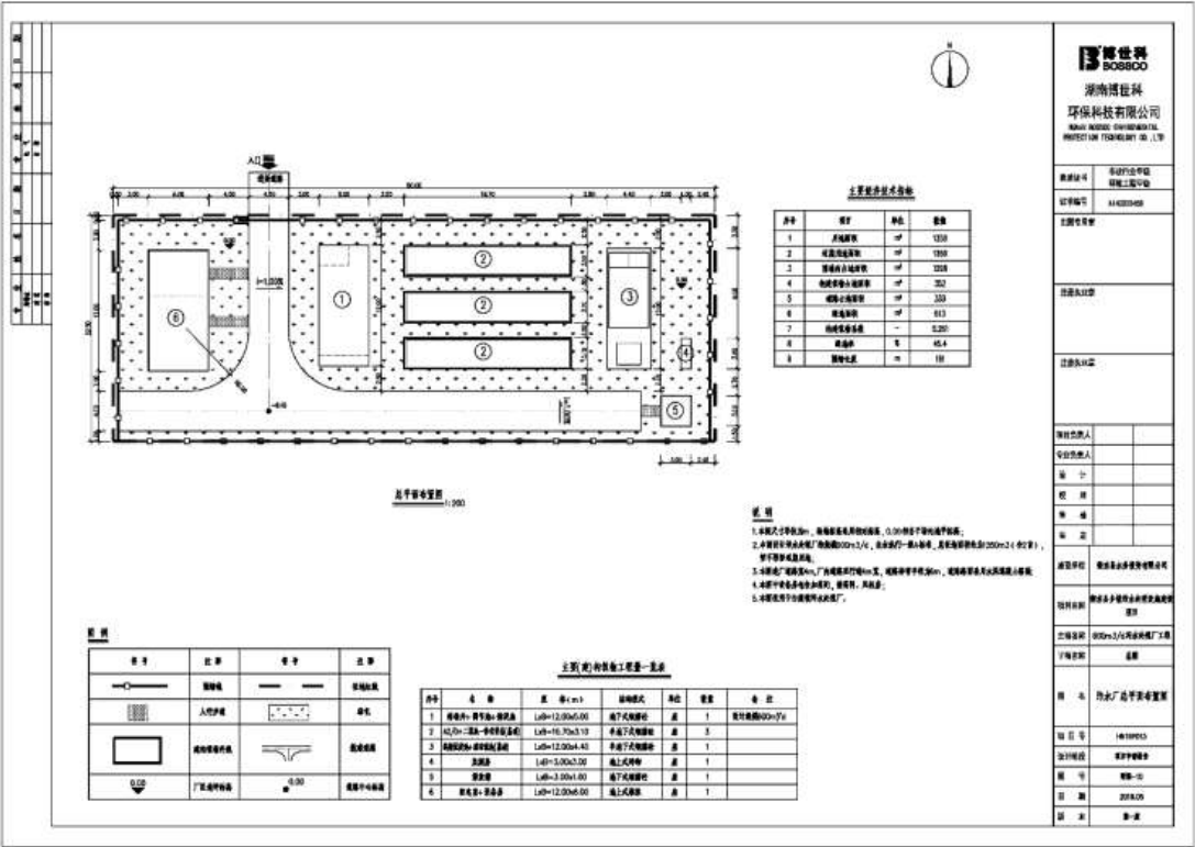
图 2.1-3 污水处理站总平面布置图
