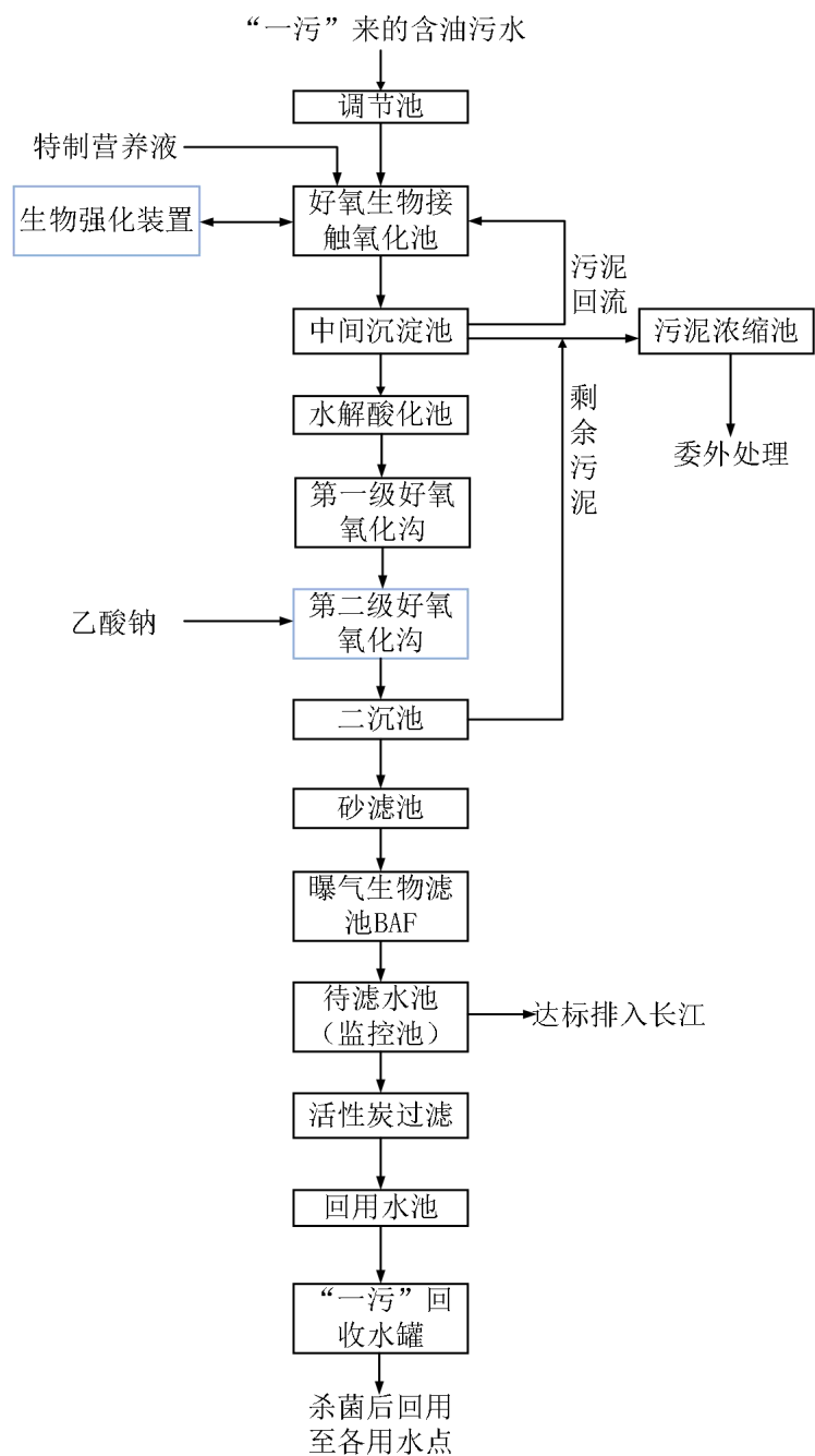
图 6.3-2 第二污水处理场含油废水处理工艺简要流程
