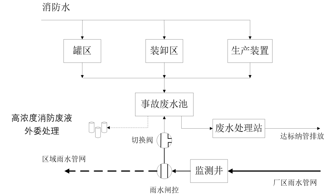
图 5.3.7-2 事故时污水收集管网示意图
