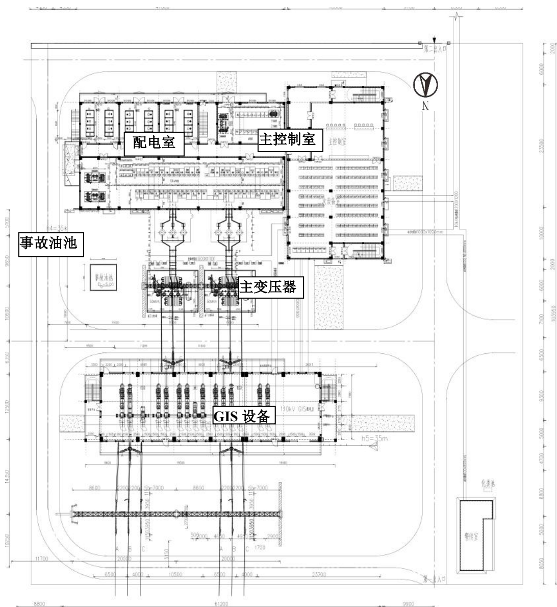
图 3.1-1 项目 110kV 变电站平面布置图
