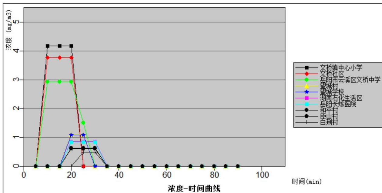
图 5.3.6-6b 主要关心点氯化亚砷浓度随时间变化情况图（最常见气象条件）
