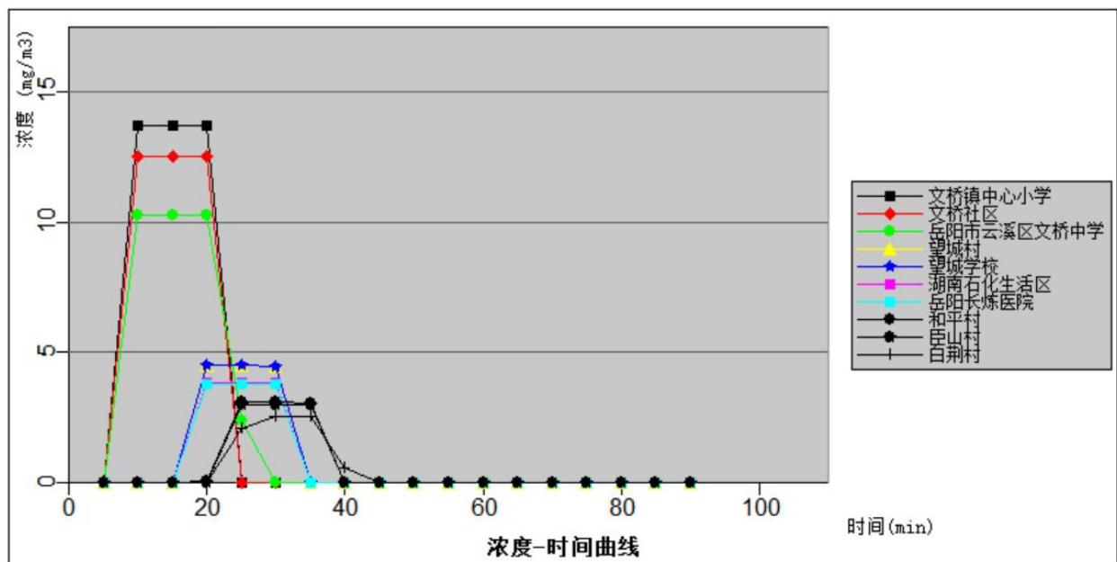
图 5.3.6-8a 主要关心点 HCl 浓度随时间变化情况图（最不利气象条件）
