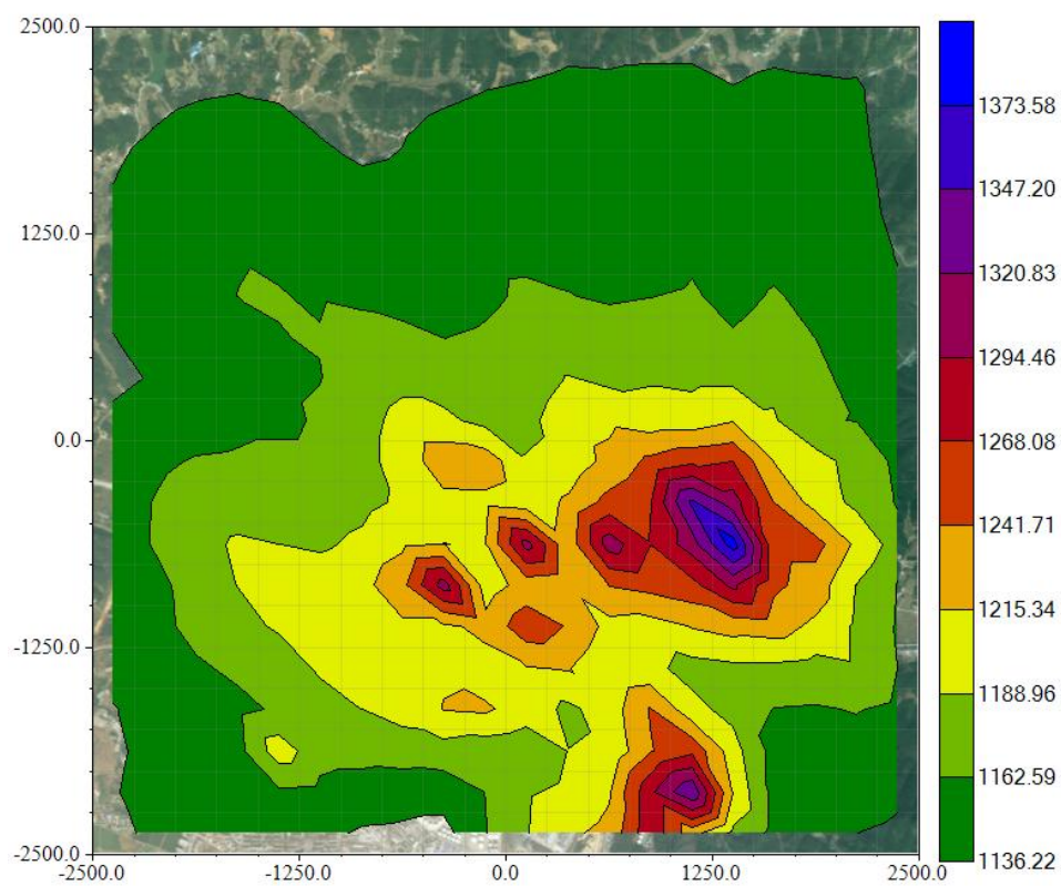
图 5.2.1.6-12 叠加后非甲烷总烃最大小时浓度影响 ( \mu\text{g}/\text{m}^3 )
