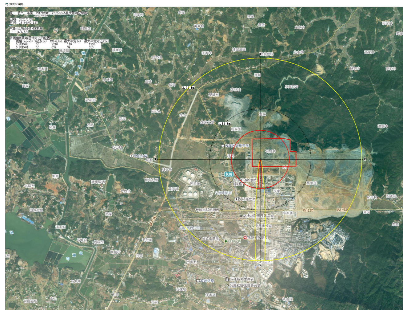
图 5.3.6-13a 氯气预测浓度达到不同毒性终点浓度的最大影响范围示意图(最不利气象条件)
