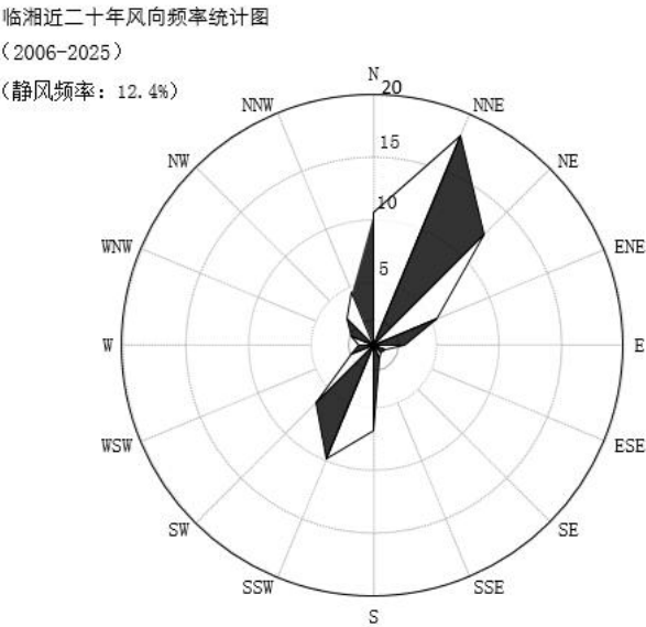
图 5.2.1.2-1 临湘站多年风向玫瑰图
