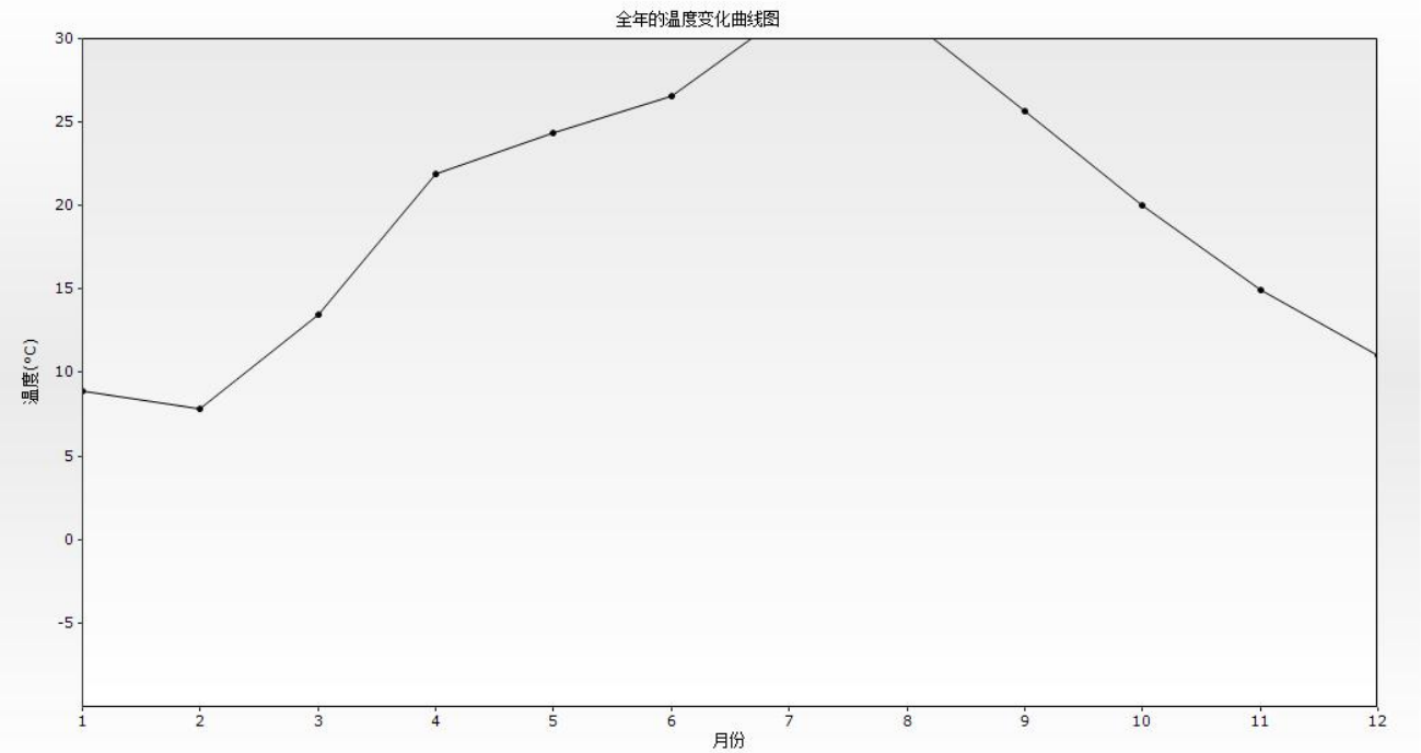
图 5.2.1.2-6 岳阳站 2025 年平均温度月变化曲线图
