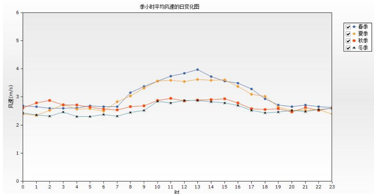
图 5.2.1.2-12 洪湖站 2025 年四季平均风速的日变化图
