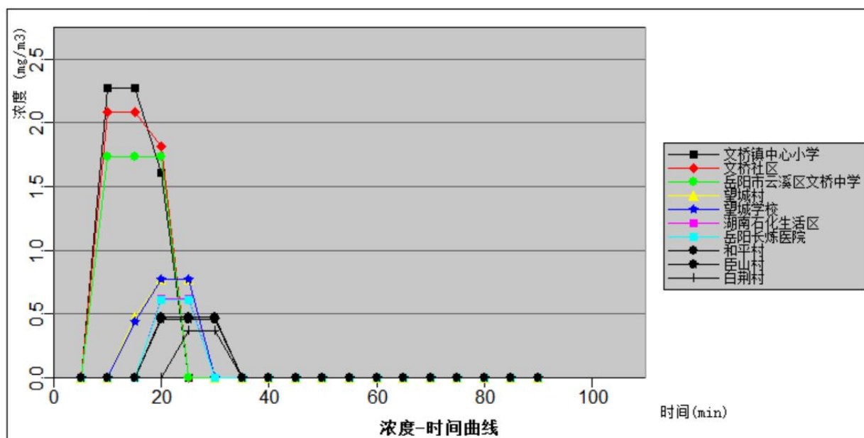
图 5.3.6-2b 主要关心点氯气浓度随时间变化情况图（最常见气象条件）
