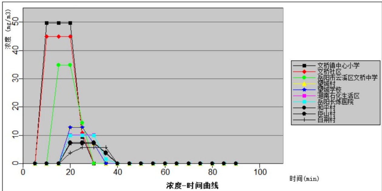
图 5.3.6-4b 主要关心点氯丙烯浓度随时间变化情况图（最常见气象条件）
