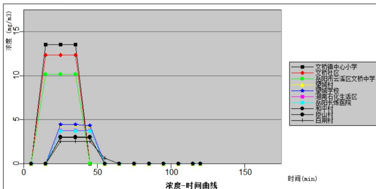
图 5.3.6-10a 主要关心点 CO 浓度随时间变化情况图（最不利气象条件）
