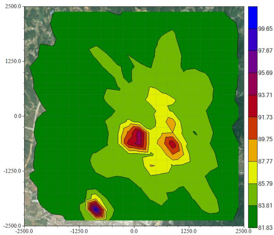
图 5.2.1.6-10 叠加后氨最大小时浓度影响 ( \mu\text{g}/\text{m}^3 )
