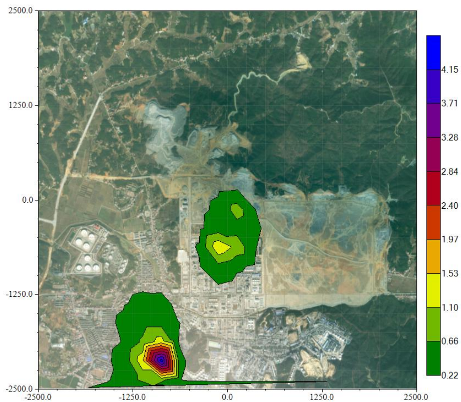
图 5.2.1.6-9 叠加后 TSP 最大日均浓度影响 ( \mu\text{g}/\text{m}^3 )
