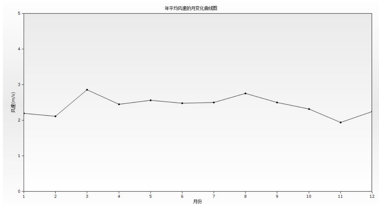
图 5.2.1.2-7 岳阳站 2025 年平均风速的月变化图
