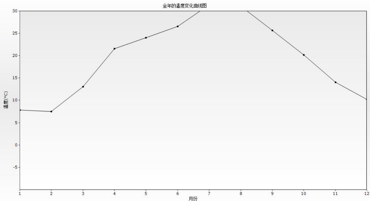
图 5.2.1.2-2 临湘站 2025 年平均温度月变化曲线图
