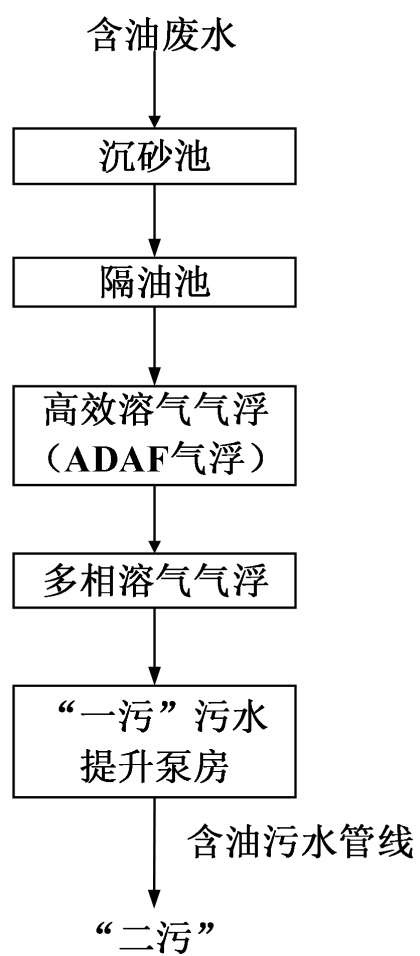
图 6.3-1 第一污水处理场含油废水处理工艺简要流程
