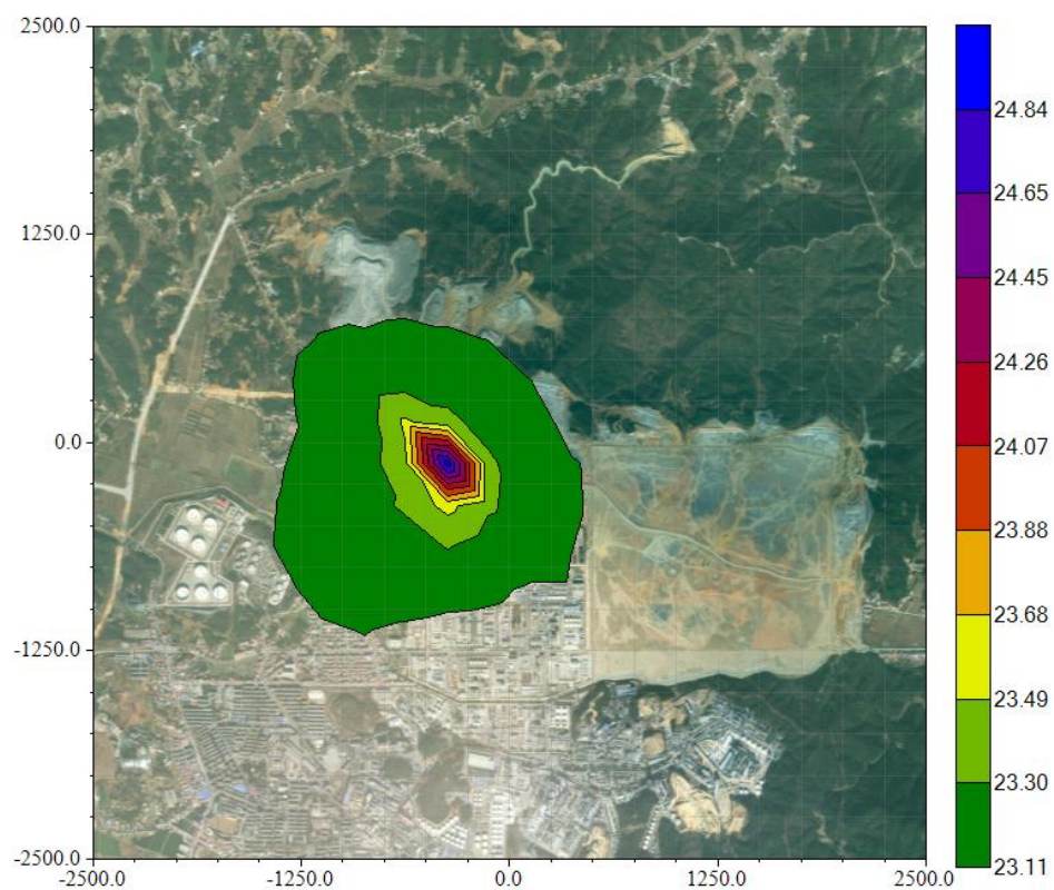
图 5.2.1.6-11 叠加后硫酸最大小时浓度影响 ( \mu\text{g}/\text{m}^3 )
