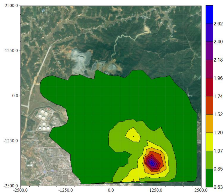
图 5.2.1.6-10 叠加后硫化氢最大小时浓度影响 ( \mu\text{g}/\text{m}^3 )
