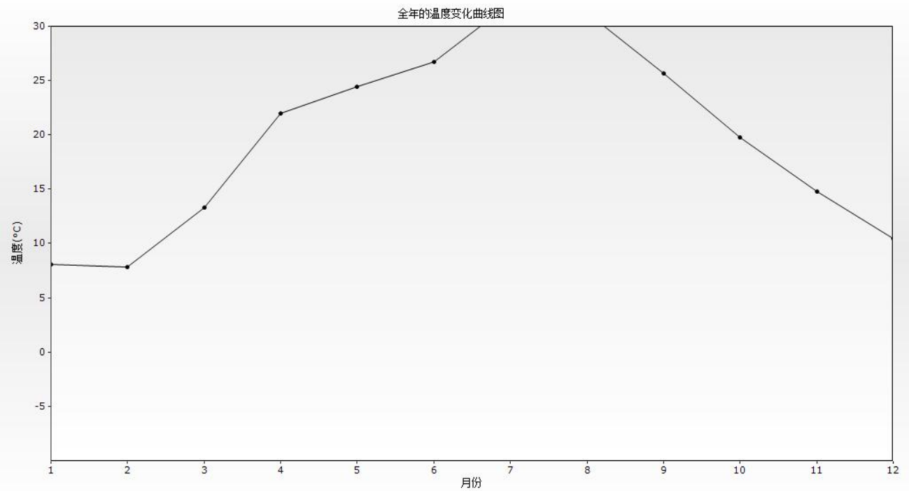
图 5.2.1.2-10 洪湖站 2025 年平均温度月变化曲线图
