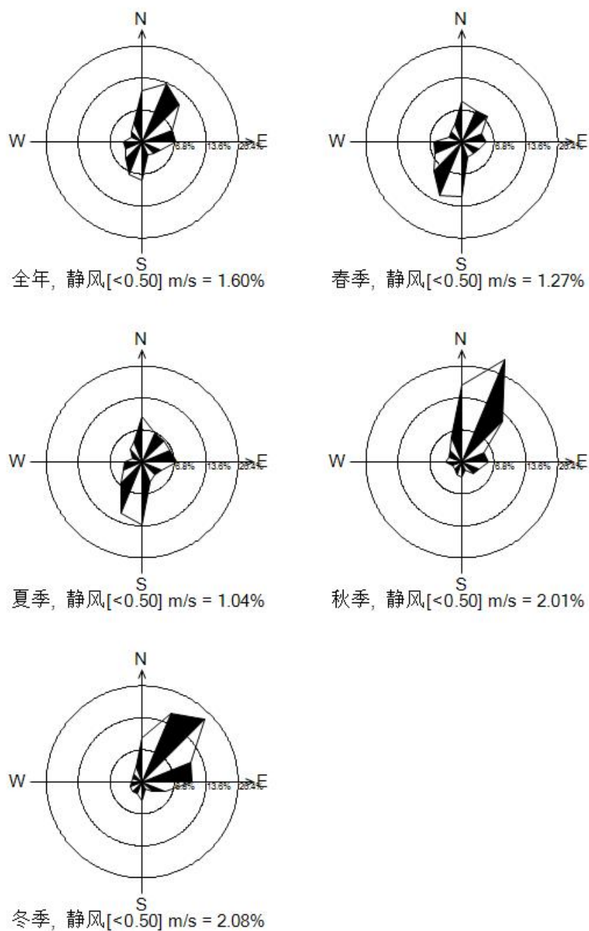
图 5.2.1.2-13 洪湖站 2025 年各季及全年风频玫瑰图
