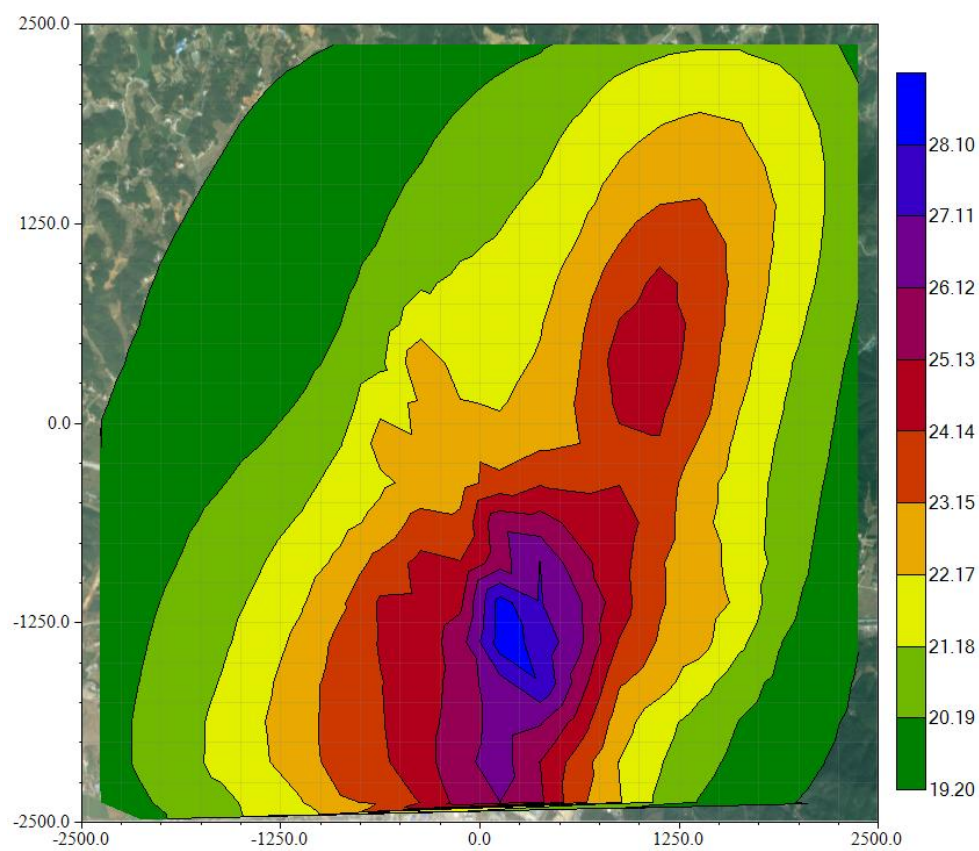
图 5.2.1.6-6 叠加后 NO 2 最大年均浓度影响 ( \mu\text{g}/\text{m}^3 )
