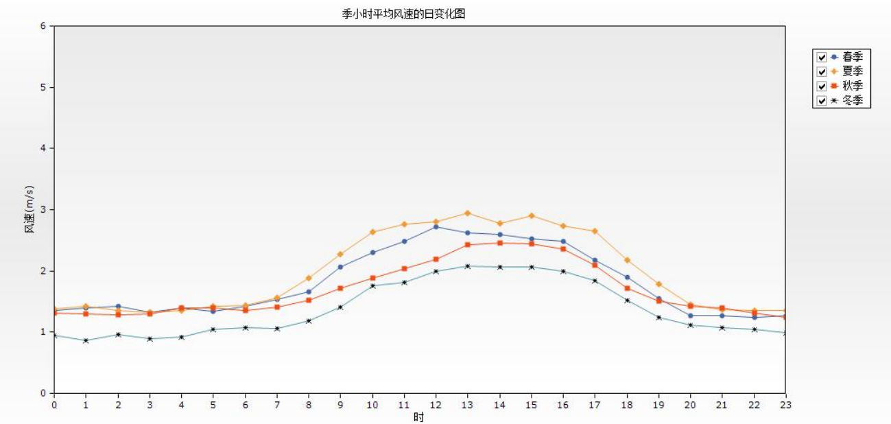
图 5.2.1.2-4 临湘站 2025 年四季平均风速的日变化图
