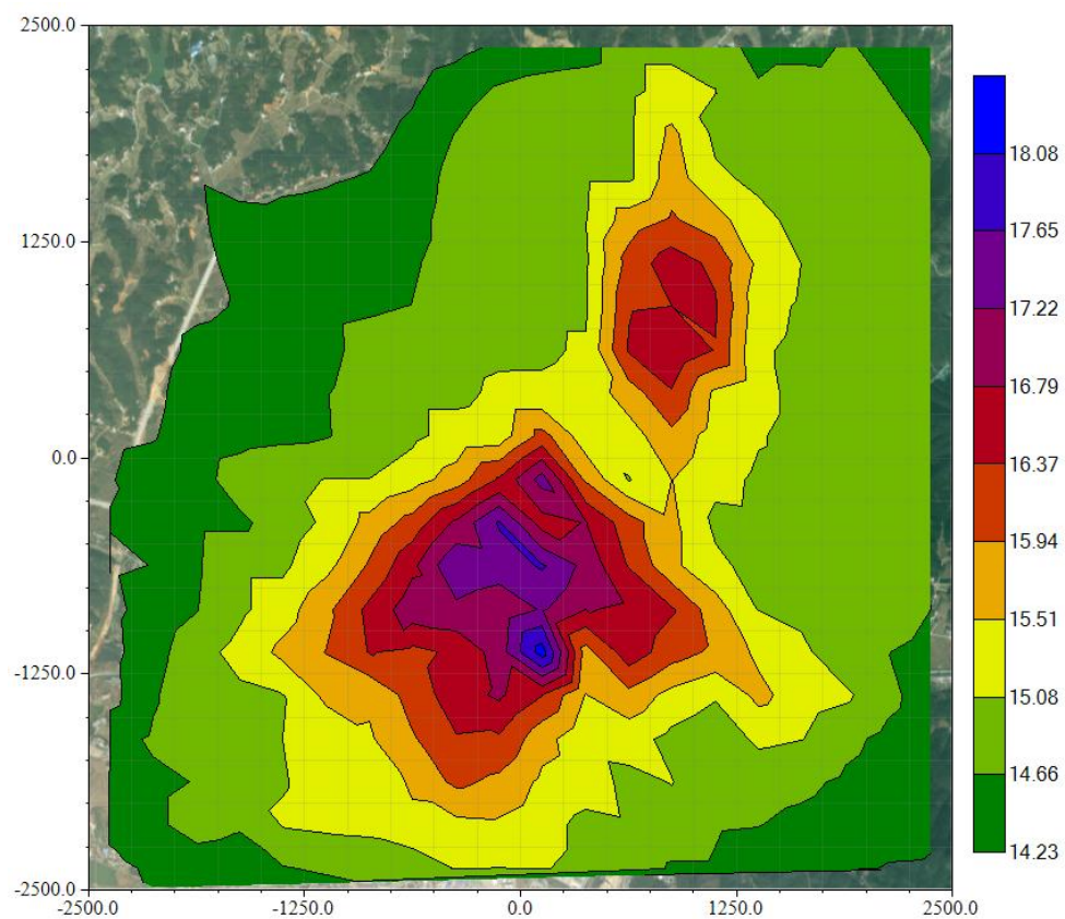
图 5.2.1.6-3 叠加后 \text{SO}_2 最大日均 (98%保证率) 浓度影响 ( \mu\text{g}/\text{m}^3 )
