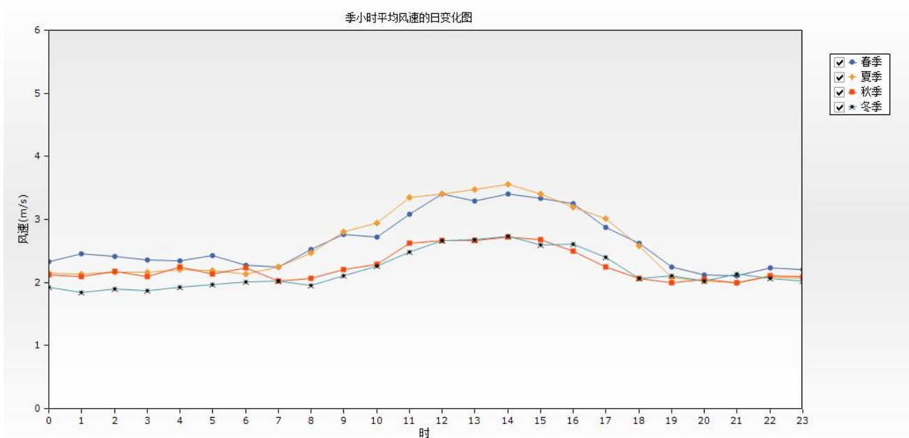
图 5.2.1.2-8 岳阳站 2025 年四季平均风速的日变化图
