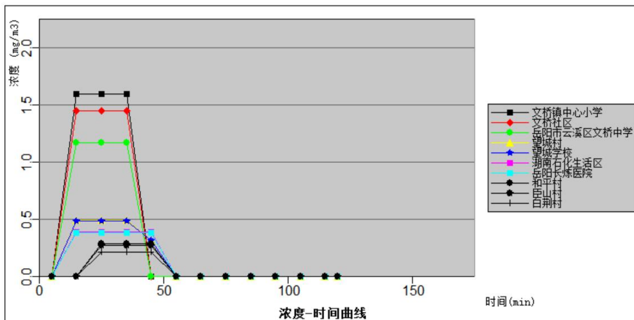
图 5.3.6-12b 主要关心点 HCl 浓度随时间变化情况图（最常见气象条件）
