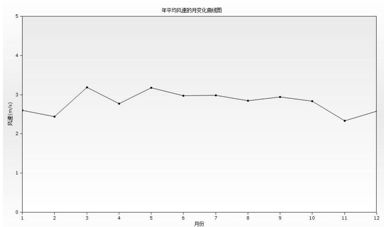
图 5.2.1.2-11 洪湖站 2025 年平均风速的月变化图
