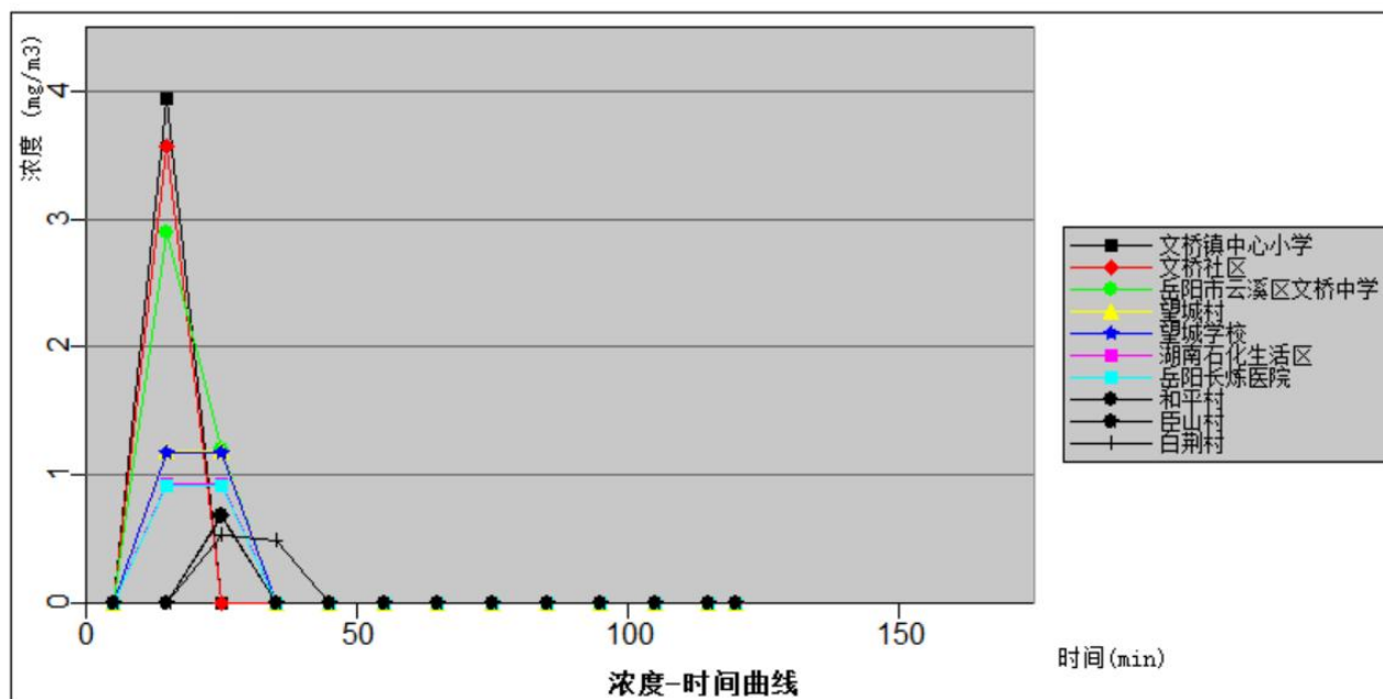
图 5.3.6-14b 主要关心点氯气浓度随时间变化情况图（最常见气象条件）
