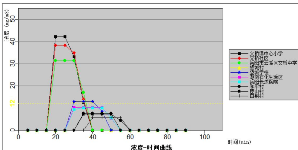
图 5.3.6-6a 主要关心点氯化亚砷浓度随时间变化情况图（最不利气象条件）
