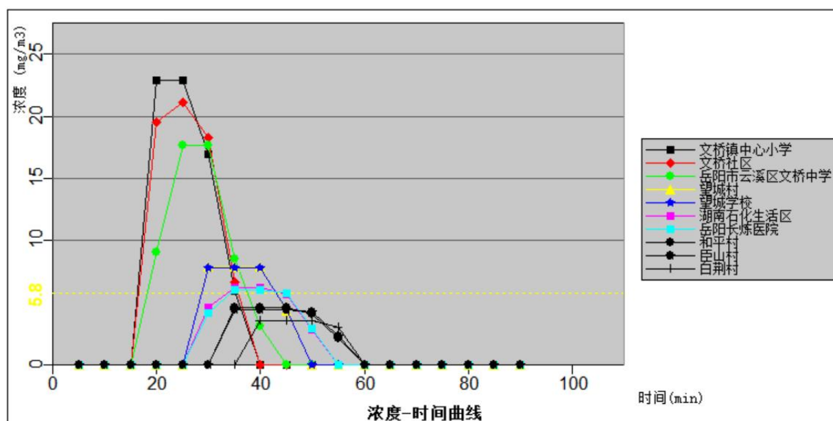
图 5.3.6-2a 主要关心点氯气浓度随时间变化情况图（最不利气象条件）
