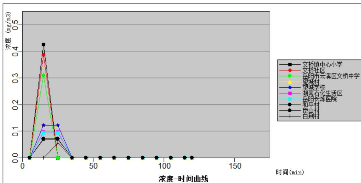
图 5.3.6-16b 主要关心点 SO 2 浓度随时间变化情况图（最常见气象条件）
