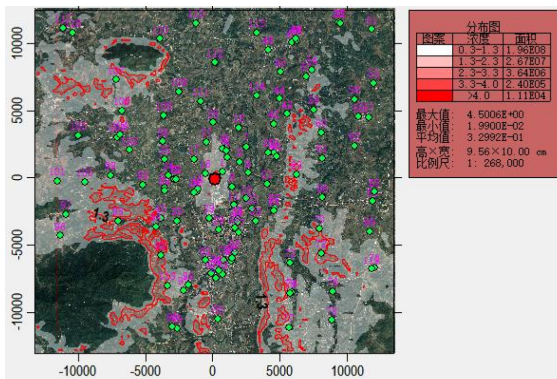
图 7.2-17 正常工况下 SO 2 24 小时平均浓度贡献值分布图
