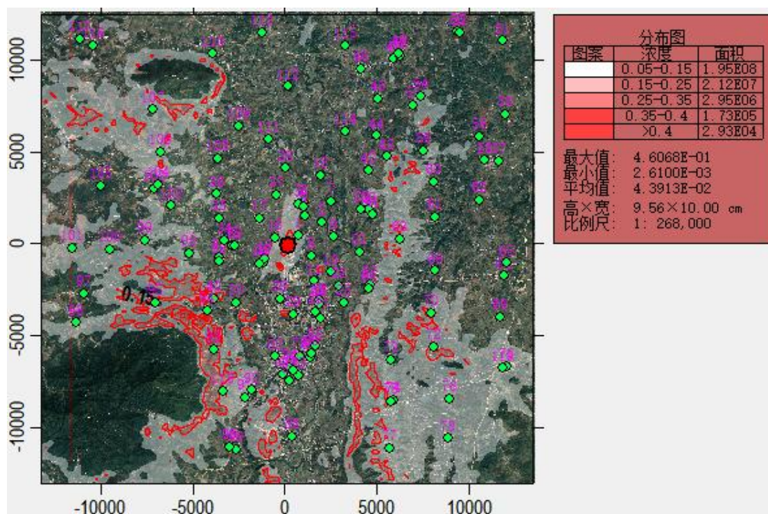
图 7.2-30 正常工况下氟化物 24 小时平均浓度贡献值分布图
