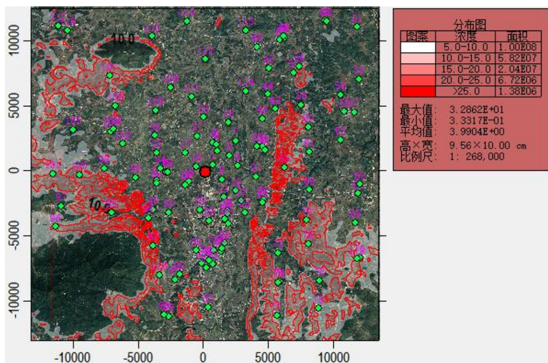
图 7.2-16 正常工况下 SO 2 1 小时平均浓度贡献值分布图
