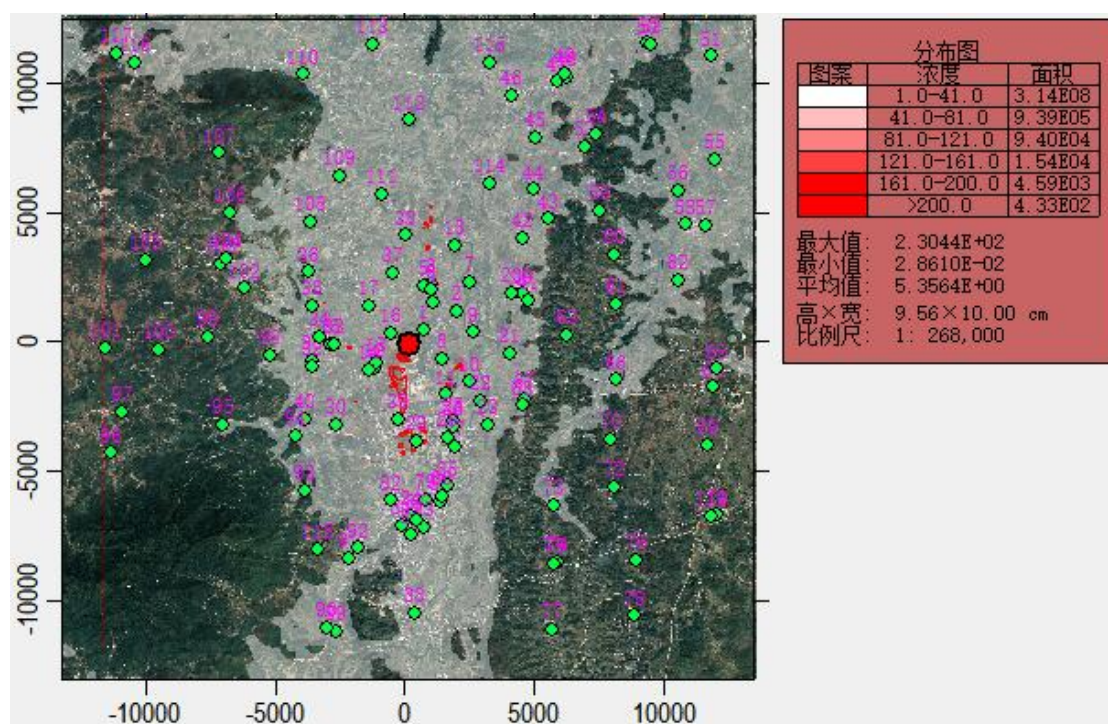
图 7.2-22 正常工况下 TSP24 小时平均浓度贡献值分布图
