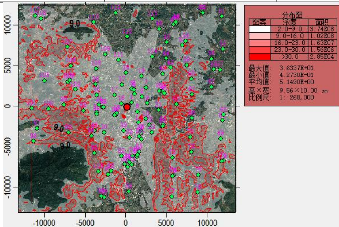
图 7.2-19 正常工况下 NO 2 1 小时平均浓度贡献值分布图
