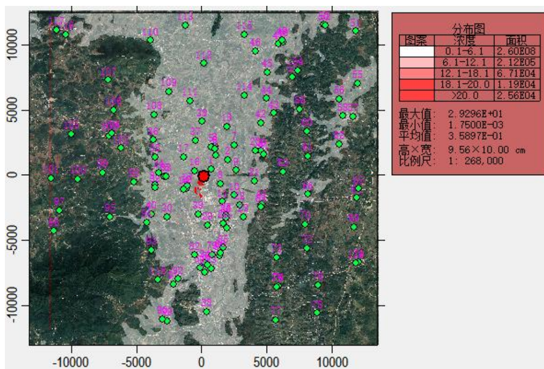
图 7.2-23 正常工况下 TSP 年平均浓度贡献值分布图
