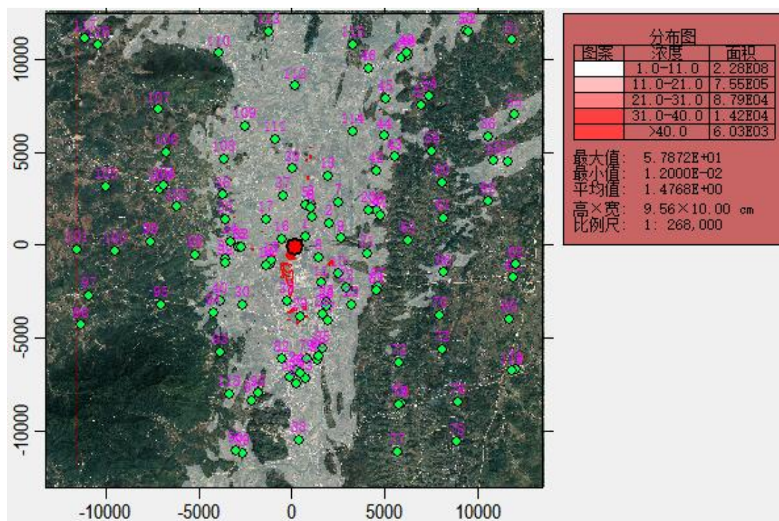
图 7.2-26 正常工况下 PM 2.5 24 小时平均浓度贡献值分布图
