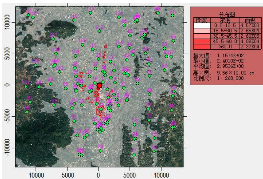
图 7.2-24 正常工况下 PM_{10} 24 小时平均浓度贡献值分布图
