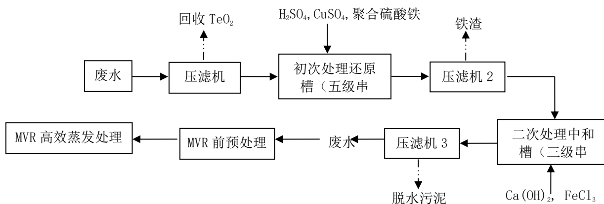
图 9.2.1-1 碲化工废水处理工艺流程图
