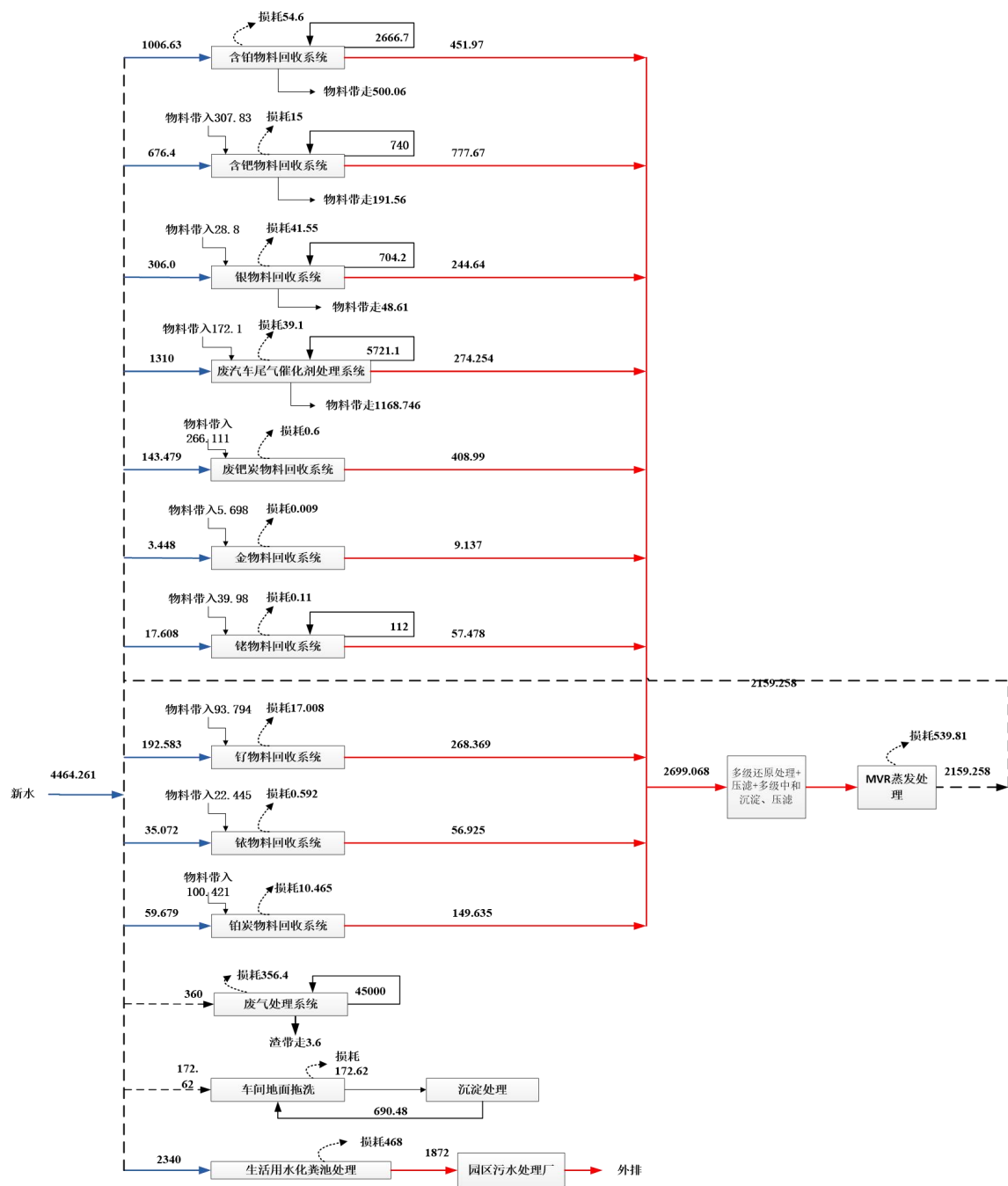
图 5.2-1 本项目水平衡图
