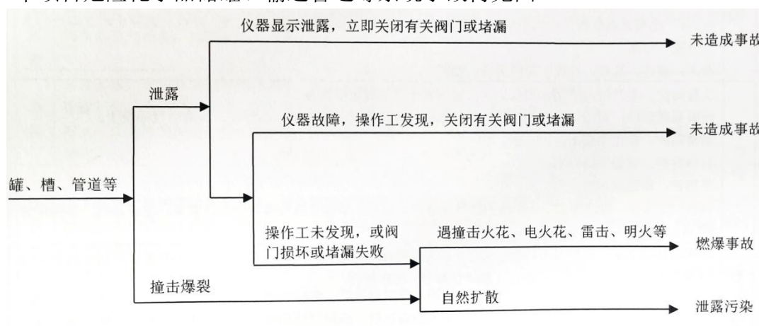
图 10.5-1 本项目事故树示意图
