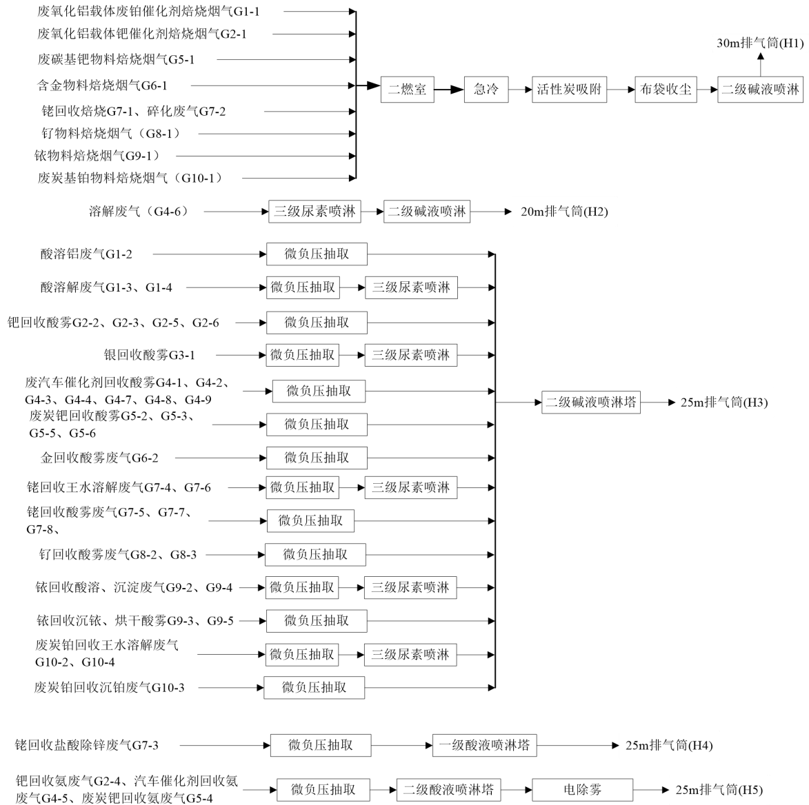
图 5.3.2-1 本项目有组织废气处理及排放去向图
