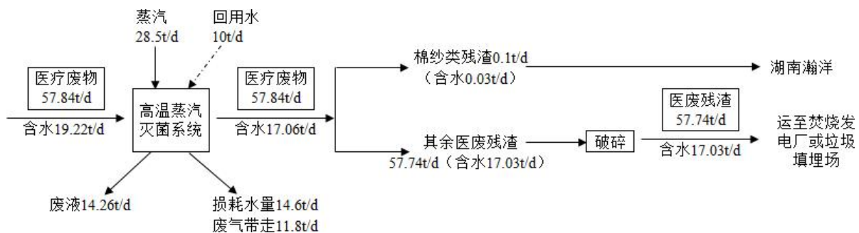
图 3.2-2 项目物料平衡分析图
