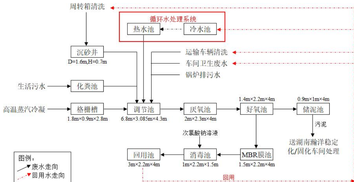
图 5.2-7 废水走向示意图
