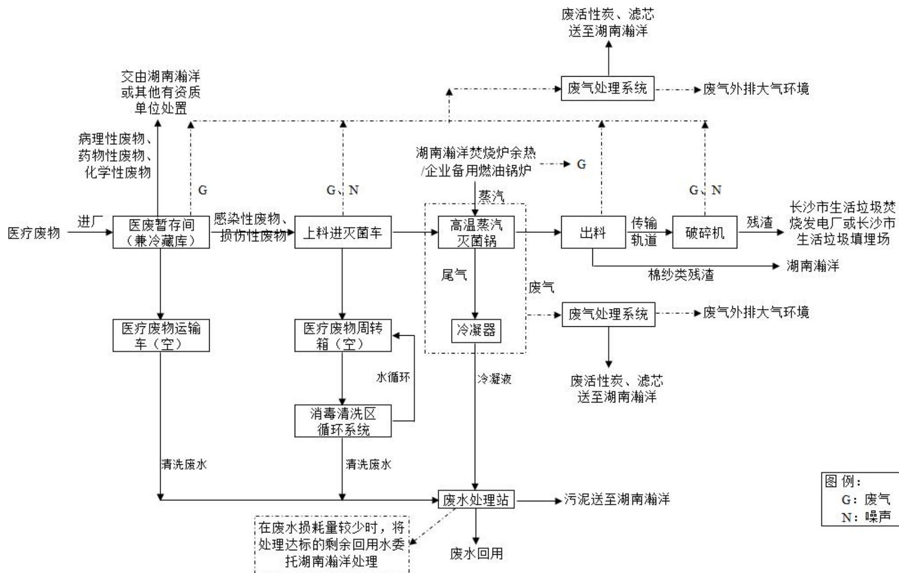
图 3.2-1 医疗废物高温蒸汽处理系统工艺流程及产污节点图
