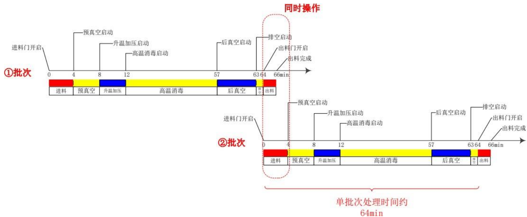
图 3.1-2 高温蒸煮全过程示意图
