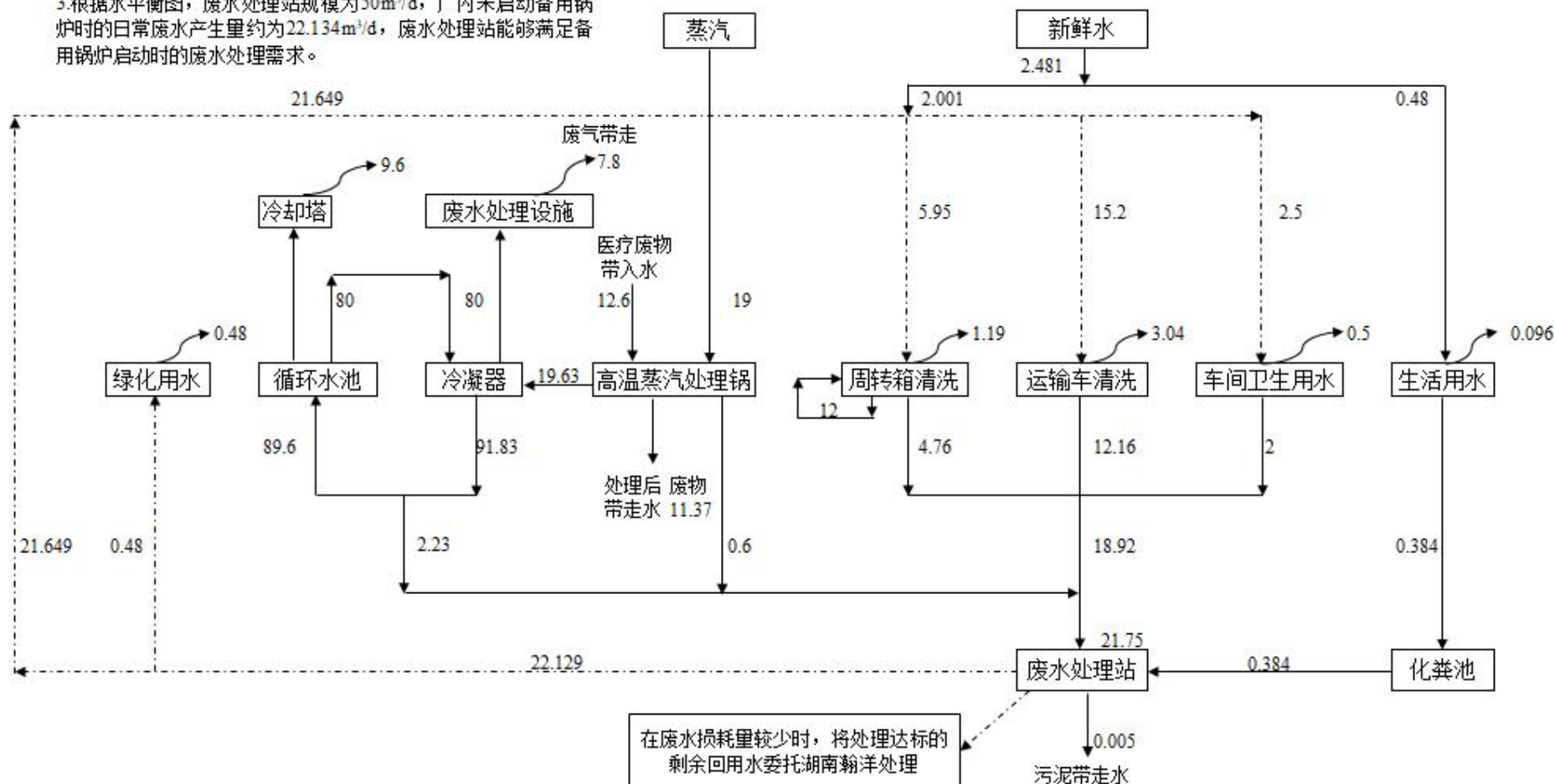
图 3.1-3 现有工程生产工序水平衡分析图 单位: \text{m}^3/\text{d}
