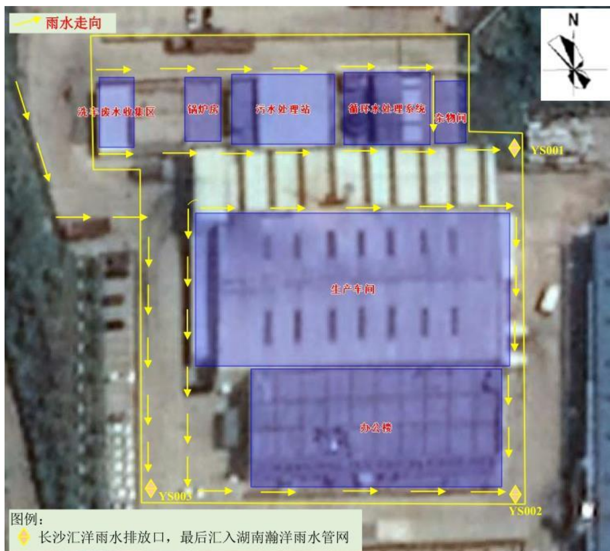
图 3.2-5 厂区雨水流向示意图
