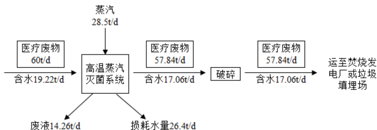
图 3.2-2 项目物料平衡分析图
