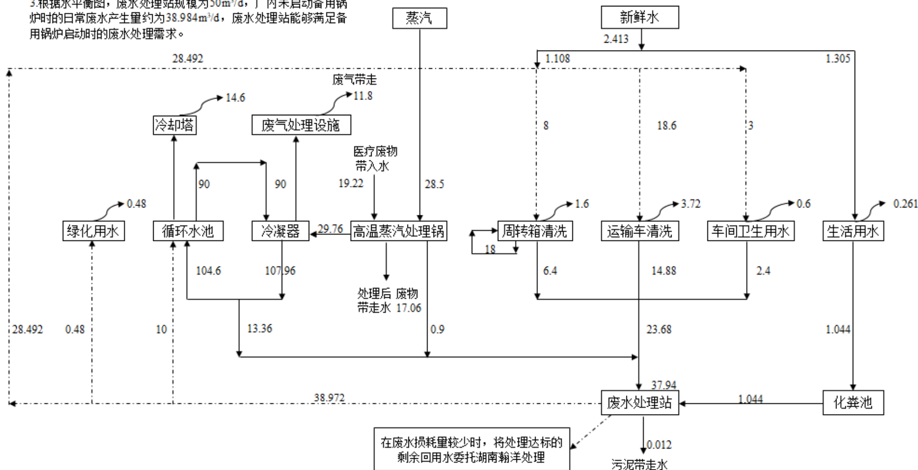
图 3.2-3 项目生产工序水平衡分析图 单位：m 3 /d
