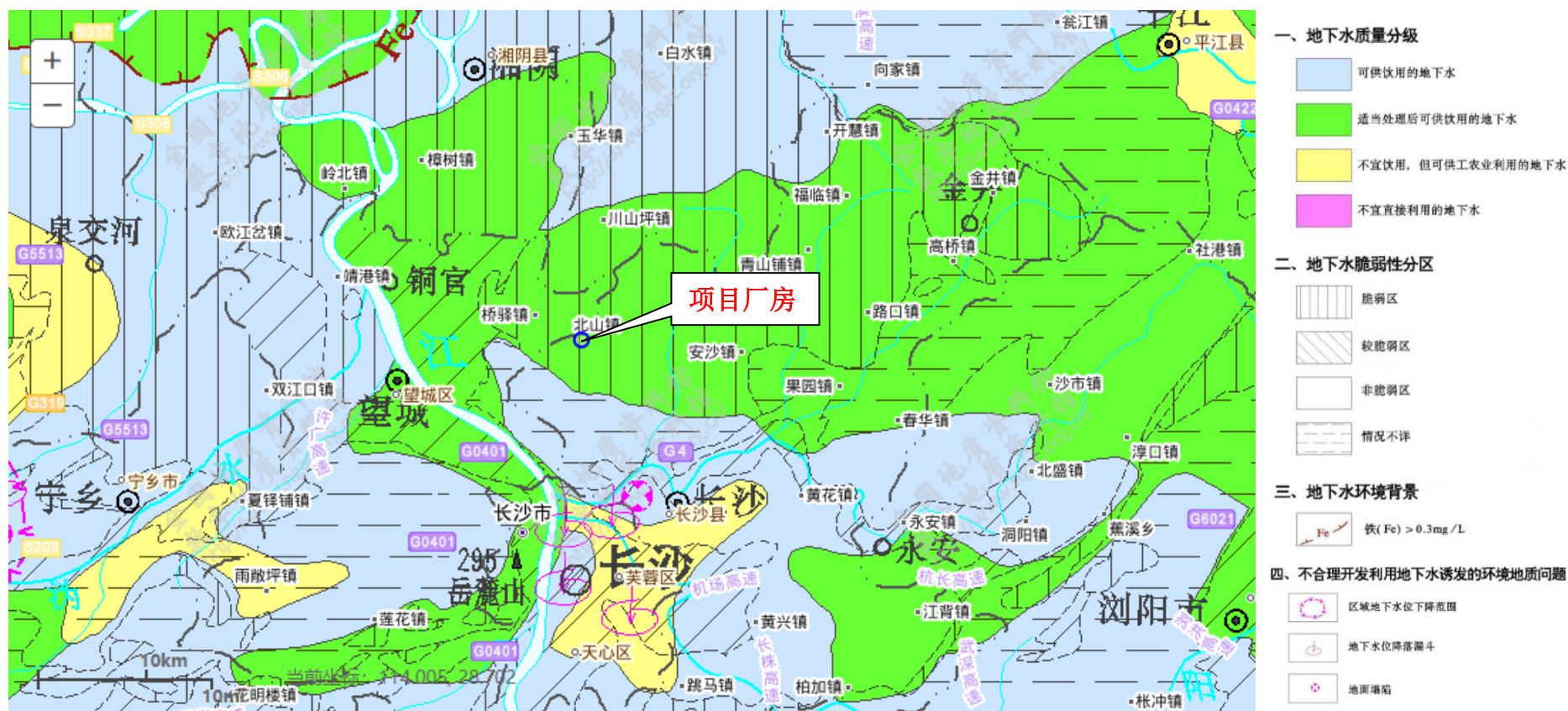
附图 7：水文地质图（1:50000）
