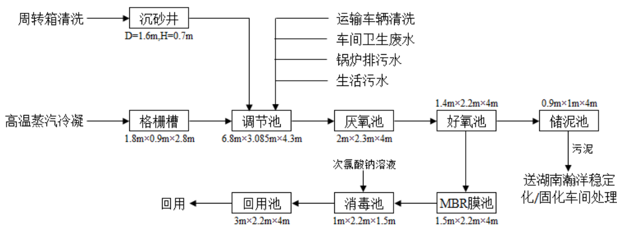
图 6.2-1 废水走向示意图
