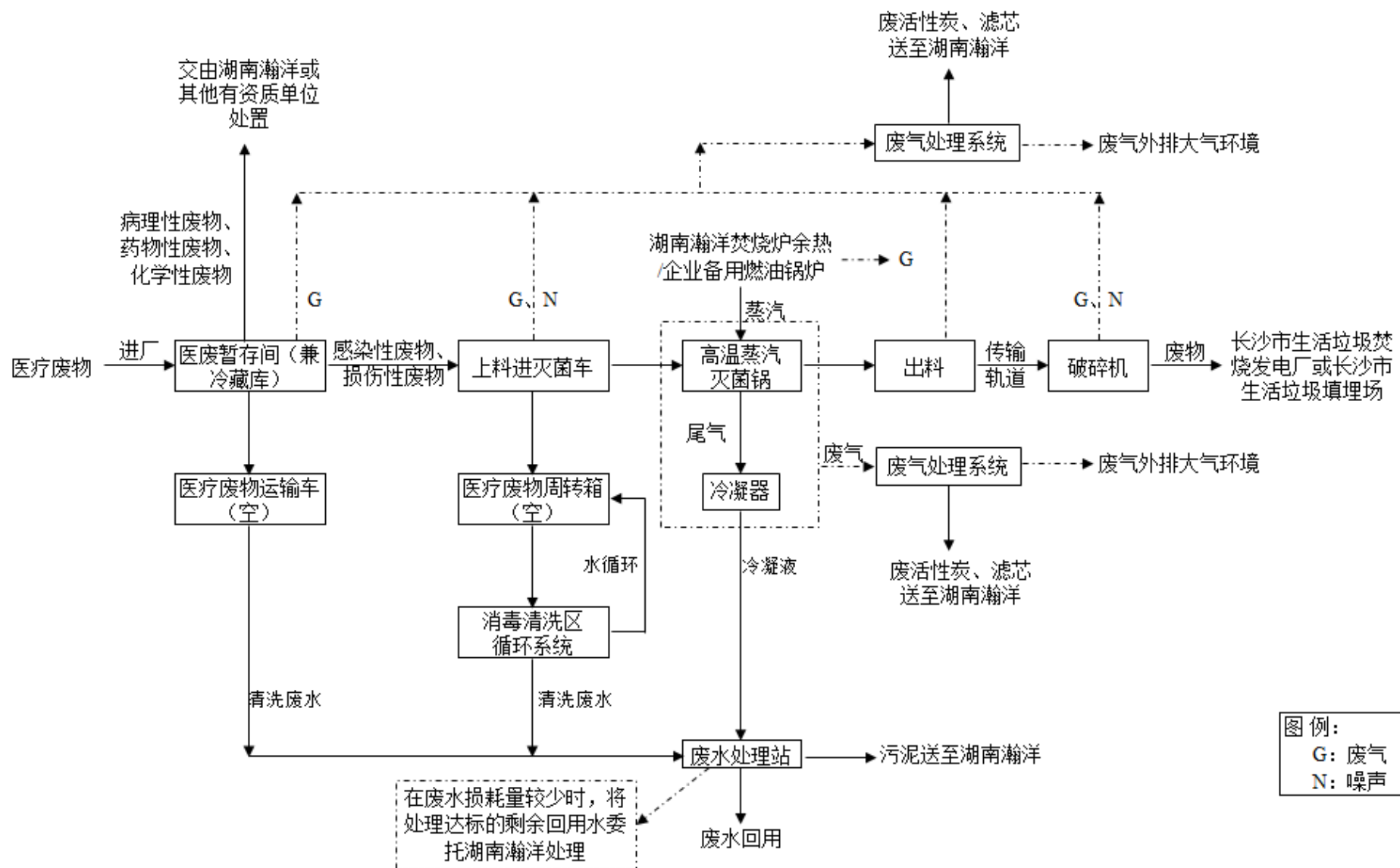
图 3.2-1 医疗废物高温蒸汽处理系统工艺流程及产污节点图
