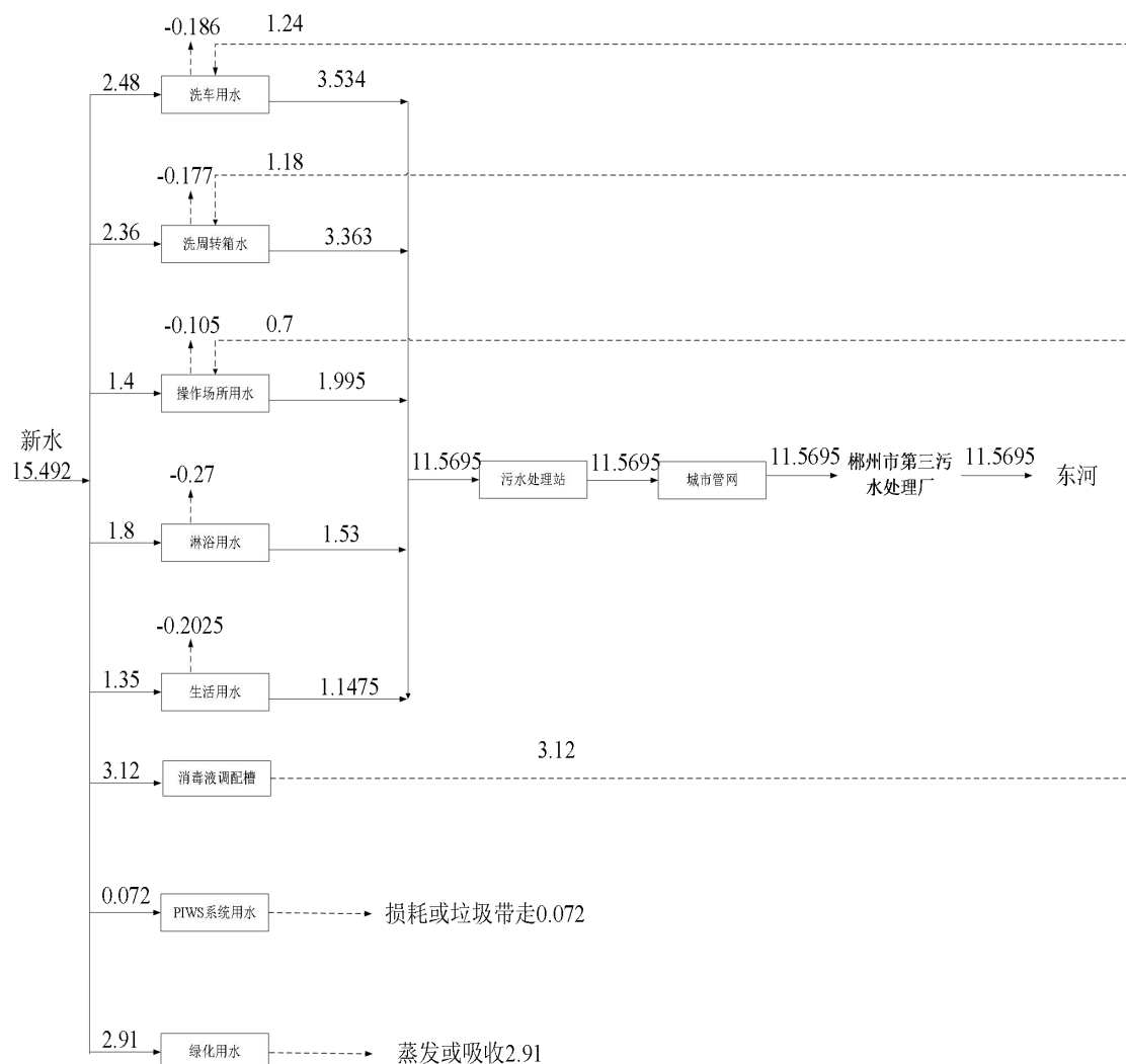
图 2.2.2-1 现有工程水平衡图 单位：m³/d
