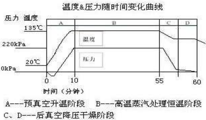
图 3.2-2 高温蒸汽处理工艺周期
