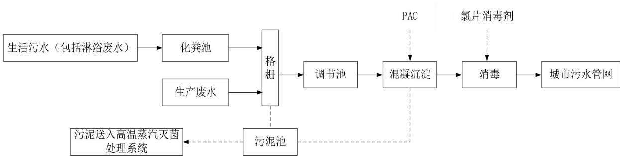
图 8.5.3-1 污水处理工艺流程图
