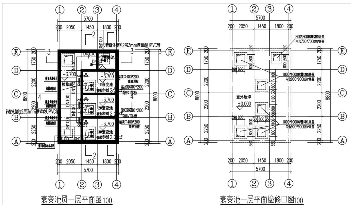
图 10-6 衰变池平面图
