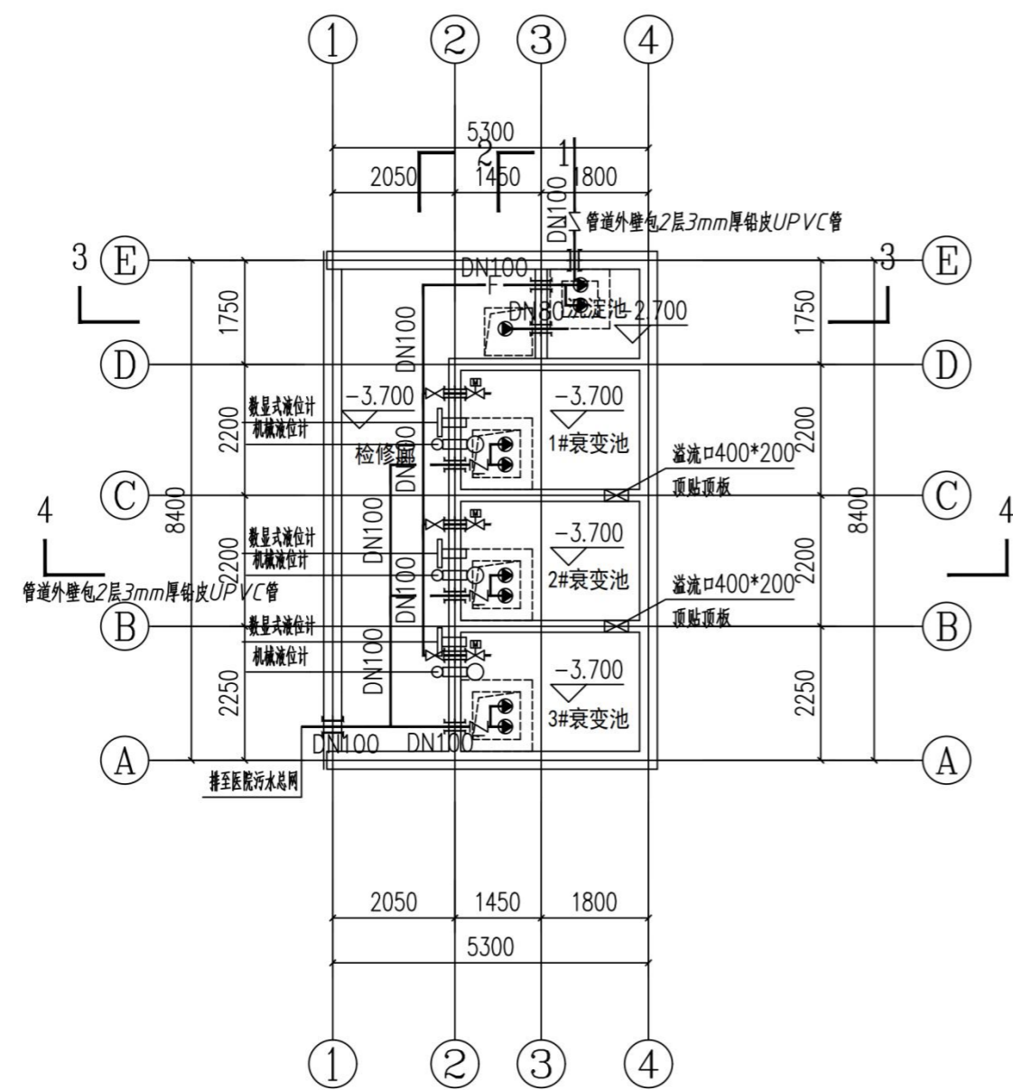
衰变池负一层平面图 1:100
