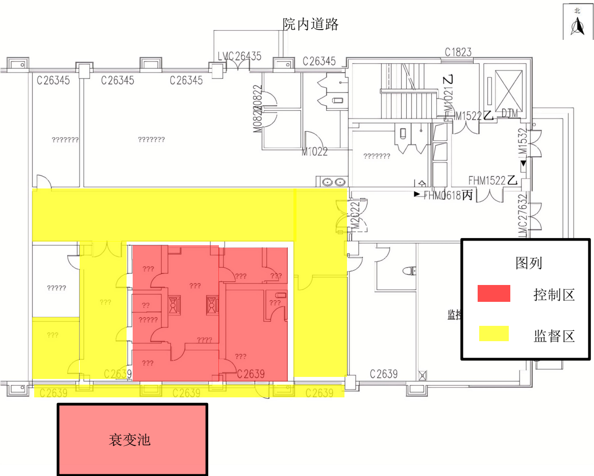
图 10-1 核医学科平面布置及分区图
