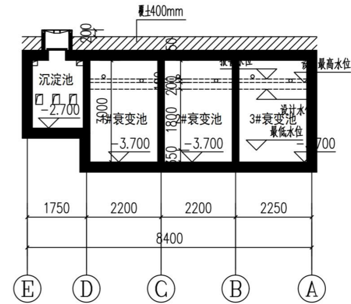
衰变池1-1剖面图 1:100
