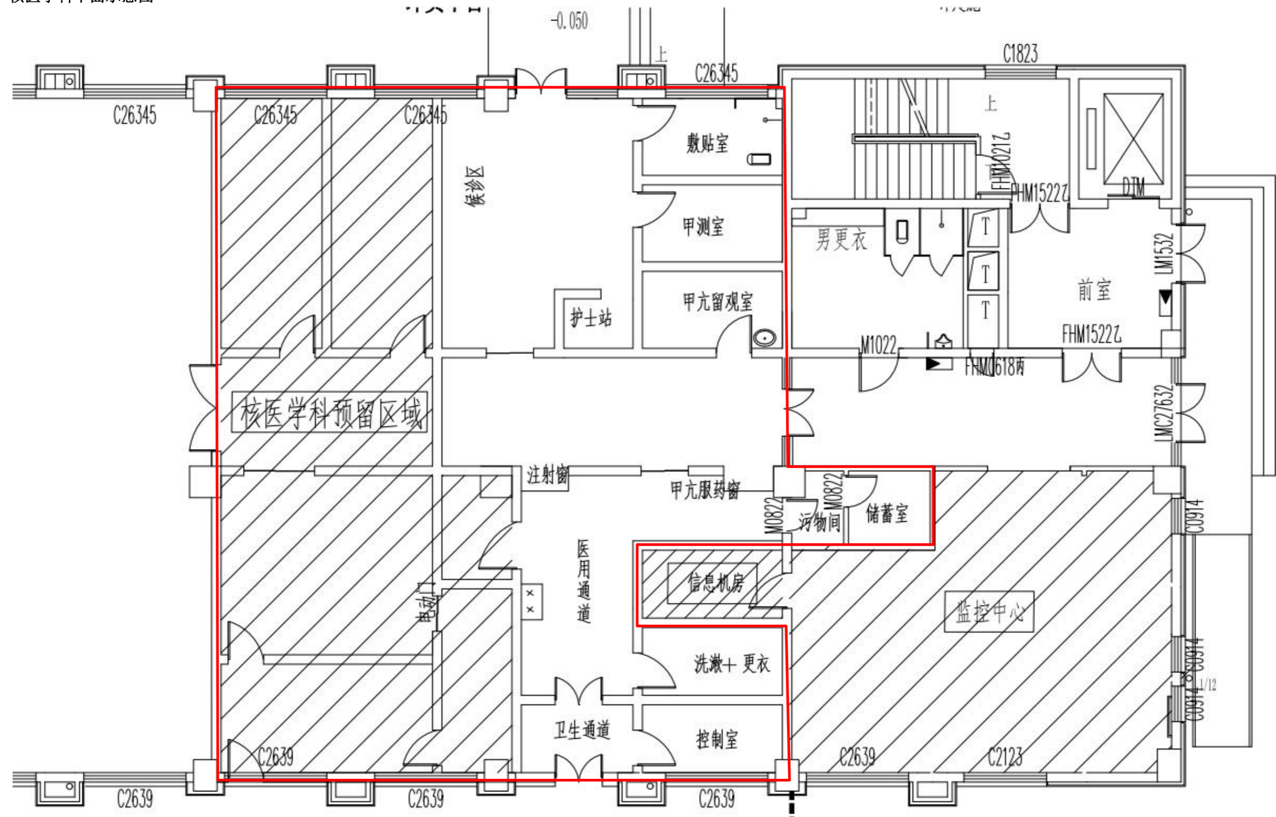
附图五：核医学科平面示意图
