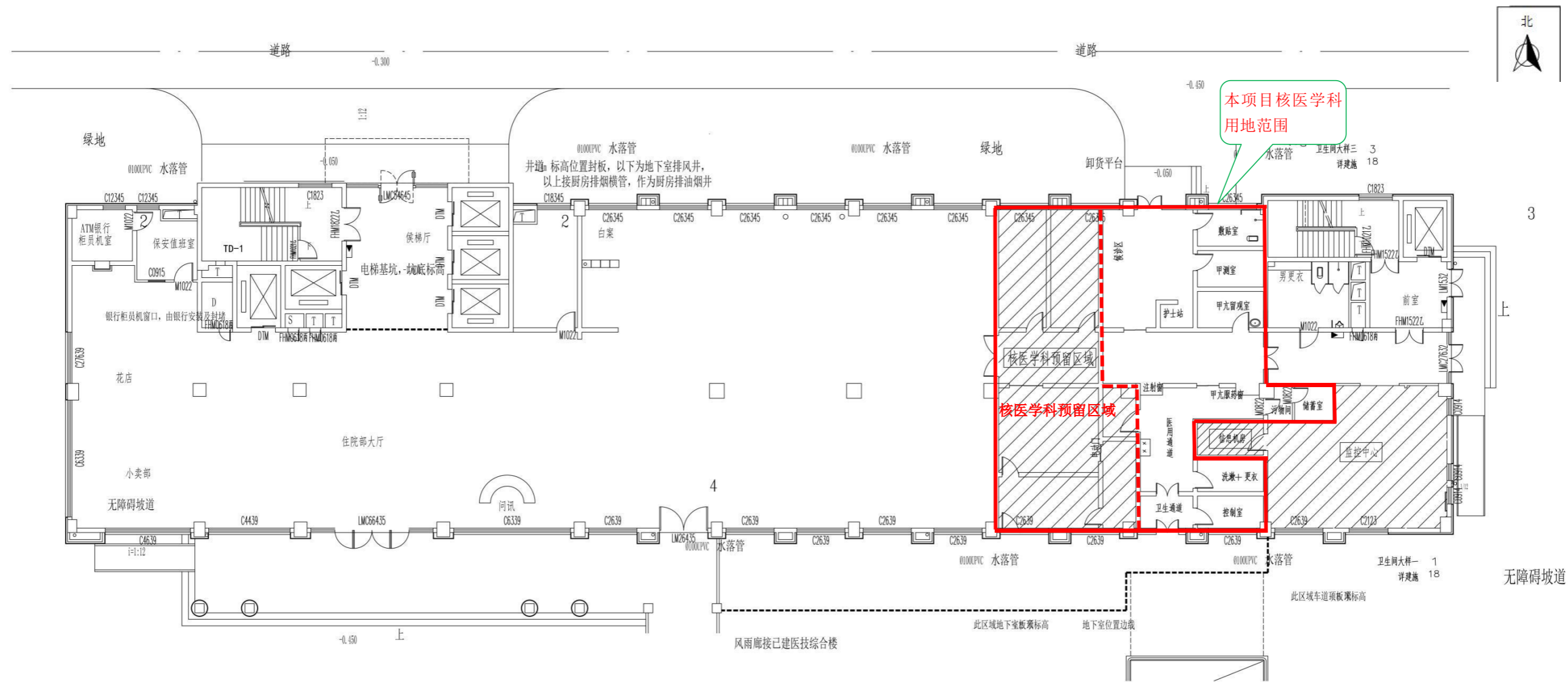
附图三：内科大楼一层平面示意图
