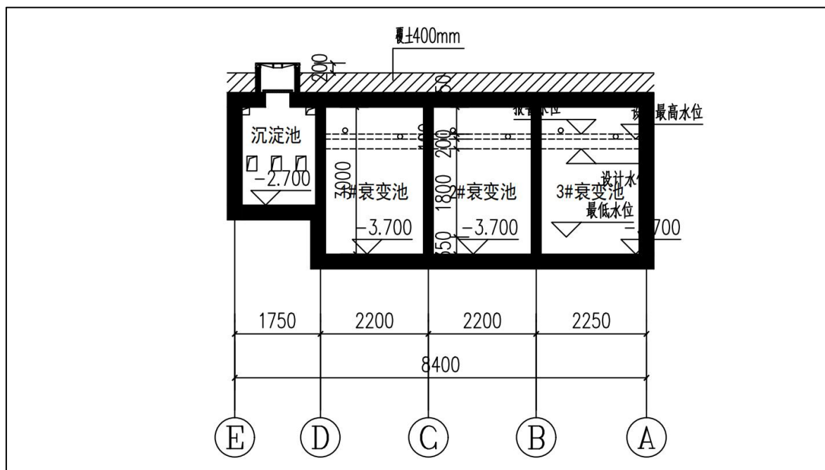
图 10-7 衰变池剖面图
