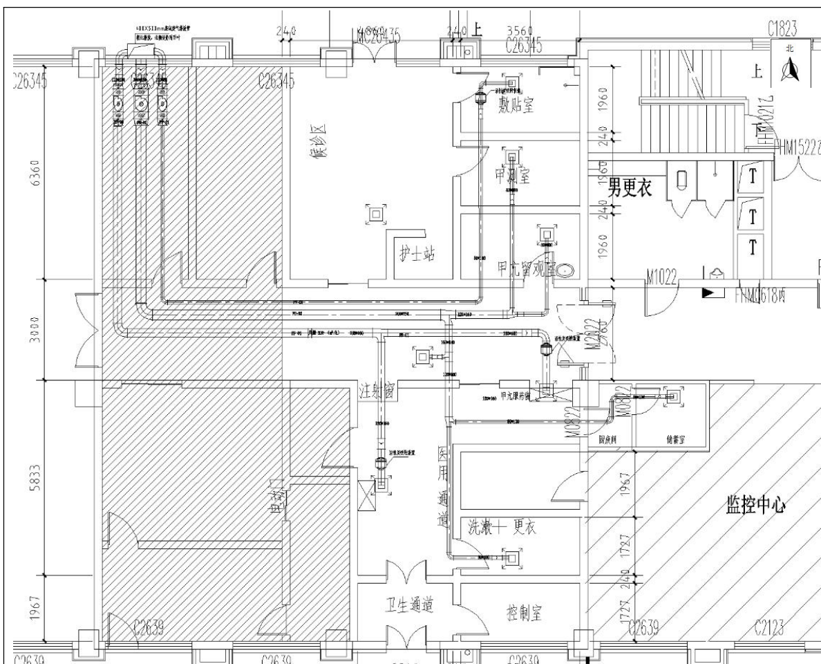
图 10-4 核医学科排风设计图
