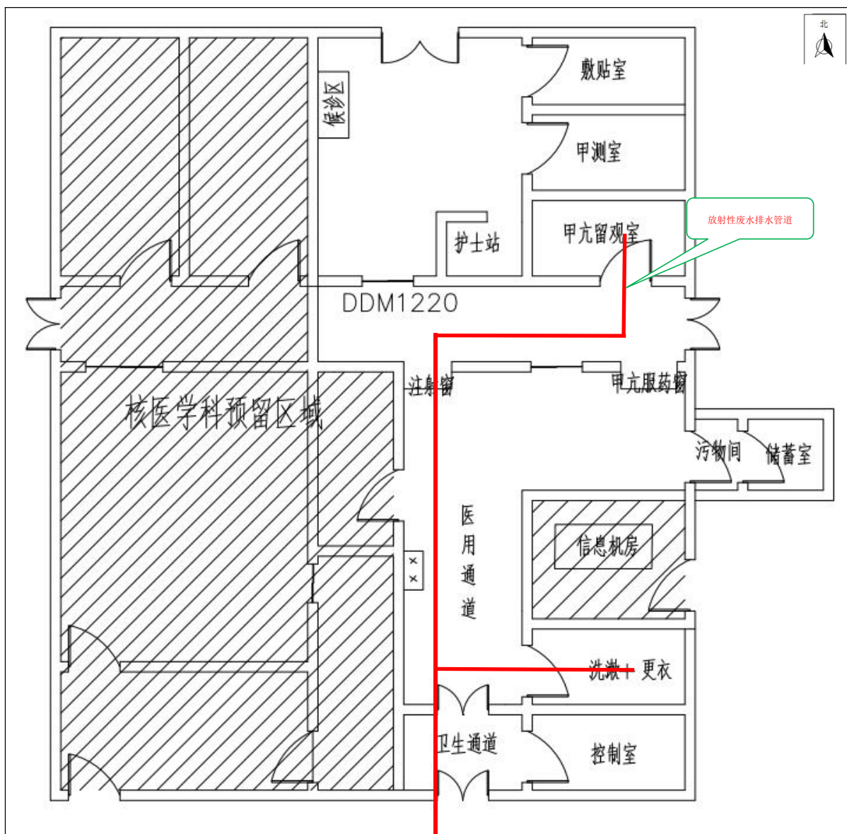
图 10-5 核医学科给排水设计图
