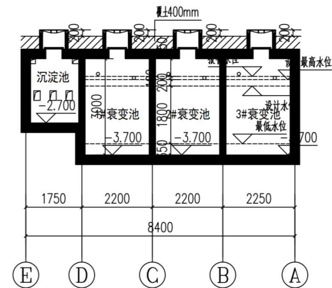
衰变池2-2剖面图 1:100
