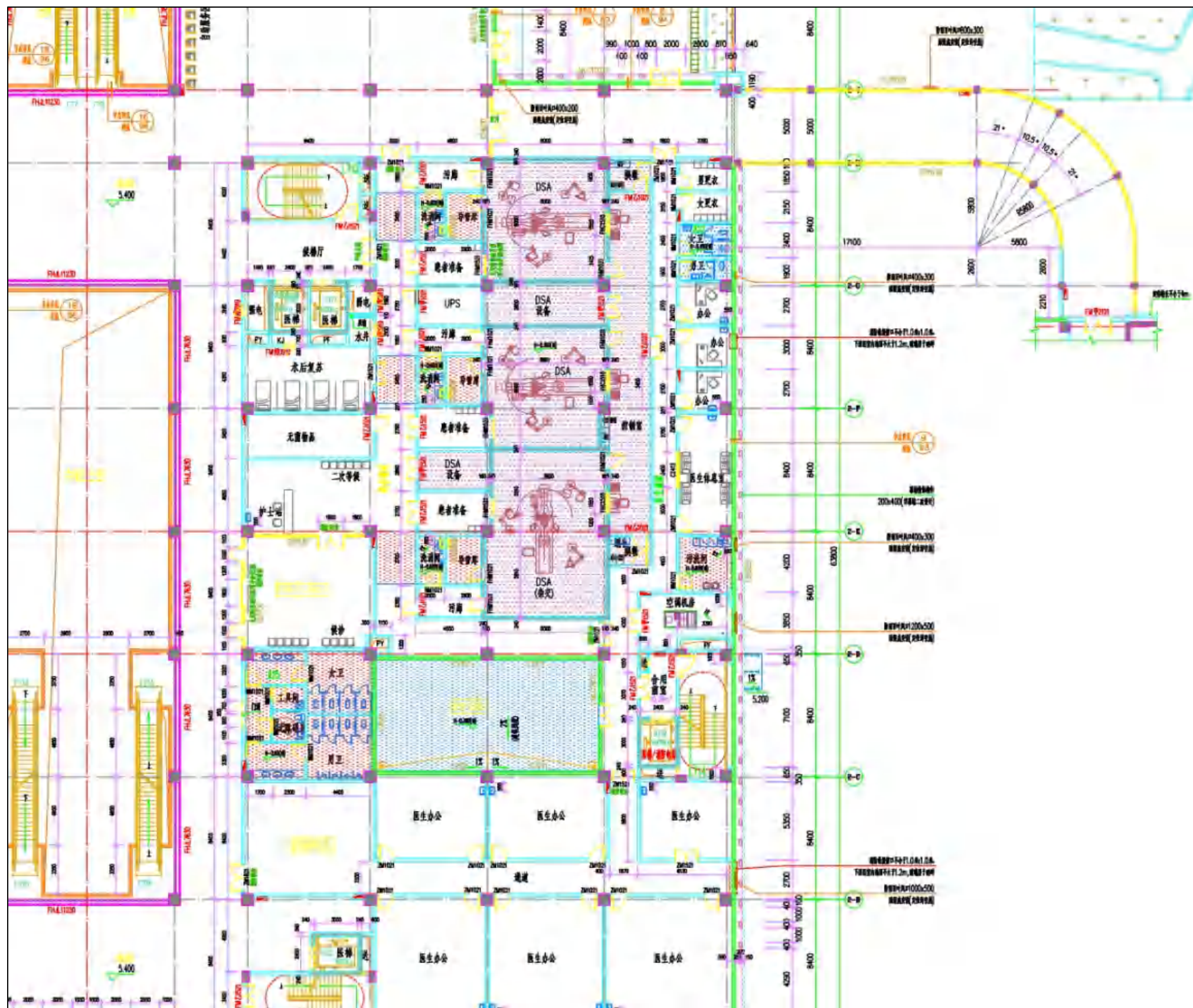
附图十二 门诊医技楼二楼 DSA 机房所在楼层平面布置图
