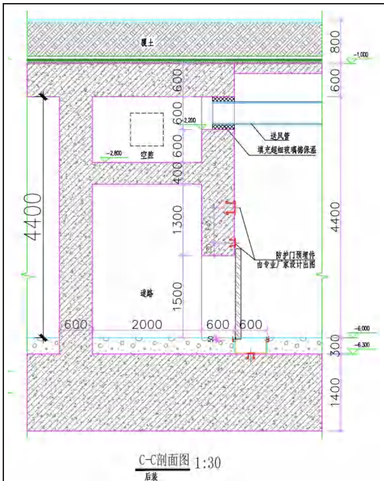
图 10-14 后装治疗机房防护示意图（剖面）
