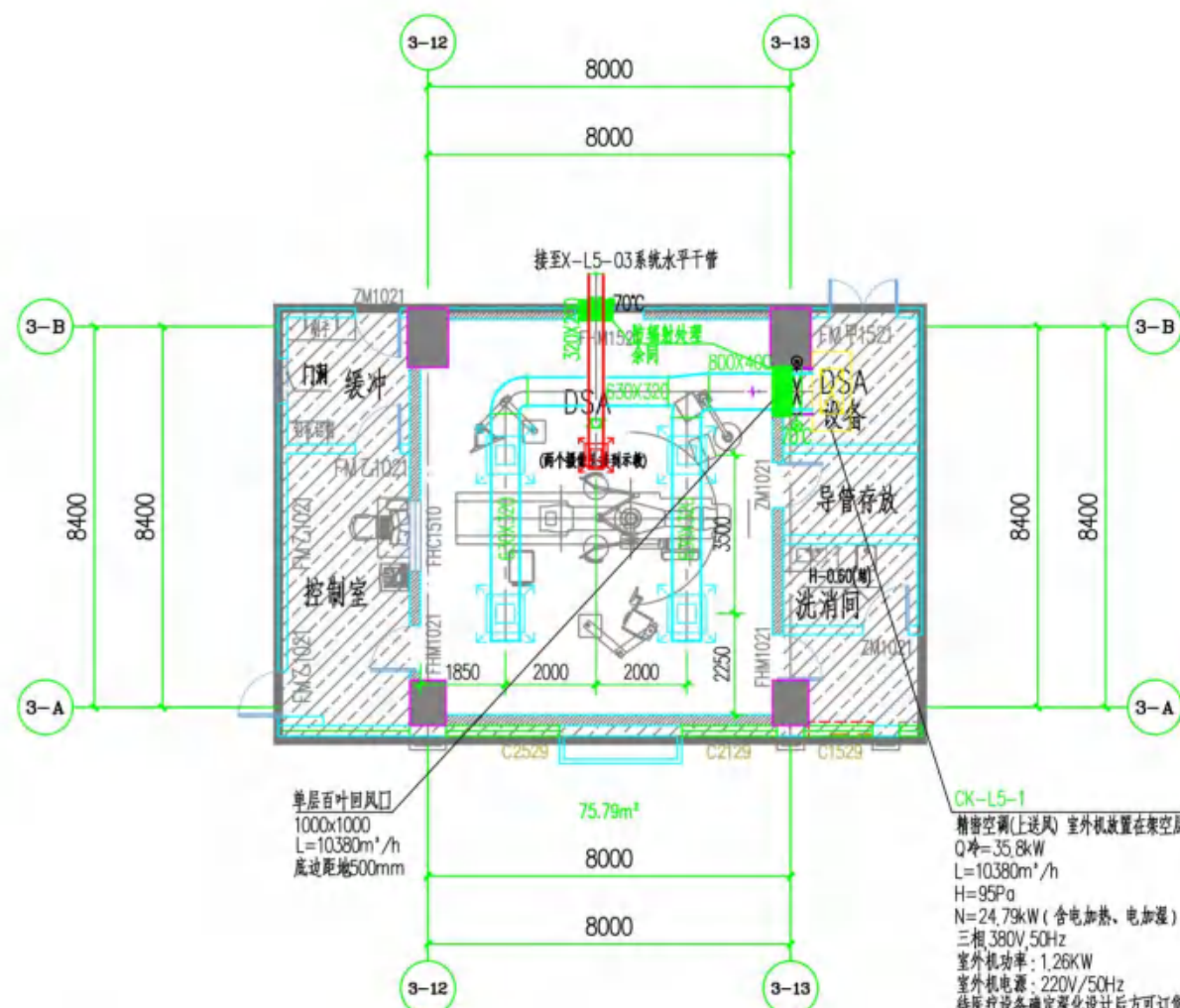
综合住院楼五层DSA防护范围空调通风平面图 1:150
