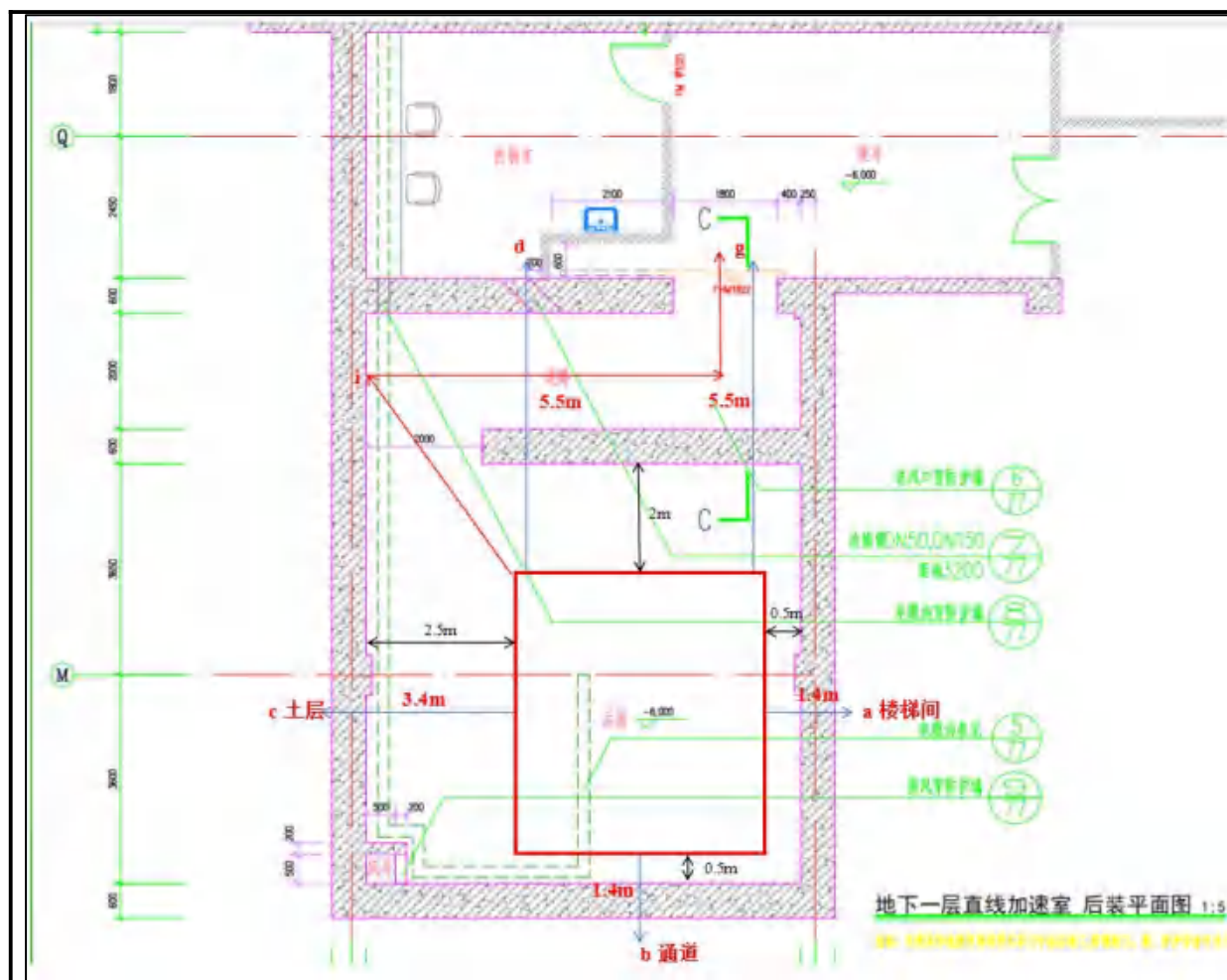
图 11-3 后装治疗机房关注点示意图（平面）
