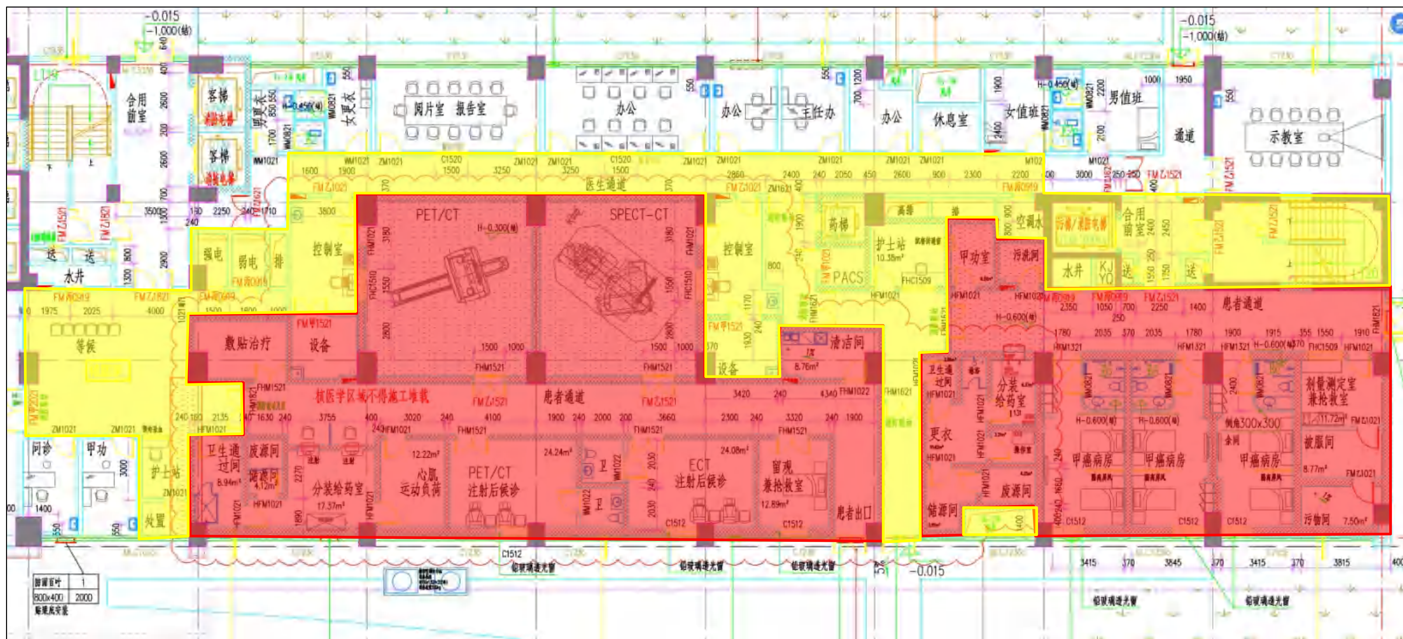
图 10-2 综合住院楼一楼核医学科场所分区图
