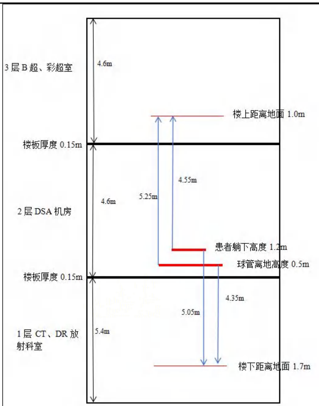
图 11-6 本项目 DSA 机房楼上楼下关注点位距离示意图（门诊医技楼）
