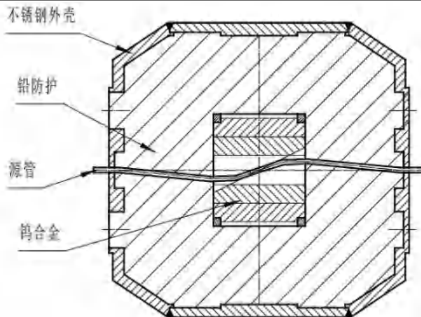
图 9-6 ^{192}\text{Ir} 放射源源罐结构示意图
