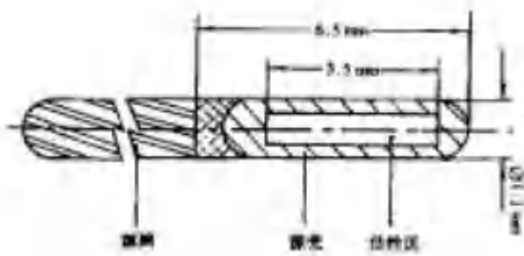
图 9-5 ^{192}\text{Ir} 源结构示意图
