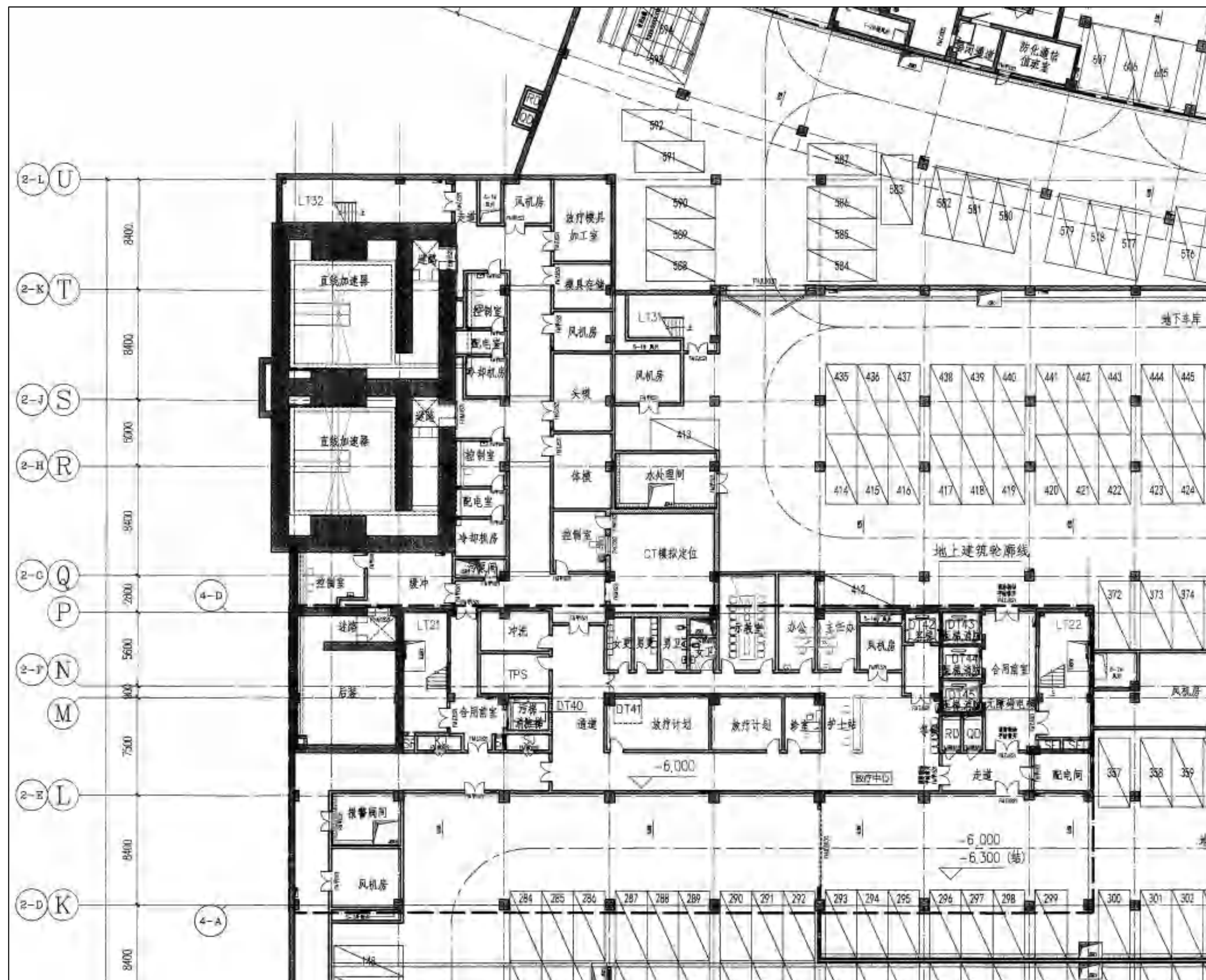
附图七 放射治疗场所所在门诊医技楼负一楼平面布置图
