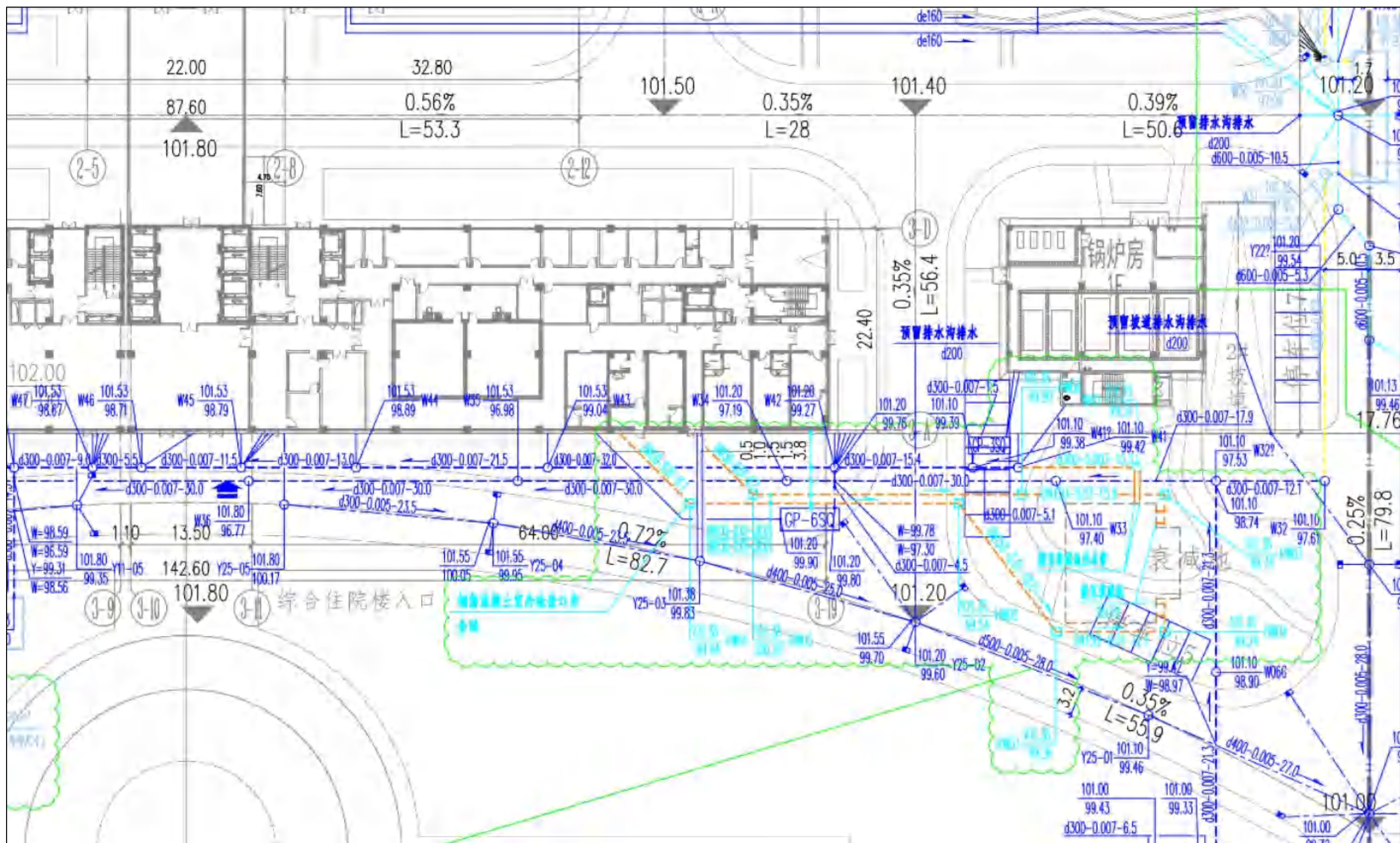
附图十七 核医学场所室外下水管道设计及衰变池位置示意图
