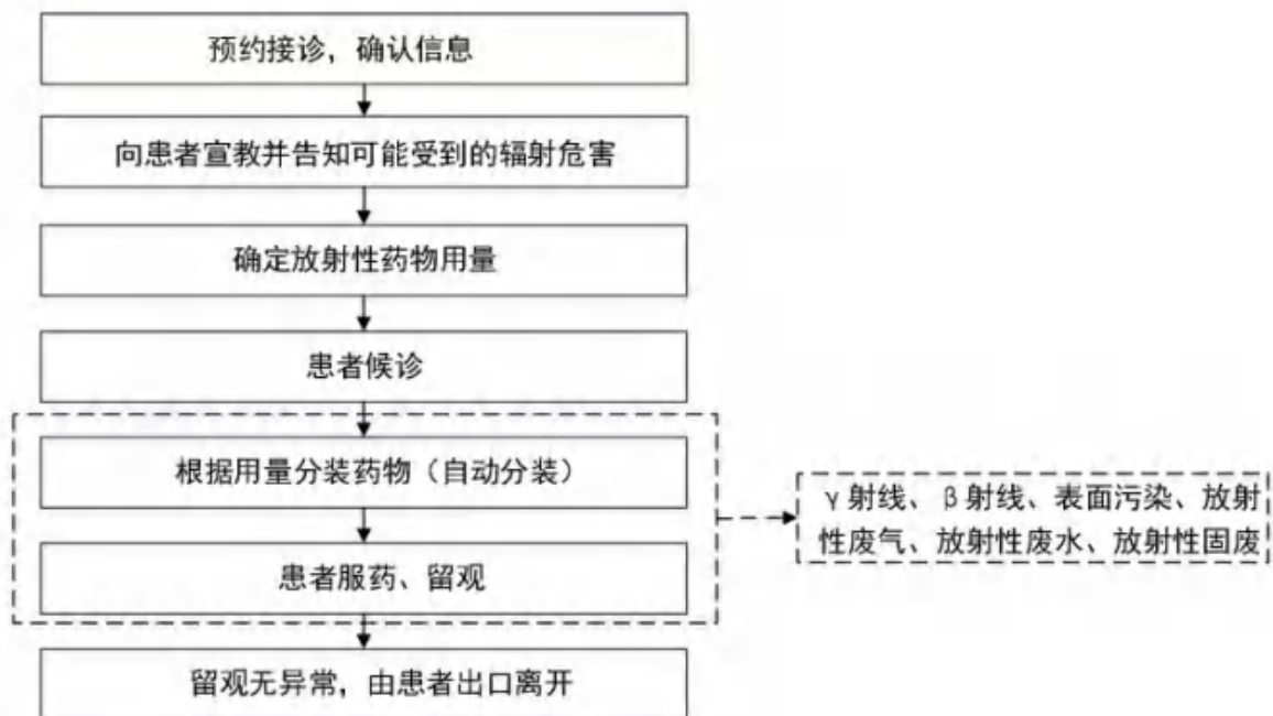
图 9-14 甲亢治疗工作流程及产污示意图
