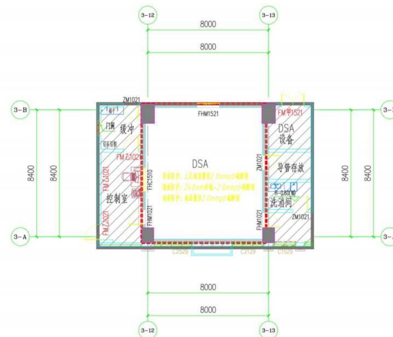
综合住院楼五层DSA设备基础图 1:150
