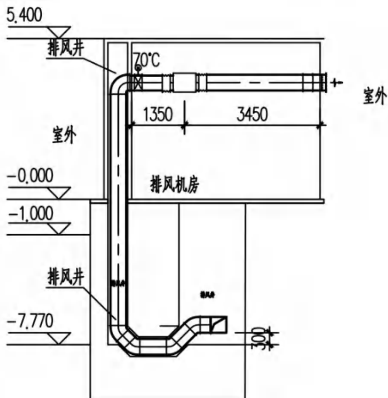
④ 排风穿防护墙剖面图 1:30 直线加速器室
