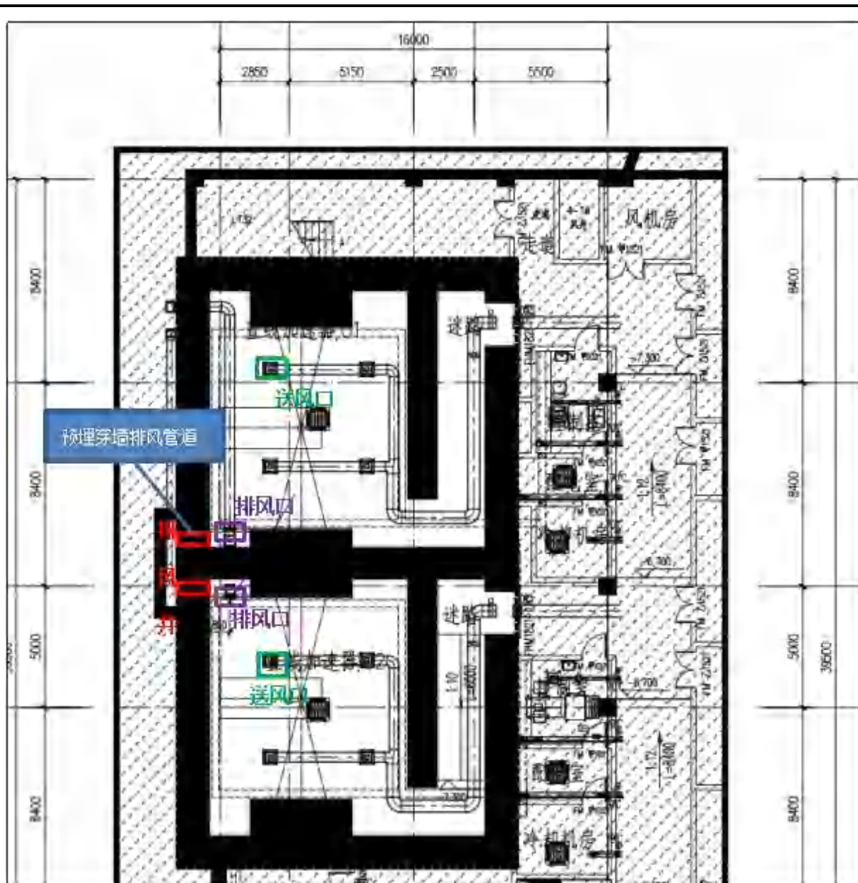
图 10-12 直线加速器机房通风示意图
