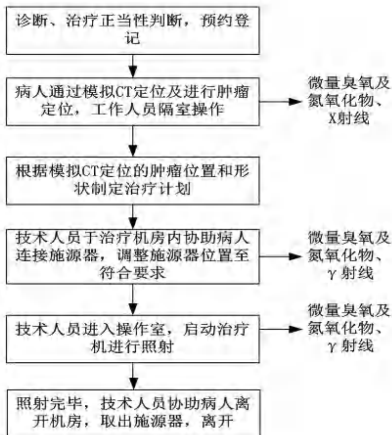
图 9-7 后装机治疗流程及产污环节示意图
