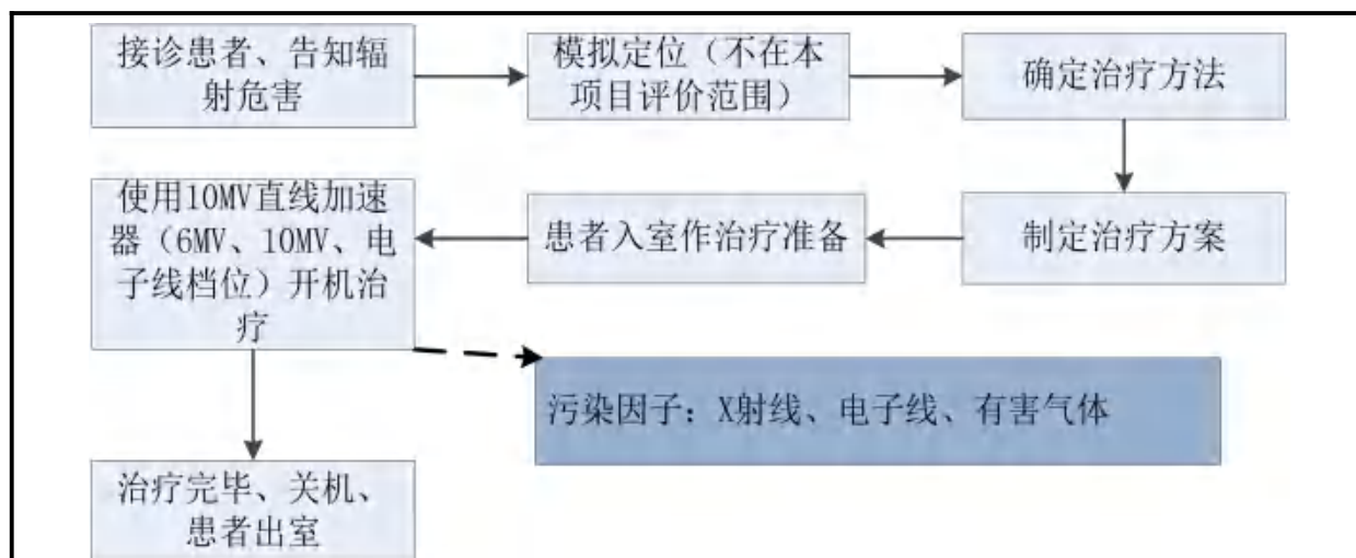
图 9-3 10MV 医用直线加速器操作流程及产污图
