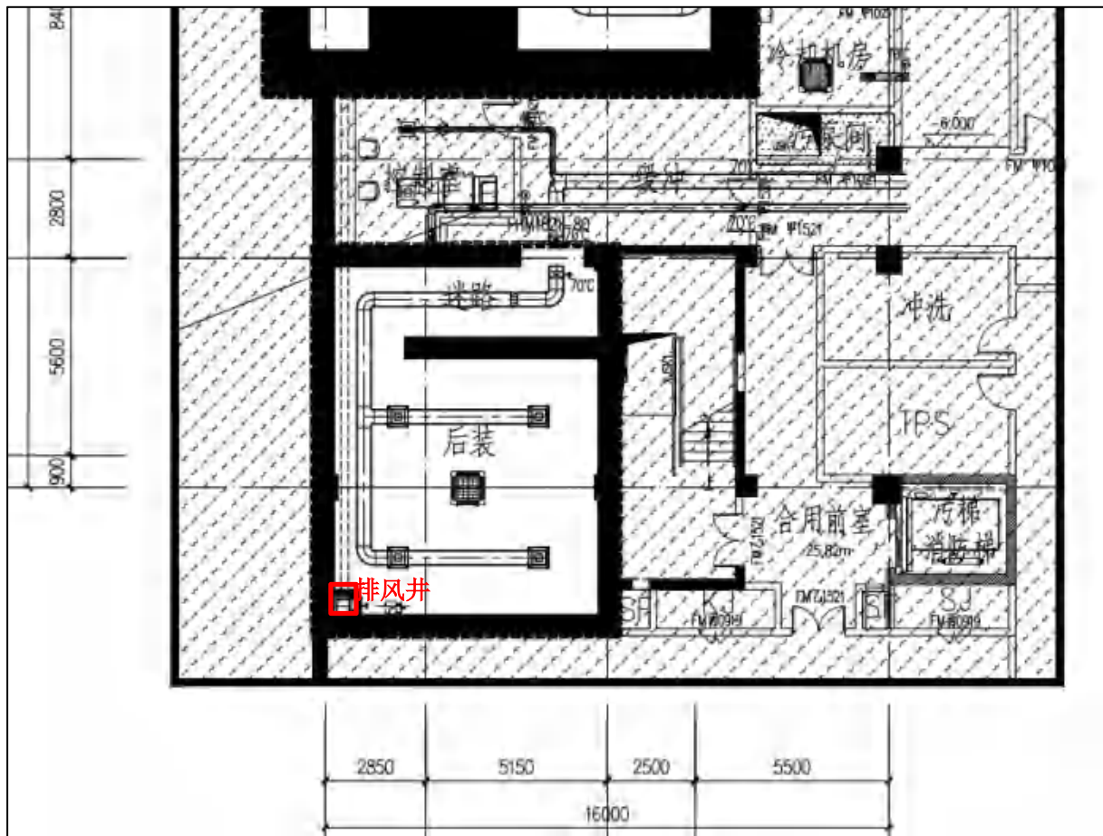
图 10-15 后装治疗机房通风示意图
