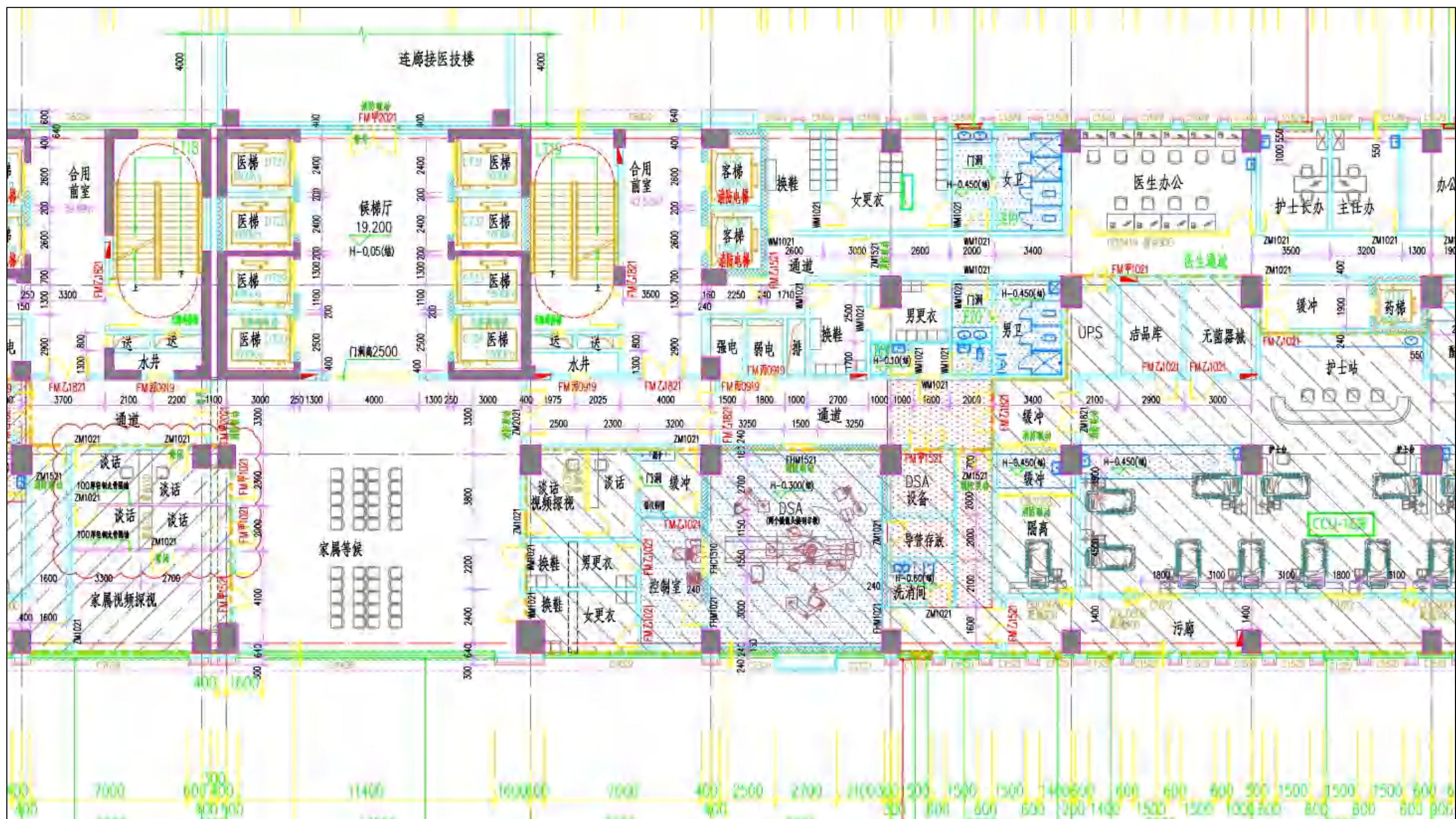
附图十三 综合住院楼五楼 DSA 机房所在楼层平面布置图
