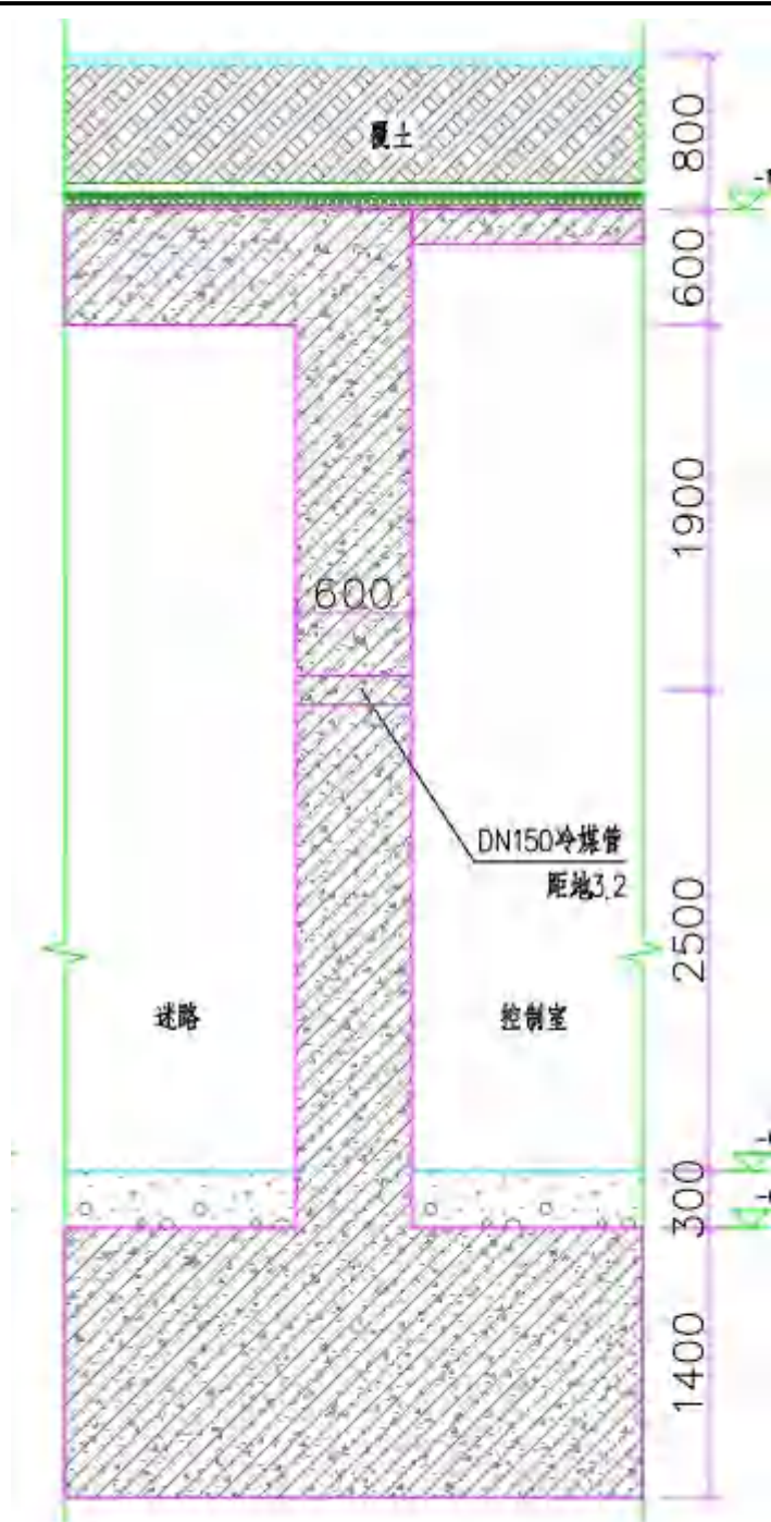
⑦ 冷媒管穿防护墙剖面图 1:30
