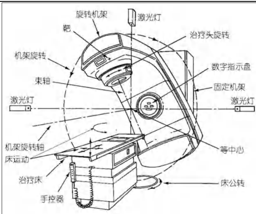
图 9-2 典型直线加速器外形示意图
