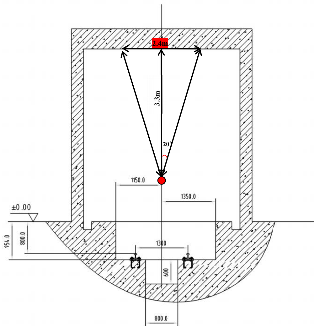
附图 4：出束角度示意图
