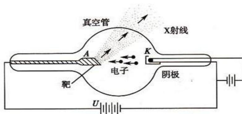
图 9-1X 射线管的原理示意图
