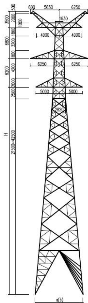
2F8-SZC2 直线塔
