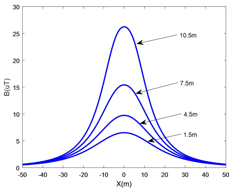
图 8-7 220kV 同塔双回线路（典型杆塔）工频磁场预测分布图
