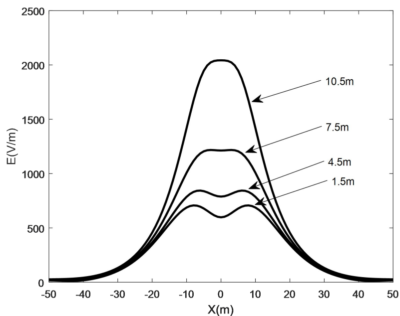
图 8-6 220kV 同塔双回线路（典型杆塔）工频电场预测分布图
