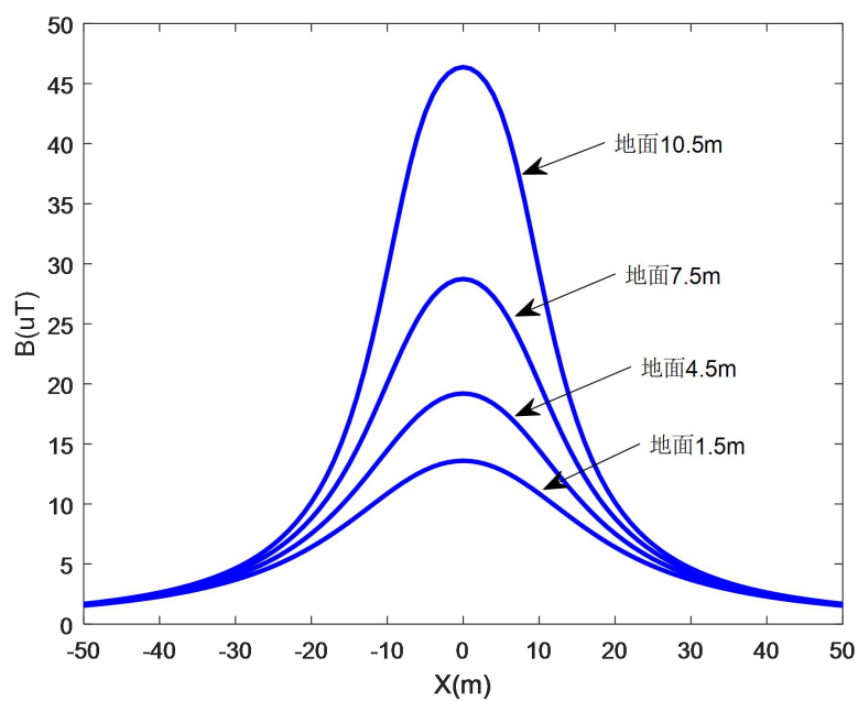
图 8-5 220kV 单回线路（典型杆塔）工频磁场预测分布图
