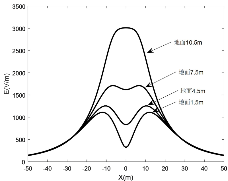
图 8-4 220kV 单回线路（典型杆塔）工频电场预测分布图
