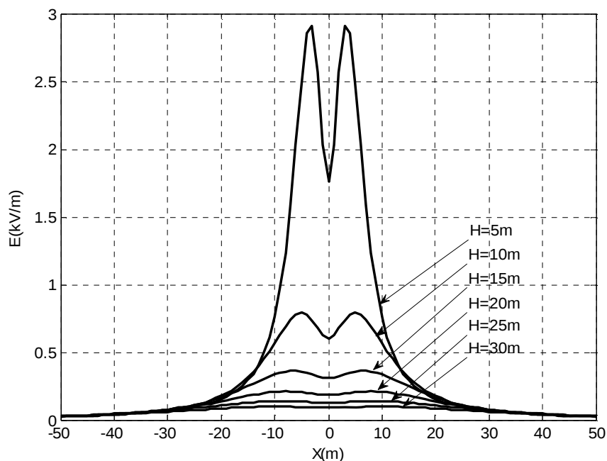
图 6 110kV 单回架设送出线路典型设计参数下工频电场强度预测结果
