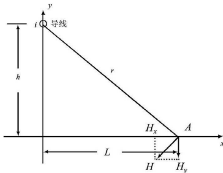
图 5 磁场向量图
