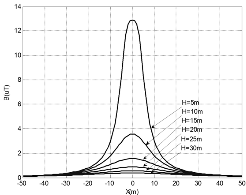
图 7 110kV 单回架设送出线路典型设计参数下磁感应强度预测结果
