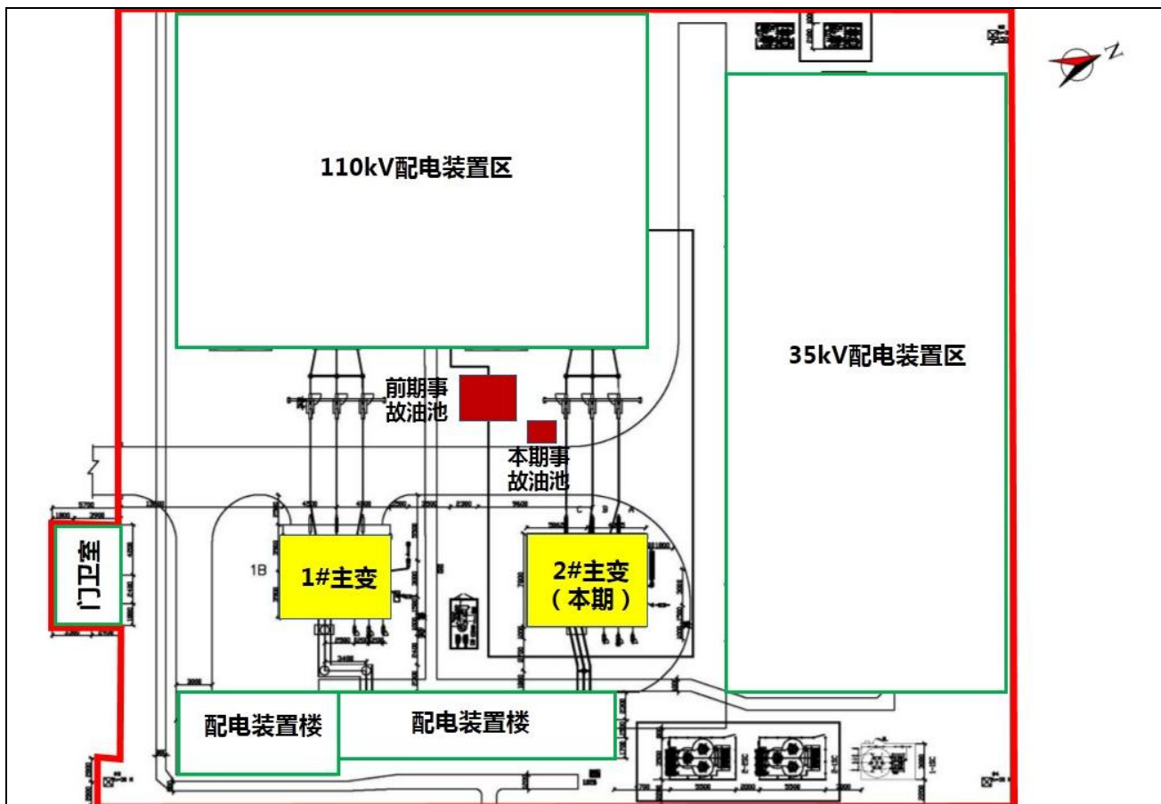
图 2 温塘 110kV 变电站总平面布置图
