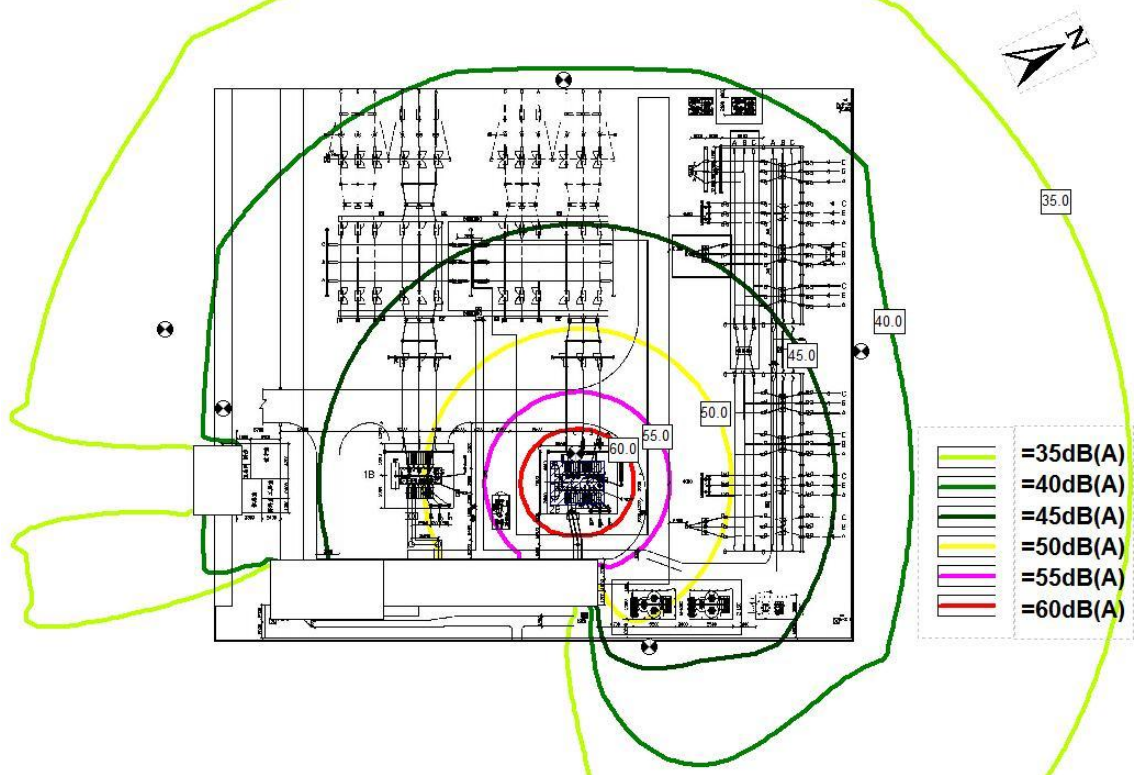
图 9 温塘 110kV 变电站本期规模噪声预测等值线图
