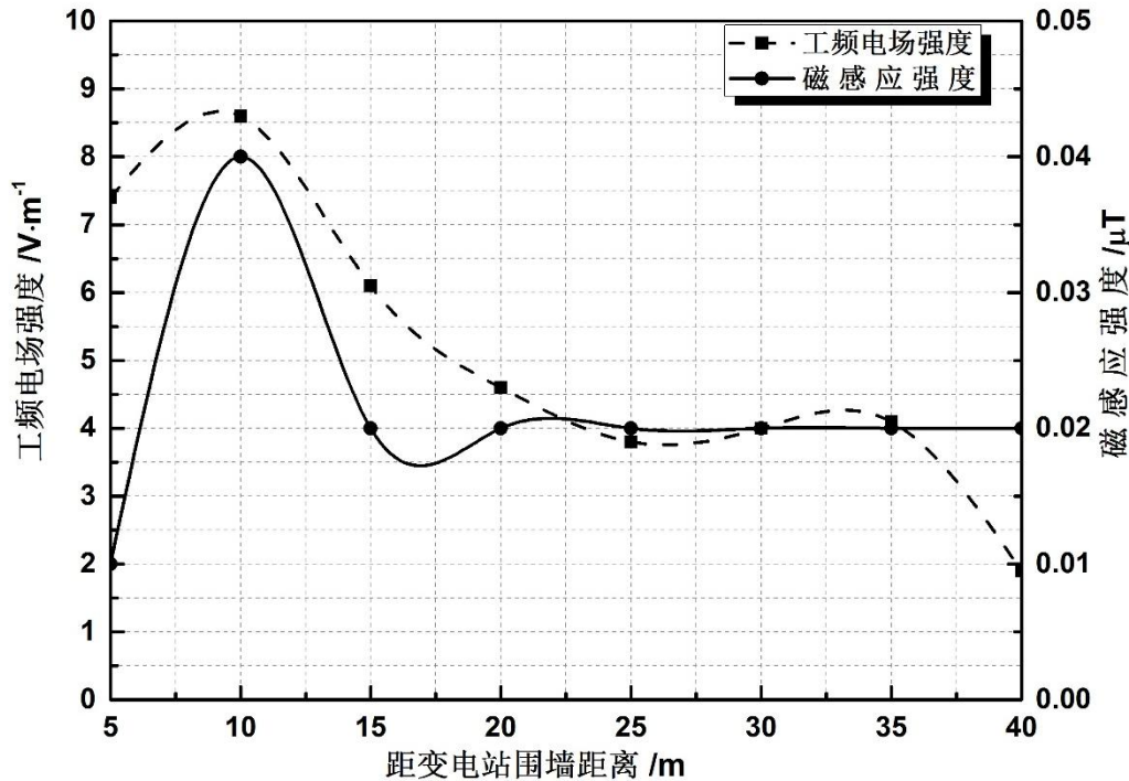
图 11 苏家村 110kV 变电站衰减断面监测结果分布图
