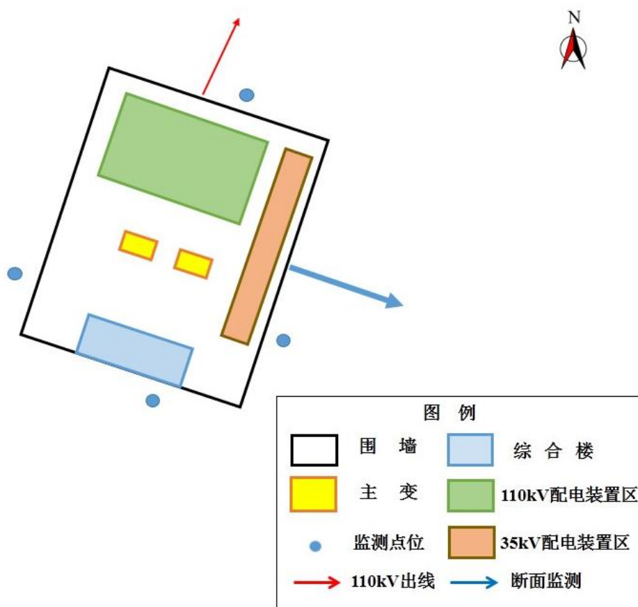
图 10 苏家村 110kV 变电站平面布置及类比监测示意图
