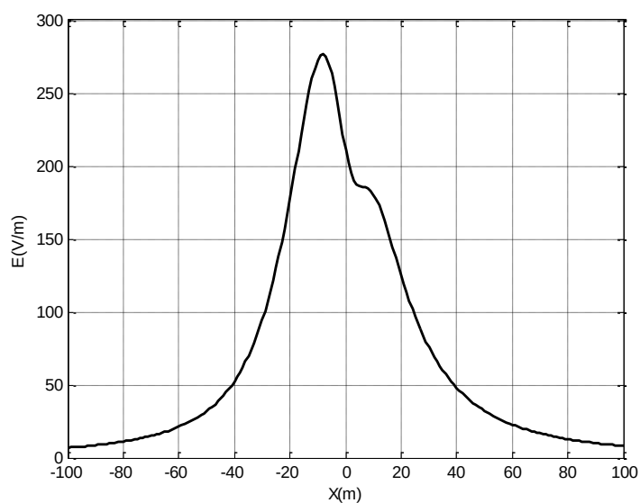
图 7-4 本项目工频电场强度预测结果
