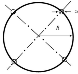
图 7-2 等效半径计算图
