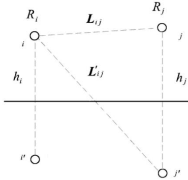
图 7-1 点位系数计算图
