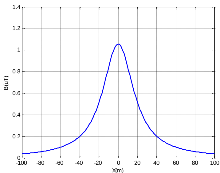
图 7-5 本项目磁感应强度预测结果
