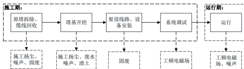
图 5-1 项目建设流程和产污节点图
