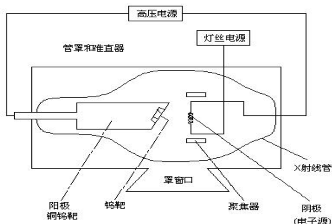
图 9-1 X 射线管的原理示意图
