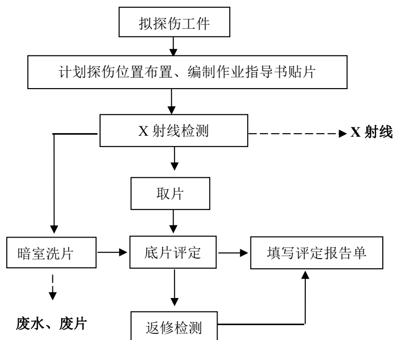
图 9-2 探伤工艺流程简图
